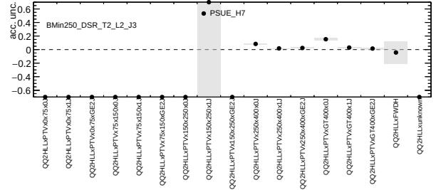
(f) qq \rightarrow ZH \rightarrow \ell^+ \ell^- b\bar{b}, 3\text{-jets}, p_T^V > 250 \text{ GeV}
