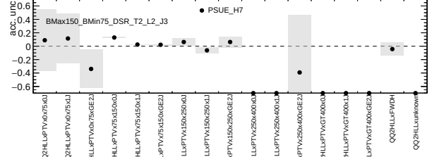
(b) qq \rightarrow ZH \rightarrow \ell^+ \ell^- b\bar{b}, 3\text{-jets}, 75 \leq p_T^V < 150 \text{ GeV}
