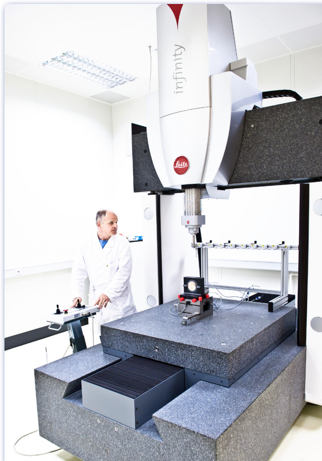
Infinity, la nouvelle machine de mesure ultra-précise, actuellement en opération au Service de métrologie du CERN.
