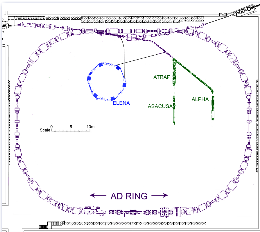
Plan de la salle de AD expérimentale : l'anneau décélérateur d'antiprotons (le grand anneau), l'ALPHA, ASACUSA et les expériences ATRAP ; l'expérience ACE (non représentée), et le nouvel anneau d'ELENA (le petit anneau).
