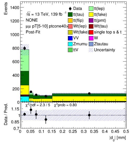
(d) \mu - \mu channel, pt_{cone40} > 2 \text{ GeV}
