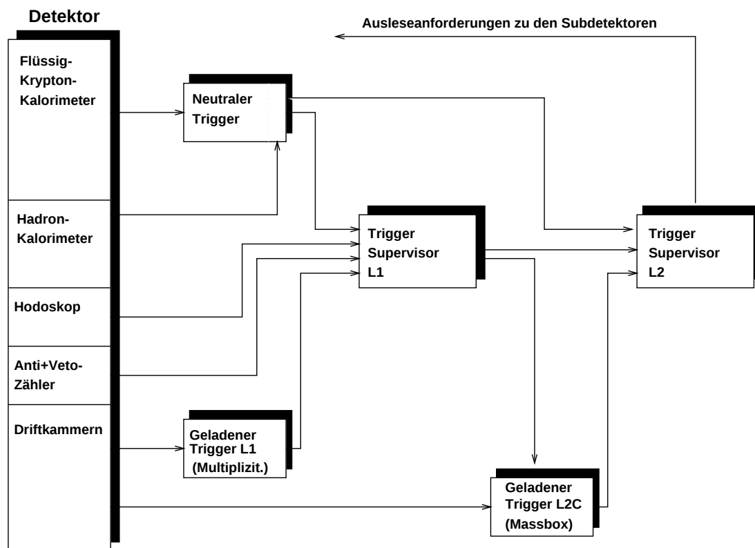
Abbildung 3.1: Übersicht über das NA48-Triggersystem.
