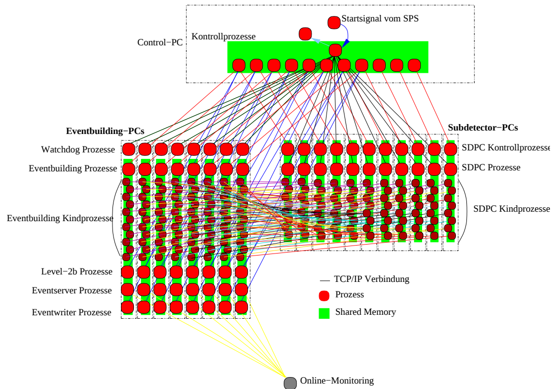
Abbildung A.3: Datenfluss in der PC-Farm.
