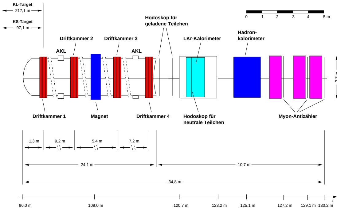
Abbildung 2.2: Aufbau des NA48-Detektors.
