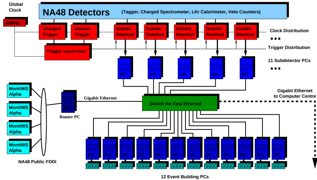
Abbildung A.1: Aufbau der Eventbuilding-Farm.
