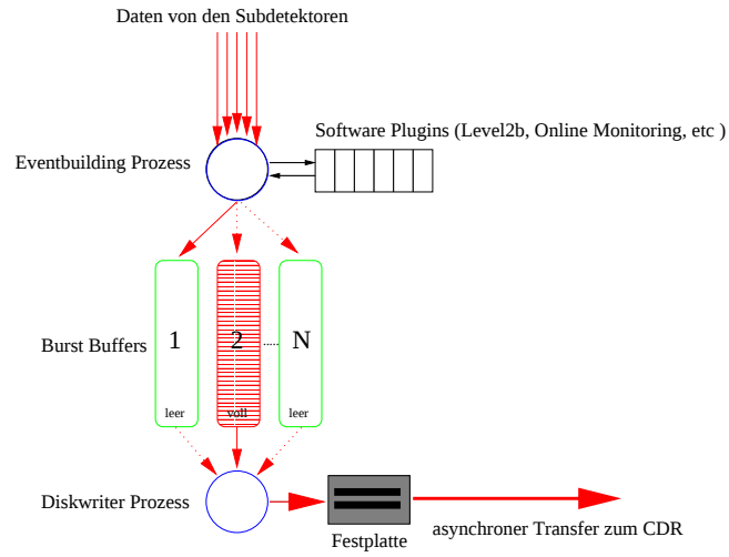
Abbildung A.2: Prozesse auf den Eventbuilding-PCs.
