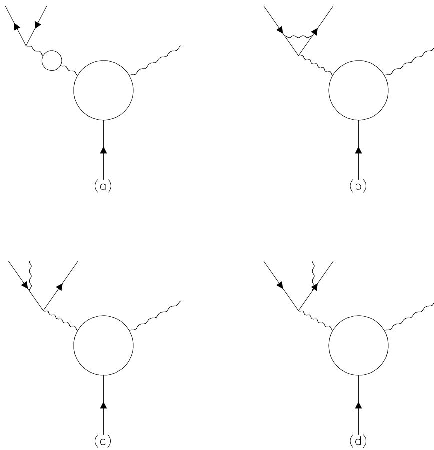
Abbildung 1.8: Feynman-Diagramme für Strahlungskorrekturen erster Ordnung.
