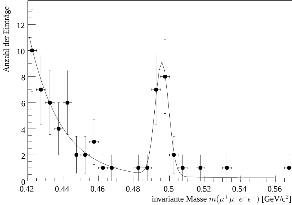
Abbildung 6.11: Die rekonstruierte Masse für \mu^+ \mu^- e^+ e^- -Kandidaten.
