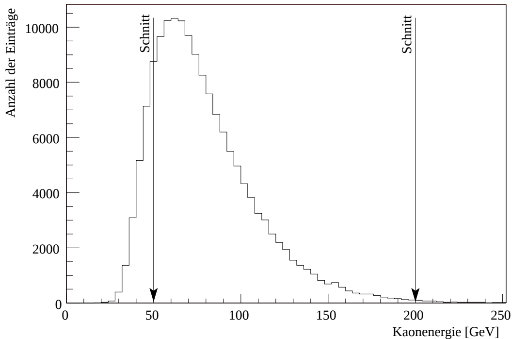
Abbildung 6.4: Die rekonstruierte Kaonenergie für K_L \rightarrow \pi^+\pi^-\pi_D^0 Kandidaten.
