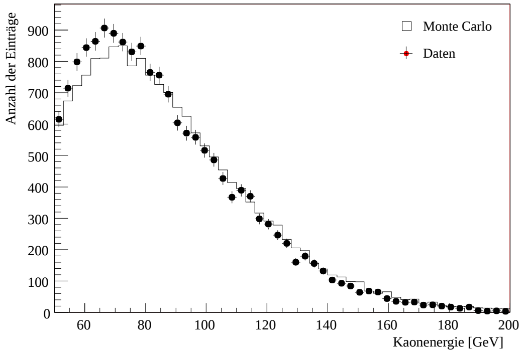
Abbildung 6.18: Vergleich der rekonstruierten Kaonenergie K_L \rightarrow \pi^+\pi^-\pi_D^0 .
