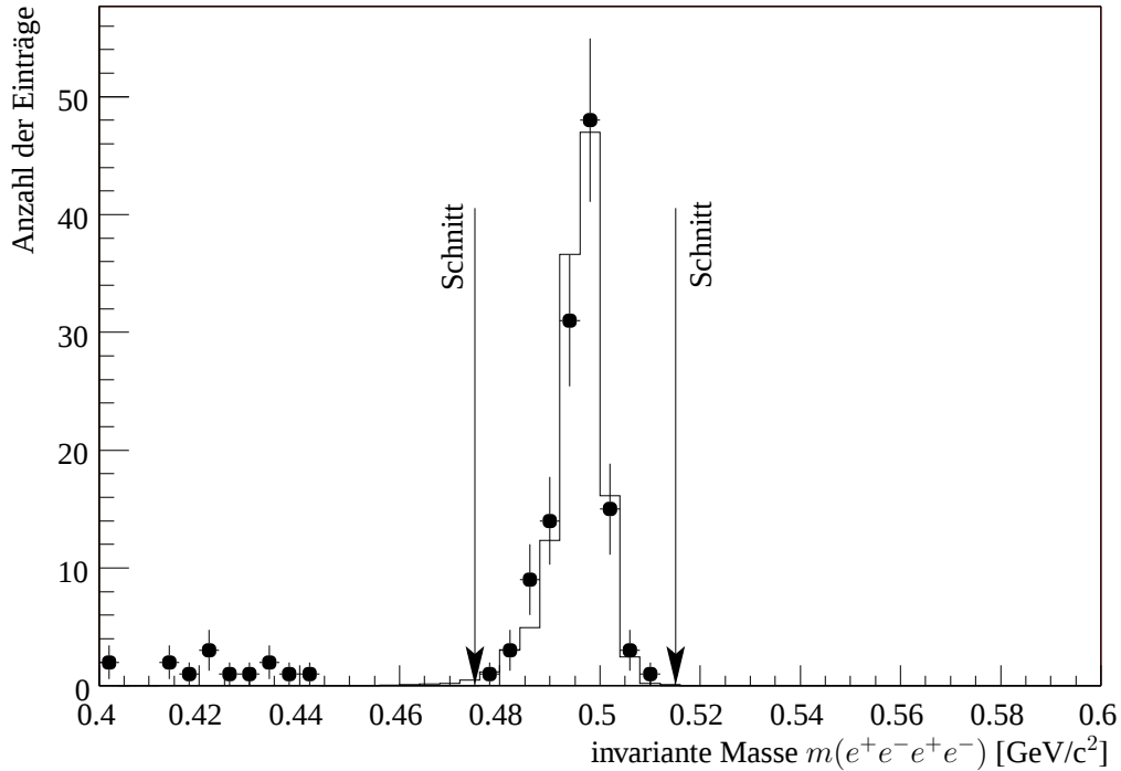
Abbildung 6.8: Die rekonstruierte Kaonmasse für K_L \rightarrow e^+e^-e^+e^- -Kandidaten.
