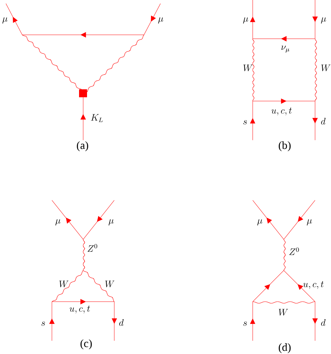
Abbildung 1.7: Langreichweitiger Beitrag (a) und kurzreichweitige Beiträge (b, c, d) zum Zerfall K_L \rightarrow \mu^+ \mu^- in niedrigster Ordnung.
