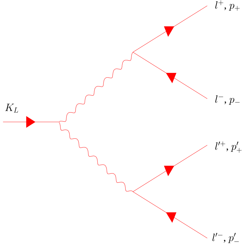
Abbildung 1.4: Feynman-Diagramm für den Zerfall K_L \rightarrow l^+ l^- l^+ l^- .
