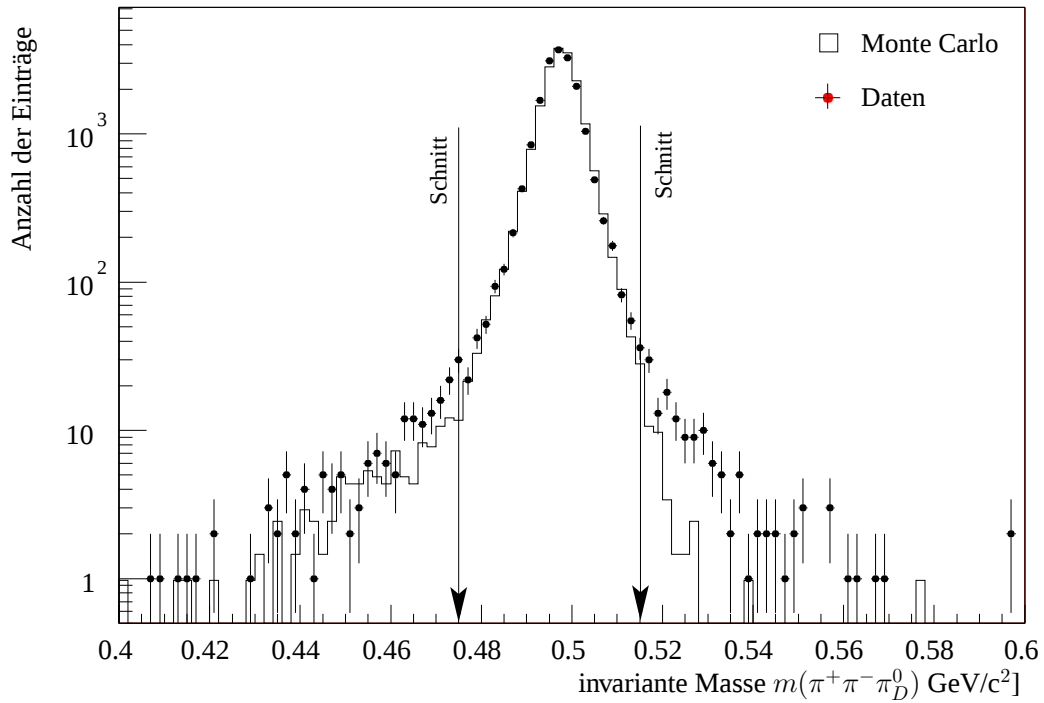
Abbildung 6.13: Die rekonstruierte Kaonmasse für K_L \rightarrow \pi^+\pi^-\pi_D^0 -Kandidaten im Vergleich von Daten und Monte-Carlo.
