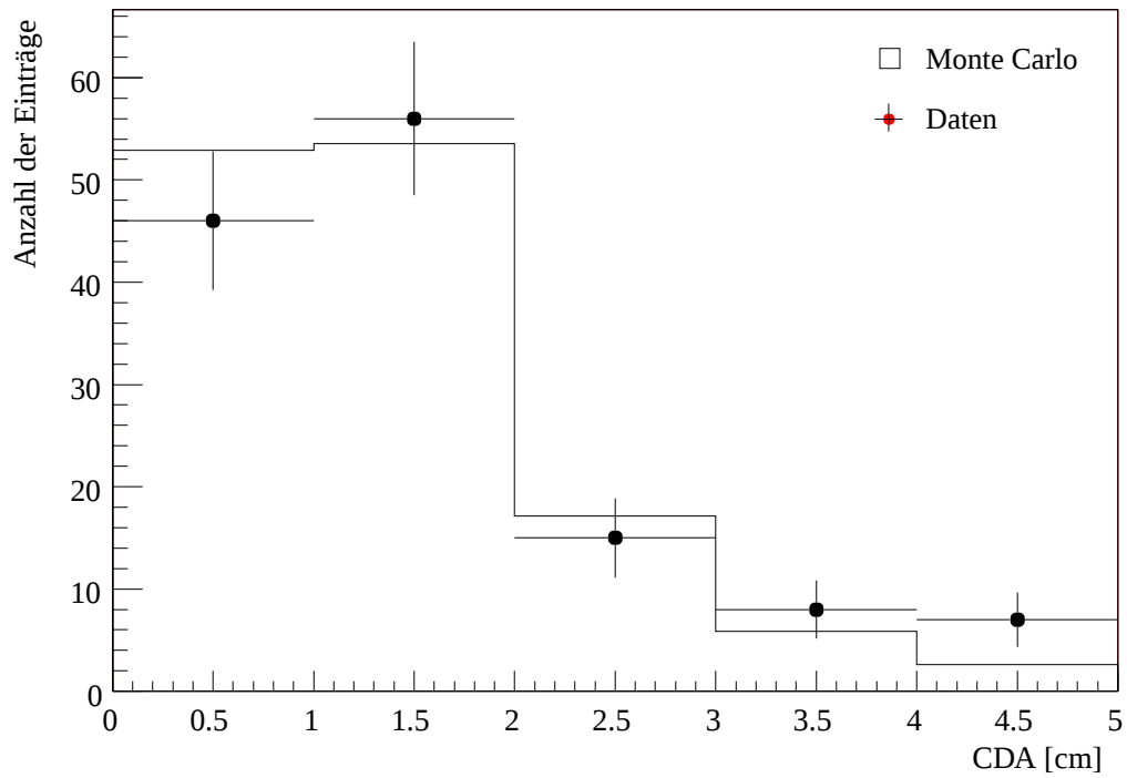
Abbildung 6.21: Vergleich der CDA-Verteilung für K_L \rightarrow e^+e^-e^+e^- .
