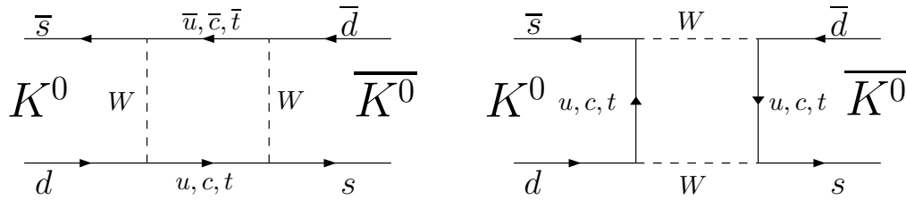
Abbildung 1.2: Box-Diagramme zur Zustandsmischung von K^0 - und \overline{K}^0 -Mesonen.
