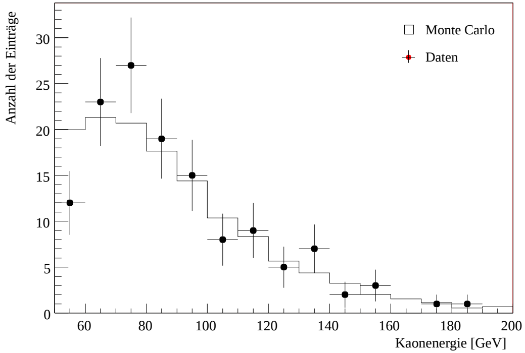
Abbildung 6.17: Vergleich der rekonstruierten Kaonenergie K_L \rightarrow e^+e^-e^+e^- .
