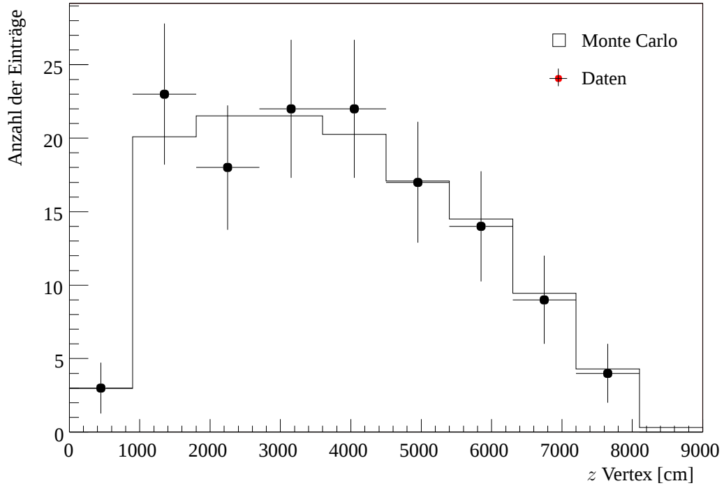
Abbildung 6.15: Vergleich der z -Vertexverteilung für K_L \rightarrow e^+e^-e^+e^- .
