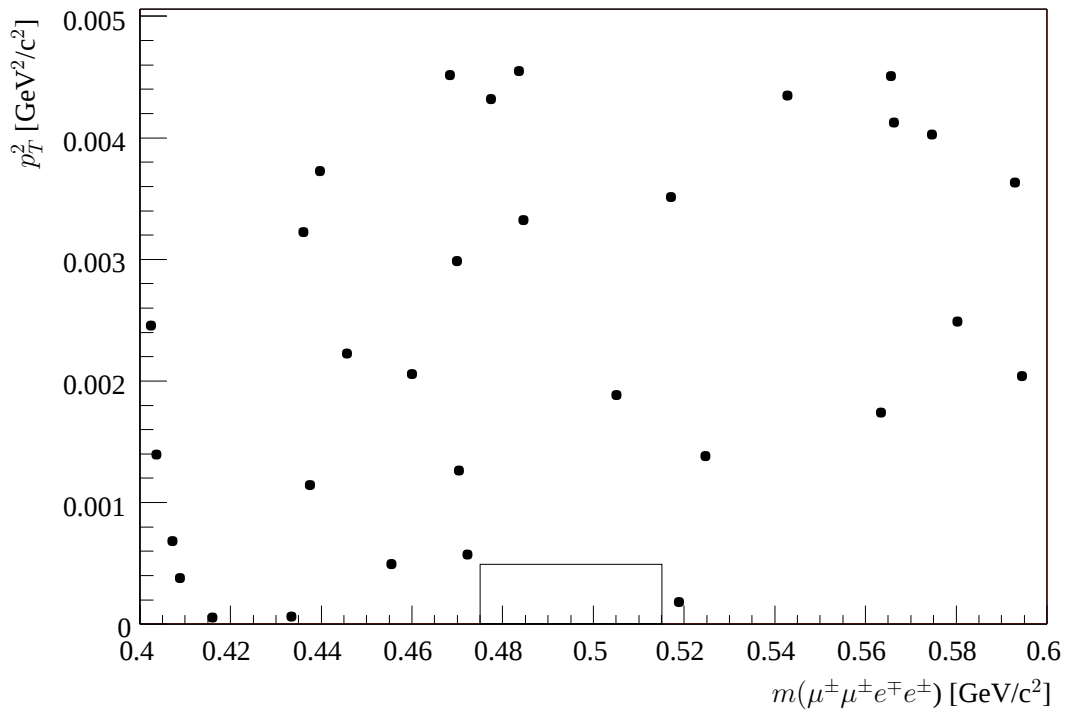
Abbildung 6.14: Das Quadrat des Transversalimpulses gegen die rekonstruierte \mu^\pm \mu^\pm e^\mp e^\mp Masse. Es verbleiben in der definierten Signalregion keine Ereignisse.
