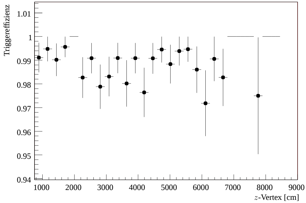
Abbildung 7.2: Effizienz des Vierspur-Triggers für K_L \rightarrow e^+e^-e^+e^- -Monte-Carlo-Ereignisse.
