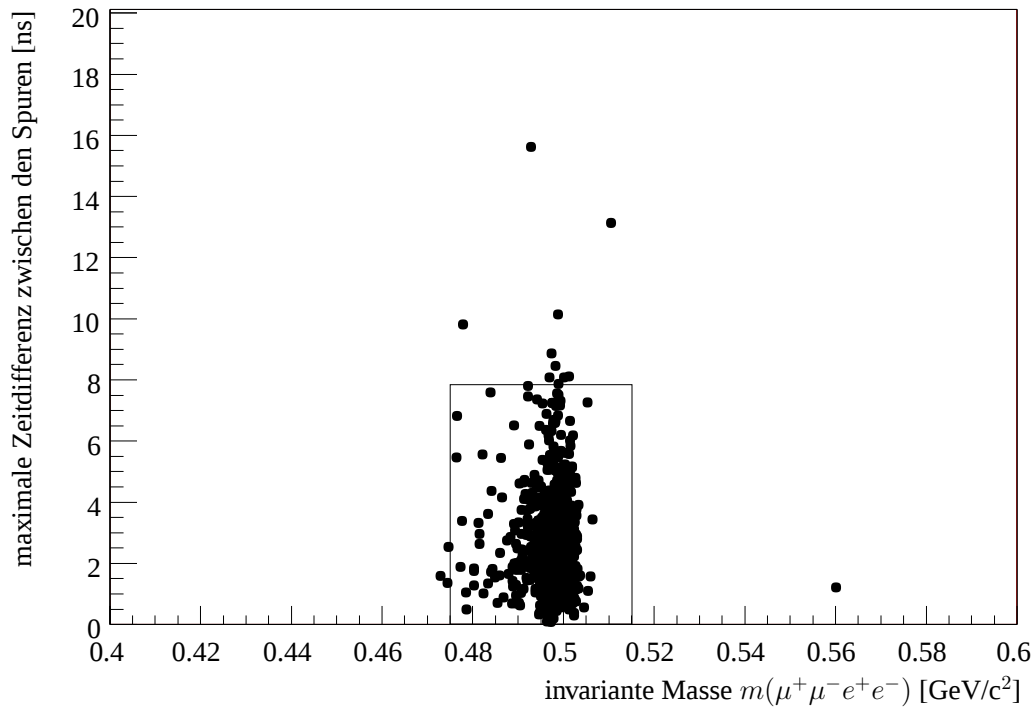
Abbildung 6.9: Maximale Zeitdifferenzen zwischen den Spuren gegen die invariante Masse des \mu^+\mu^-e^+e^- -Systems. Oben für Daten-, unten für Monte-Carlo-Ereignisse.
