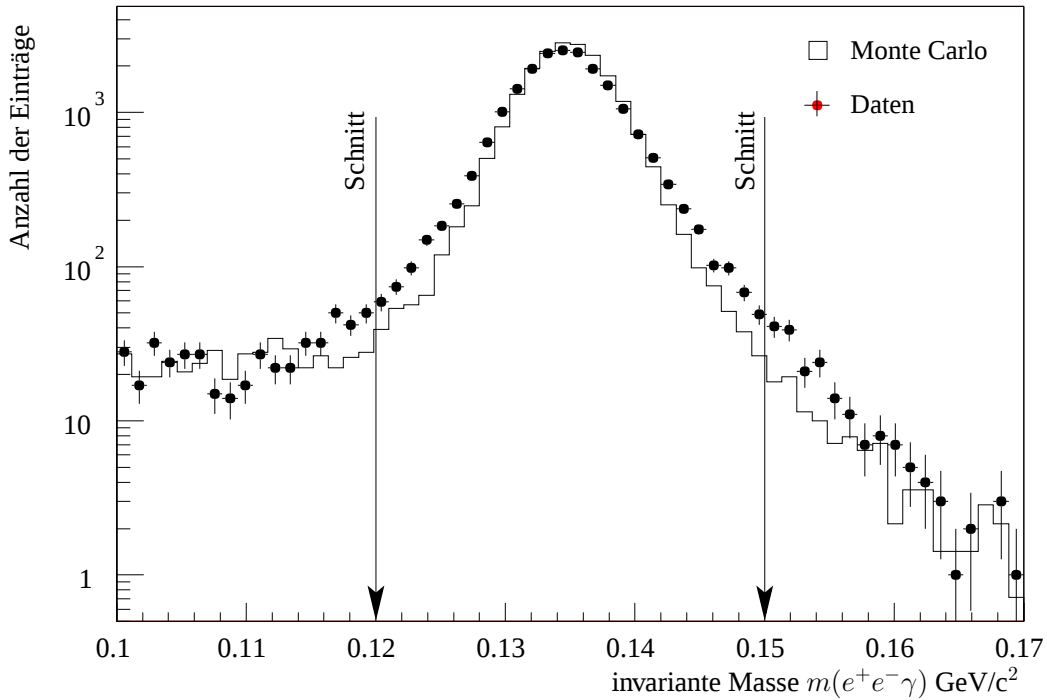
Abbildung 6.12: Vergleich der rekonstruierten \pi^0 -Masse aus K_L \rightarrow \pi^+\pi^-\pi_D^0 Zerfällen zwischen Daten und Monte-Carlo.
