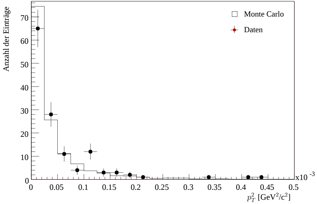
Abbildung 6.19: Vergleich der p_T^2 -Verteilung für K_L \rightarrow e^+e^-e^+e^- .
