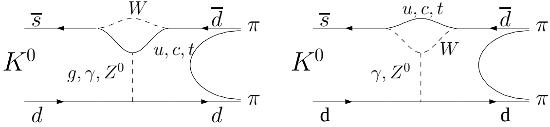
Abbildung 1.3: Penguin-Diagramme zur CP -Verletzung im System der neutralen Kaonen.
