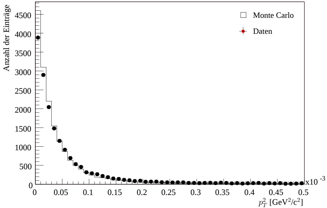
Abbildung 6.20: Vergleich der p_T^2 -Verteilung für K_L \rightarrow \pi^+\pi^-\pi_D^0 .
