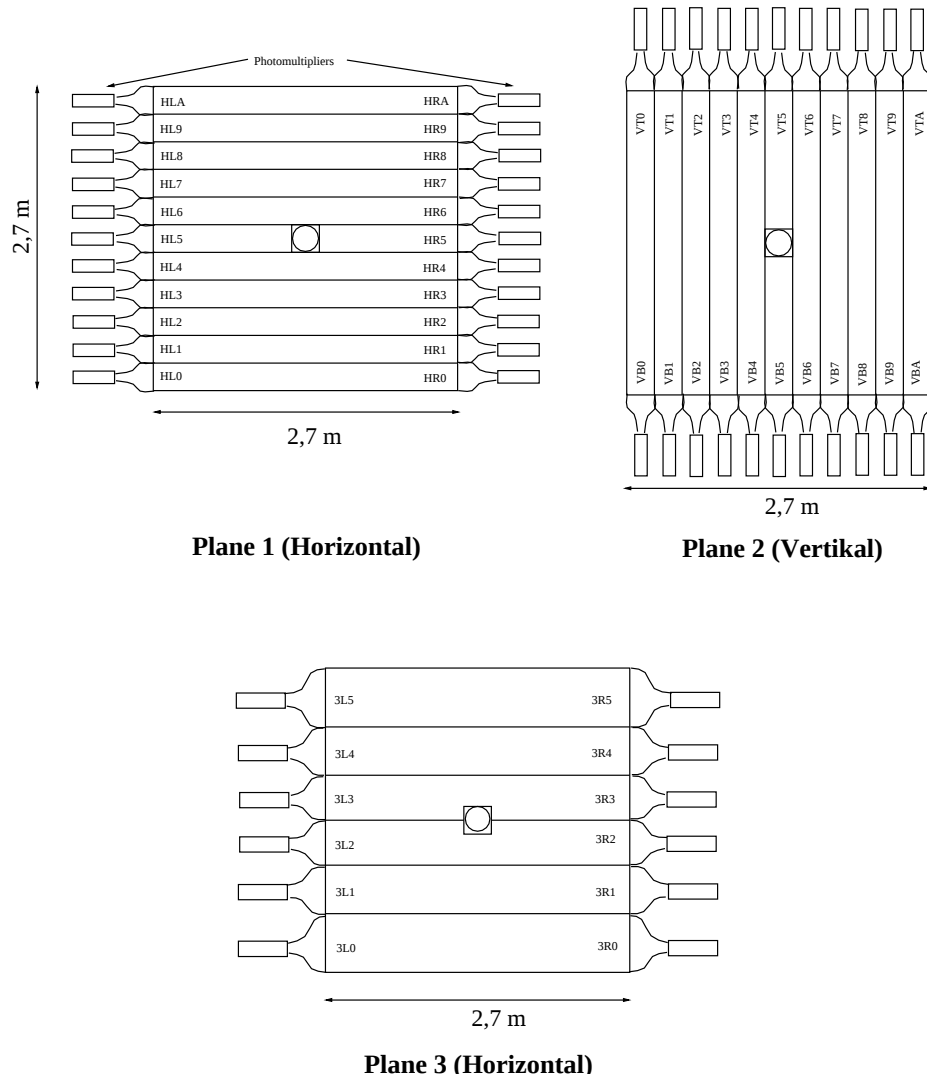
Abbildung 2.11: Aufbau des Myon-Antizählers (aus [NA48]).
