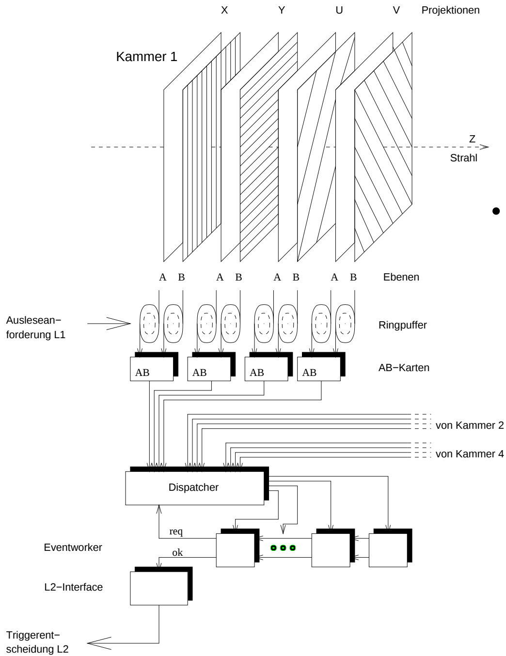
Abbildung 3.2: Übersicht über den Massbox-Trigger.
