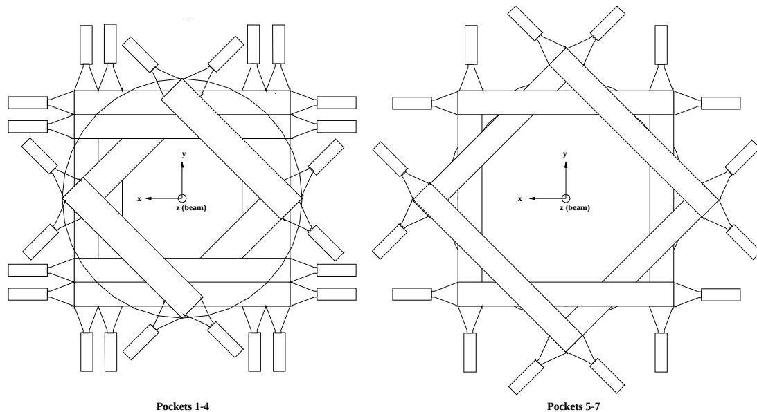
Abbildung 2.5: Aufbau der AKL-Antizähler (aus [NA48]).
