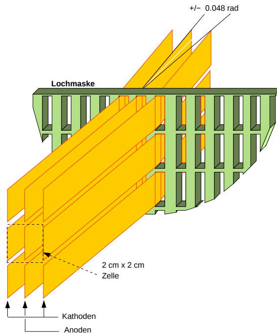
Abbildung 2.8: Aufbau des LKR-Kalorimeters. Eine Kalorimeterzelle wird von zwei Kathodenstreifen und einem Auslesestreifen auf positivem Potential gebildet.
