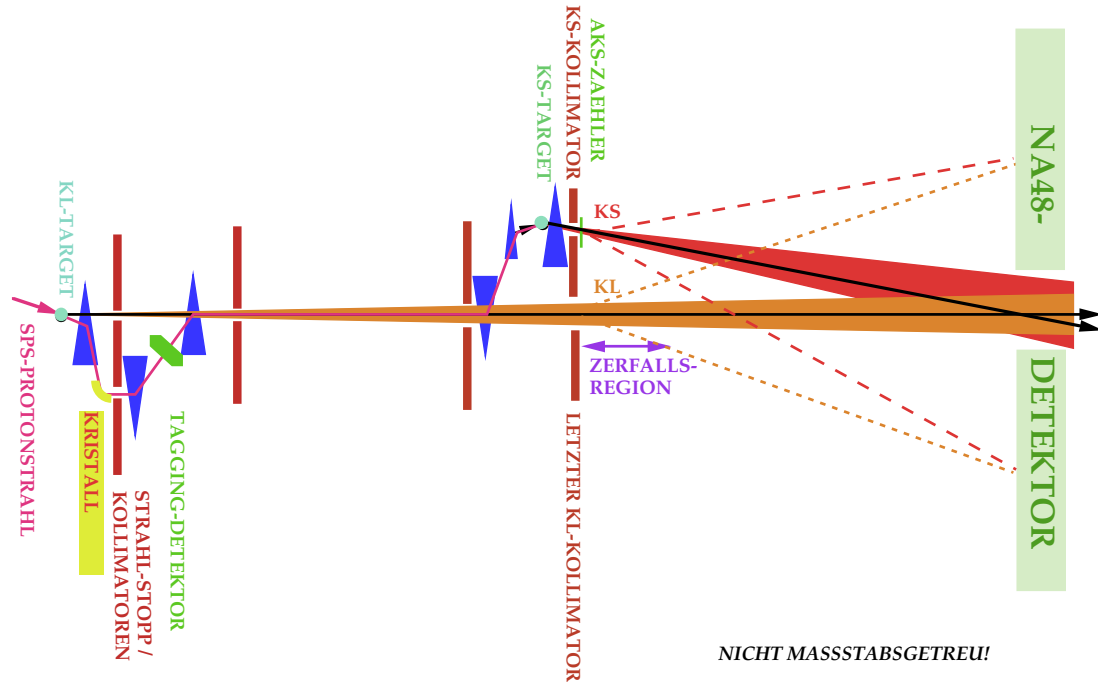
Abbildung 2.1: Prinzip der kollinearen K_L - und K_S -Strahlen.
