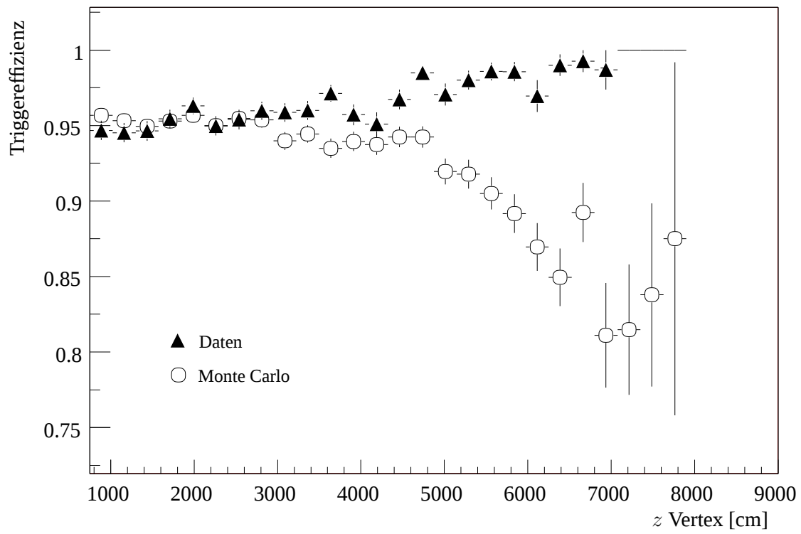
Abbildung 7.1: Vergleich der Effizienz des Vierspur-Triggers für K_L \rightarrow \pi^+ \pi^- \pi_D^0 -Daten- und Monte-Carlo-Ereignissen.
