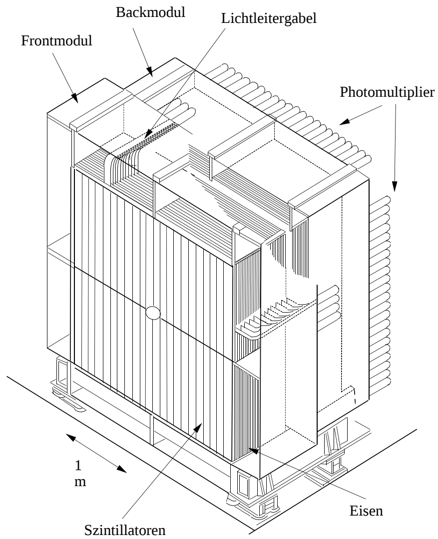
Abbildung 2.10: Das Hadron-Kalorimeter.
