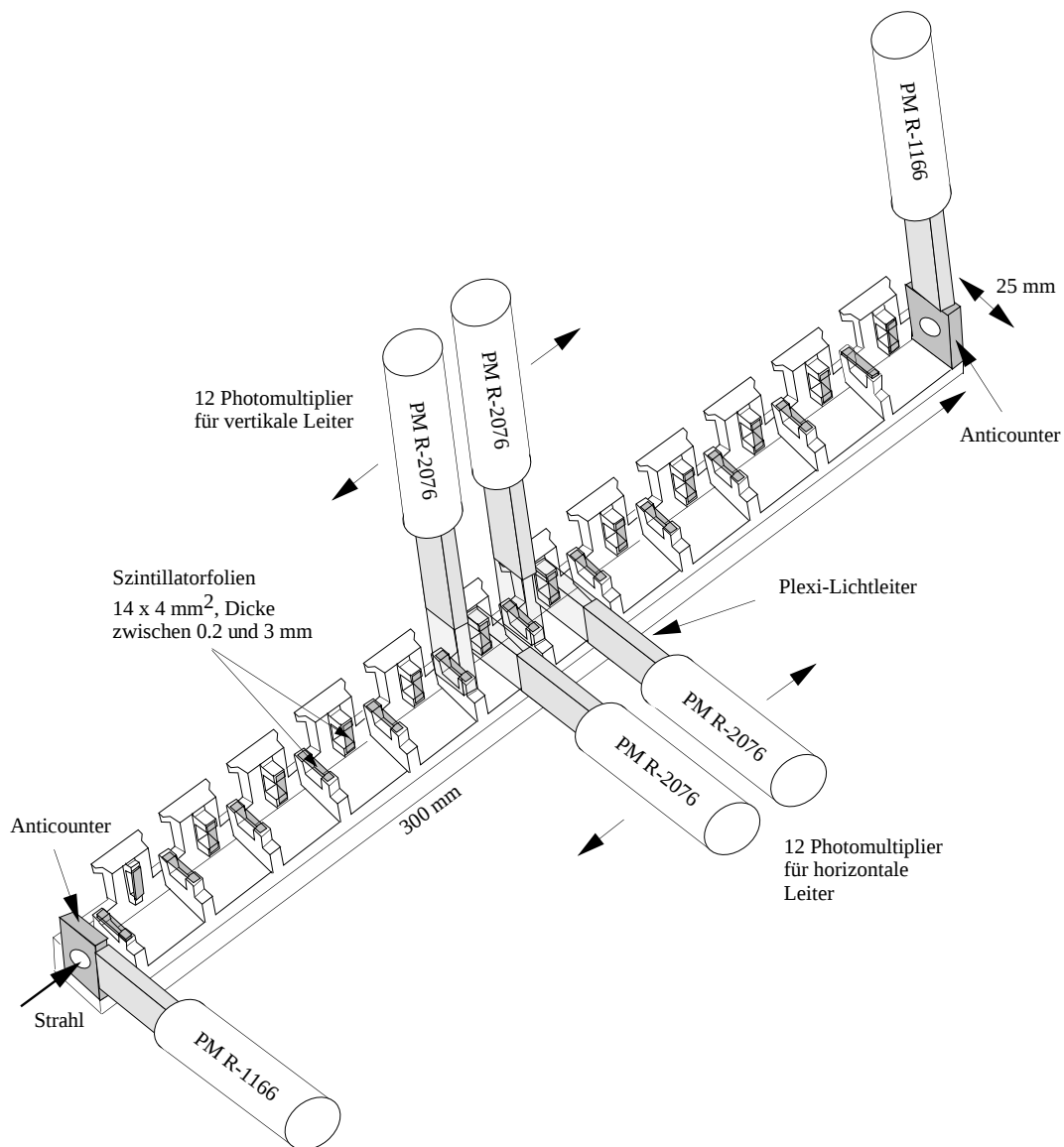
Abbildung 2.4: Der Tagging-Detektor.
