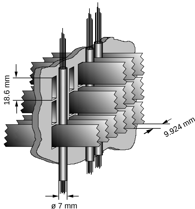
Abbildung 2.9: Fiberbündel des neutralen Hodoskops auf der 2. Lochmaske des LKR-Kalorimeters.
