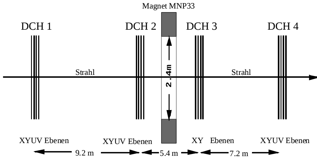
Abbildung 2.7: Das Magnetspektrometer.
