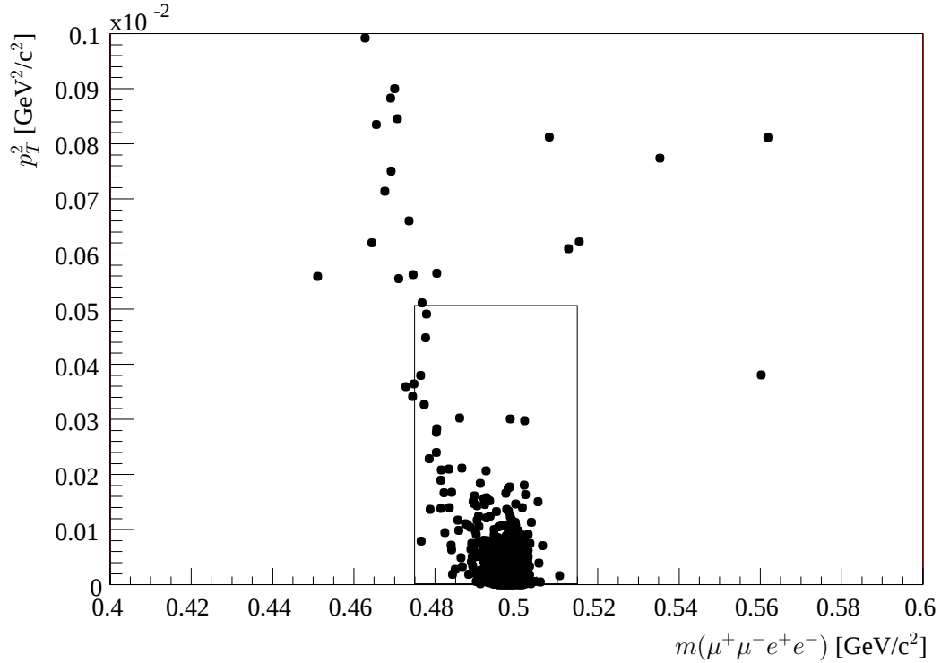
Abbildung 6.6: Das Quadrat des Transversalimpulses gegen die rekonstruierte Kaonmasse von K_L \rightarrow \mu^+\mu^-e^+e^- -Kandidaten aufgetragen. Oben für Daten-, unten für Monte-Carlo-Ereignisse.
