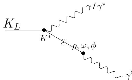
Abbildung 1.6: Feynman-Diagramm für den V-V Beitrag zur Zerfallsamplitude.
