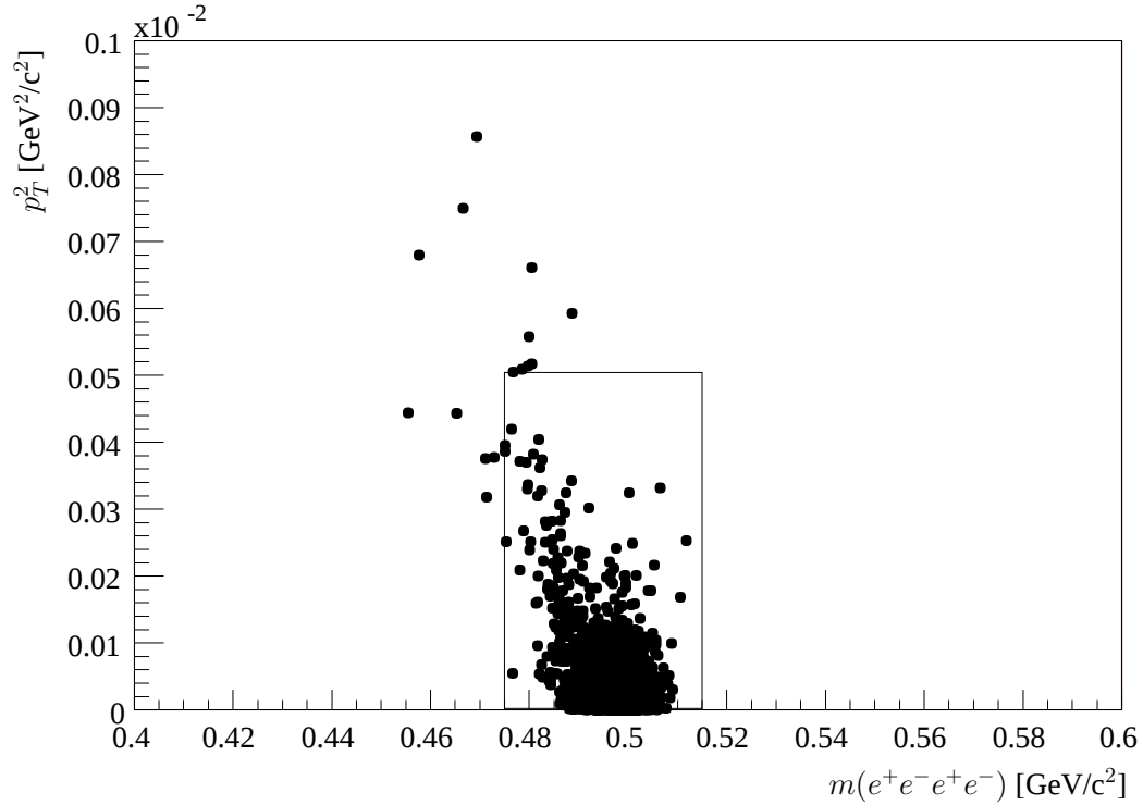
Abbildung 6.5: Das Quadrat des Transversalimpulses von K_L \rightarrow e^+e^-e^+e^- -Kandidaten gegen die rekonstruierte Kaonmasse aufgetragen. Oben für Daten-, unten für Monte-Carlo-Ereignisse.
