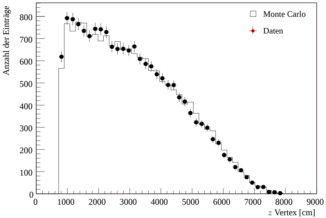
Abbildung 6.16: Vergleich der z -Vertexverteilung für K_L \rightarrow \pi^+\pi^-\pi^0 .
