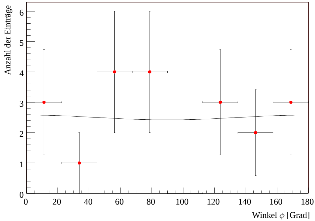
Abbildung 7.5: Winkel zwischen den von e^+e^- - und \mu^+\mu^- -Paaren aufgespannten Ebenen. Die Kurve ist die angepasste Funktion.
