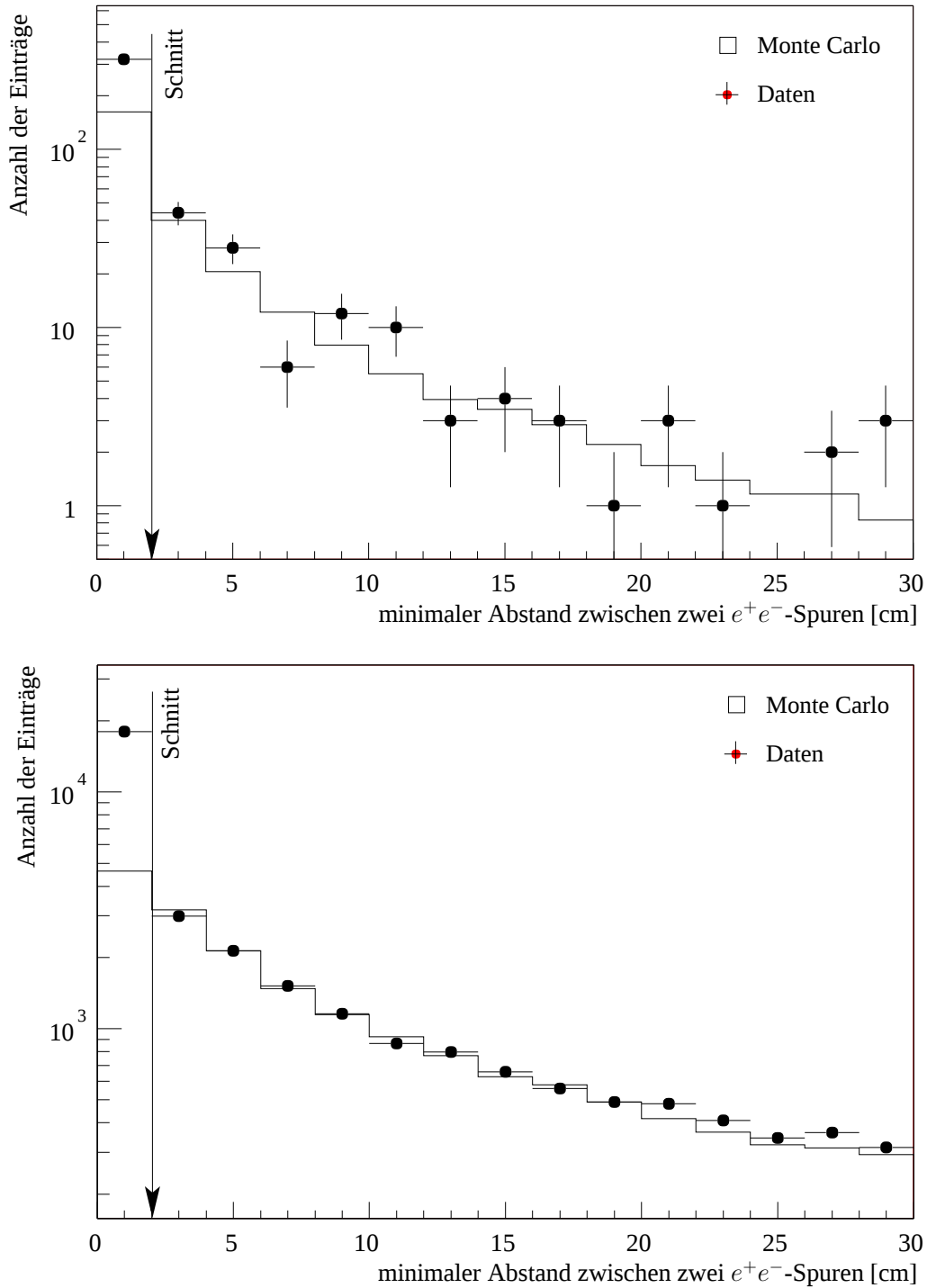
Abbildung 6.7: Der Spurabstand zwischen e^+e^- -Paaren in der ersten Driftkammer. Oben für K_L \rightarrow e^+e^-e^+e^- -Kandidaten, unten für K_L \rightarrow \pi^+\pi^-\pi_D^0 -Kandidaten. Der Überschuss von Datenereignissen für einen Spurabstand kleiner als 2 cm stammt von Konversionen am Detektormaterial.
