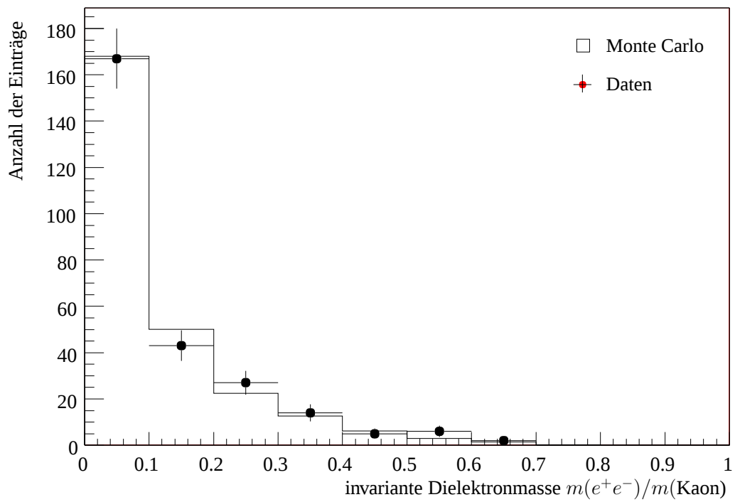
Abbildung 6.23: Vergleich der Dielektronmassen in Einheiten der Kaonmasse für K_L \rightarrow e^+e^-e^+e^- .
