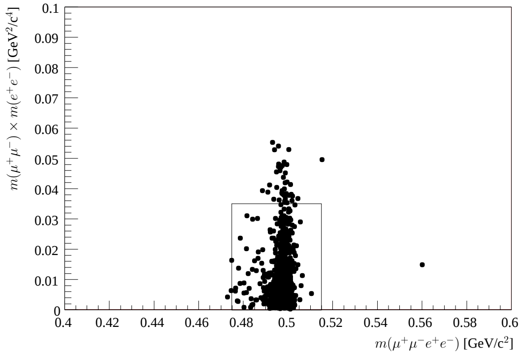
Abbildung 6.10: Das Produkt der Dimuon- und Dielektronmasse gegen die rekonstruierte \mu^+ \mu^- e^+ e^- -Masse. Oben für Daten-, unten für Monte-Carlo-Ereignisse.
