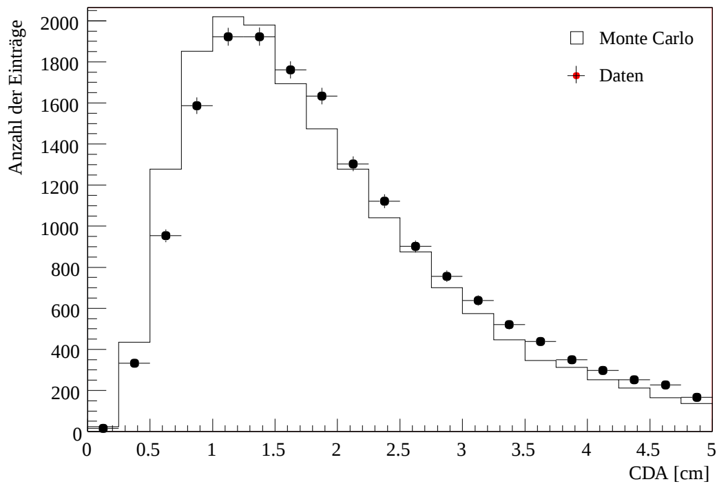
Abbildung 6.22: Vergleich der CDA-Verteilung K_L \rightarrow \pi^+\pi^-\pi_D^0 .
