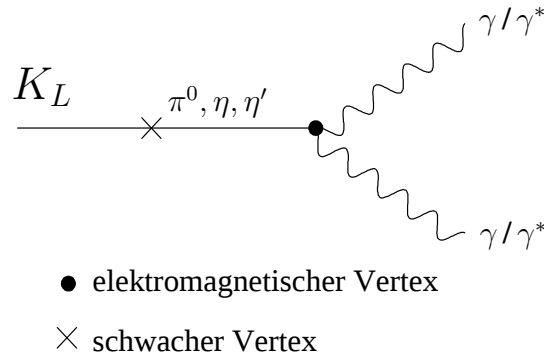
Abbildung 1.5: Feynman-Diagramm für den P-P Beitrag zur Zerfallsamplitude.
