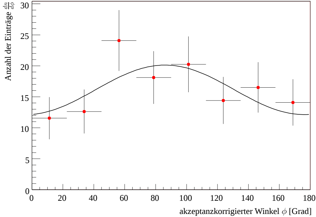
Abbildung 7.4: Winkel zwischen den von den beiden e^+e^- -Paaren aufgespannten Ebenen. Die Kurve zeigt die angepasste Funktion f(\phi) .
