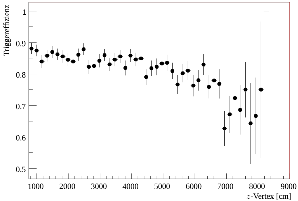
Abbildung 7.3: Effizienz des Vierspur-Triggers für K_L \rightarrow \mu^+\mu^-e^+e^- -Monte-Carlo-Ereignisse.
