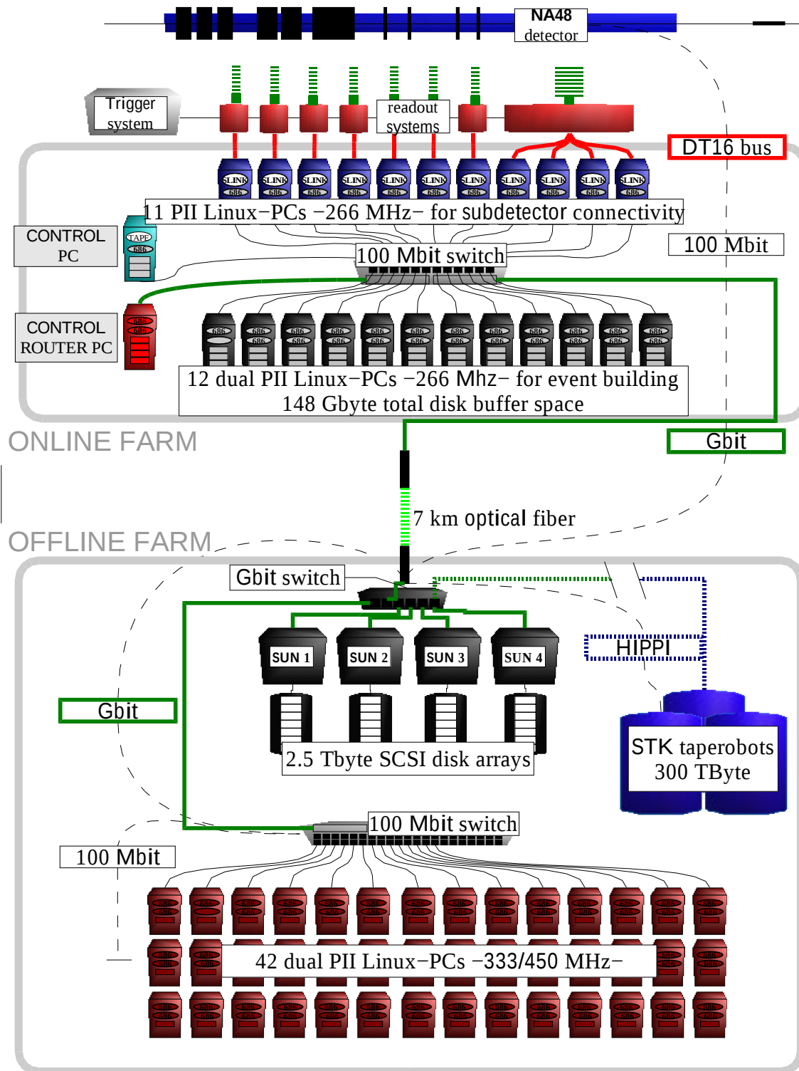
Abbildung 3.3: Aufbau der PC-Farm 1999.
