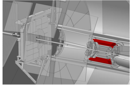
(d) The SSD layers
