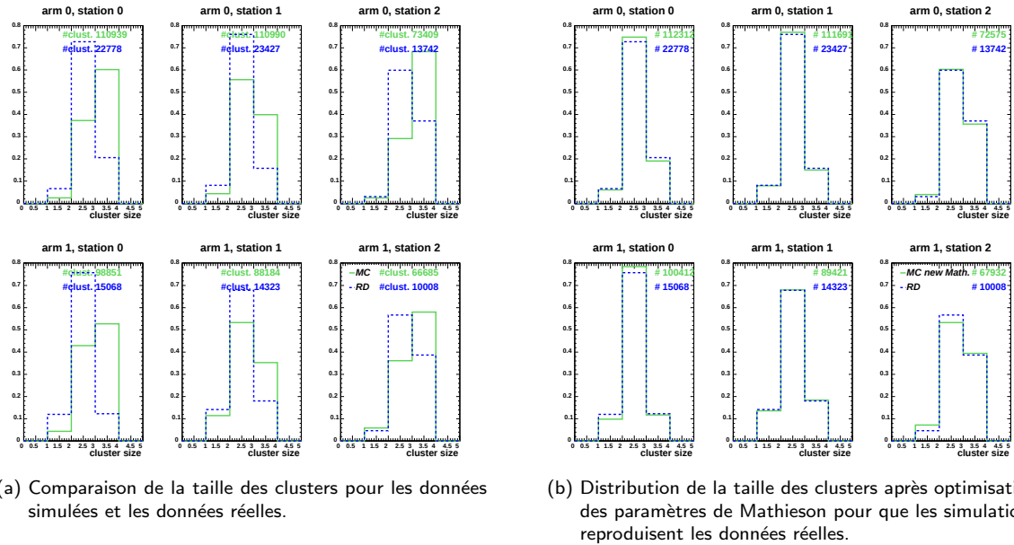
Fig. III.35 – Comparaison de la distribution de la taille des clusters avec les paramètres initiaux et optimisés pour que cette distribution des données réelles soit bien reproduite par les simulations.
