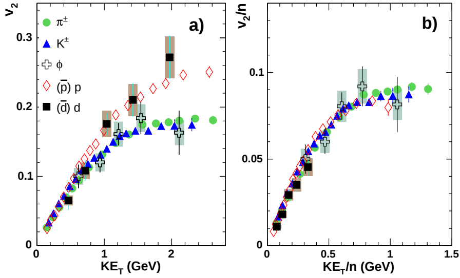
Fig. 1.33 – (a) Flot elliptique v_2 en fonction de l'énergie cinétique transverse kE_T pour plusieurs particules identifiées (pions, kaons, phi, protons, deutérons) à centralité [20-60]%) dans les collisions. (b) v_2/n en fonction de kE_T/n_q pour les mêmes particules [192]
