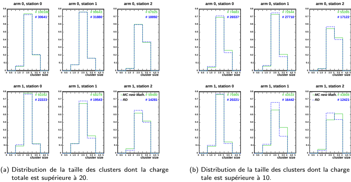
Fig. III.41 – Comparaison de distribution de la taille des clusters pour deux coupures sur la charge totale.
