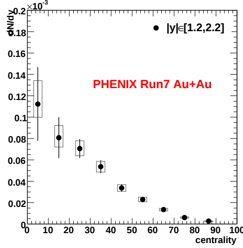
Fig. V.10 – Taux de production du J/\psi en fonction de la centralité, intégré sur tout le spectre en p_T .
