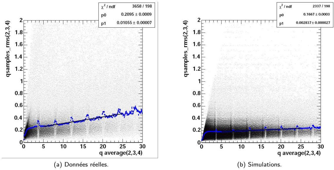
Fig. III.46 – Distributions des écarts types des trois échantillons utilisés pour calculer la charge totale en fonction de la valeur moyenne de la charge totale.
