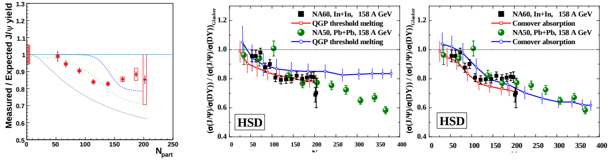
Fig. I.21 – Gauche : Production du J/\psi mesurée par NA60 dans les collisions In+In à 158 GeV au SPS [135] comparée à des prédictions théoriques basées sur (a) un scénario de fonte séquentielle dans un QGP [89] (ligne supérieure en pointillée), (b) suppression dans le QGP et la phase hadronique dans une boule de feu thermique [133] (ligne centrale en tireté), et (c) dans un modèle de co-voyageurs [116] (ligne inférieure). Tous ces modèles sont en relativement bon accord avec les données de NA50 pour les collisions Pb+Pb. Droite : Production du J/\psi dans les collisions Pb+Pb [136] et In+In [137] obtenue avec le modèle de transport HSD [134] en utilisant également soit un scénario de fonte séquentielle dans un QGP (centre) soit un modèle de co-voyageurs (droite).
