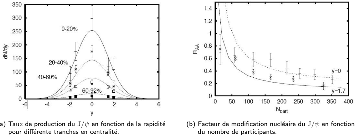
Fig. 1.25 – Production du J/\psi dans les collisions Au+Au mesurée par PHENIX à rapidité nulle et positive [140] comparée aux prédictions de effets de la saturation de gluons [143].
