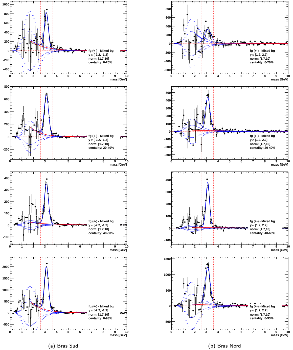
Fig. V.6 – Distributions de la masse invariante obtenues avec la soustraction du bruit de fond combinée pour différents centrages.
