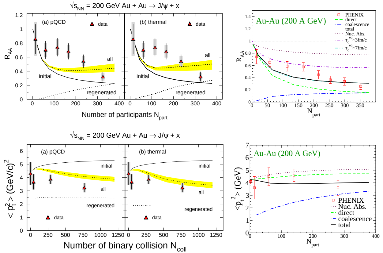
Fig. I.30 – Production du J/\psi dans les collisions Au+Au à RHIC calculée selon des équations de taux cinétique dans un milieu en évolution thermique, ce qui correspond à l'approche comparée aux données de SPS à la Fig. I.21. Panneaux de gauche : dissociation gluonique dans une simulation dynamique [149, 148] avec l'énergie de liaison dans le vide. Panneaux de droite : dissociation quasi libre dans une boule de feu en expansion thermique avec l'énergie de liaison du milieu [123, 132]. Les panneaux du haut montrent le facteur de modification nucléaire en fonction du nombre de participants pour les taux de production du J/\psi inclusifs. Les panneaux du bas montrent la dépendance en centralité de l'impulsion transverse moyenne du J/\psi au carré. Les données correspondent aux données préliminaires [140, 150] mais les conclusions ne changent pas avec les données finales. Ces prédictions n'ont été réalisées que pour la rapidité nulle.
