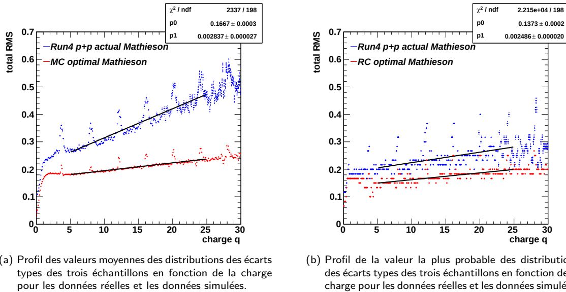
Fig. III.47 – Distributions des écarts types des trois échantillons utilisés pour calculer la charge totale en fonction de la valeur moyenne de la charge totale.
