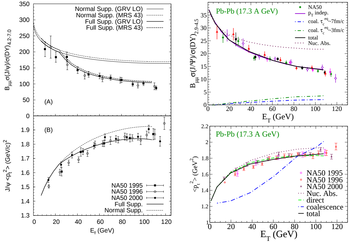
Fig. I.20 – Production du J/\psi dans les collisions Pb+Pb à SPS en fonction de l'énergie transverse avec plusieurs prédictions (voir texte) : (haut) rapport de modification nucléaire, et (bas) impulsion transverse moyenne au carré.
