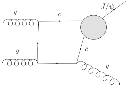
(a) Exemple de diagramme d'ordre le plus bas pour la production directe de J/\psi à partir de la fusion de gluons dans le cadre du CSM. La paire c\bar{c} est dans l'état de singlet de couleur.
