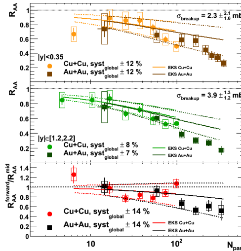
Fig. I.23 – Rapport de modification nucléaire de la production du J/\psi mesuré par PHENIX dans les collisions Au+Au [140] et Cu+Cu [139]. Les lignes correspondent à un modèle de shadowing EKS auquel est ajouté une section efficace d'absorption nucléaire ajustée sur les données d+Au, l'ensemble étant extrapolé aux collisions Cu+Cu et Au+Au.
