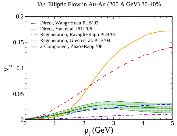
(b) Prédictions de modèles de coalescence et de suppression du J/\psi en utilisant une approche de boule de feu et de dissociation presque libre [132, 202].
