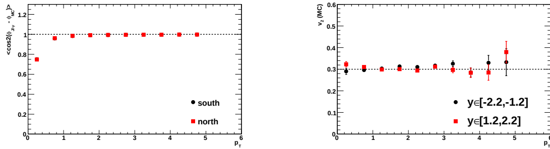
(a) Facteur de correction lié à la résolution finie de l'angle reconstruit \phi du J/\psi en fonction de p_T .
