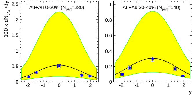
(b) Production du J/\psi en fonction de la rapidité dans les collisions Au+Au par PHENIX.
