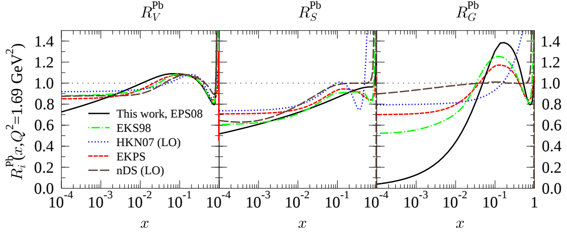
Fig. I.15 – Comparaison des modifications moyennes des quarks de valence et de la mer, ainsi que des gluons à Q^2 = 1,69 \text{ GeV}^2 pour des noyaux Pb à partir des analyses LO DGLAP globales EKS98, HKN07, nDS, EPS08 et NLO EKPS [84].
