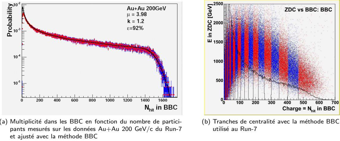
Fig. II.5 – Variables globales mesurées avec la nouvelle méthode BBC.
