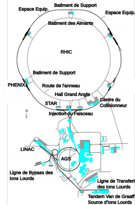
Fig. II.1 – Vue d'ensemble de l'accélérateur RHIC
