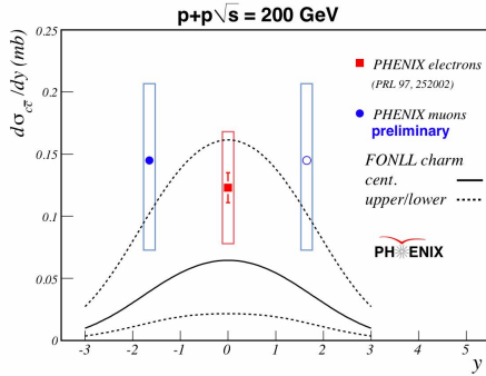
(a) Mesures du charme ouvert par PHENIX et STAR en fonction de la rapidité comparées à des prédictions FONLL.
