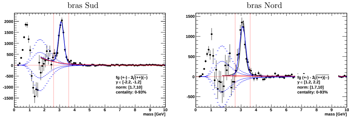
Fig. V.3 – Distribution de la masse invariante des paires de muons obtenue avec la méthode de soustraction des paires de même signe pour la centralité [0,93]\% , à gauche pour le bras Sud et à droite pour le bras Nord.
