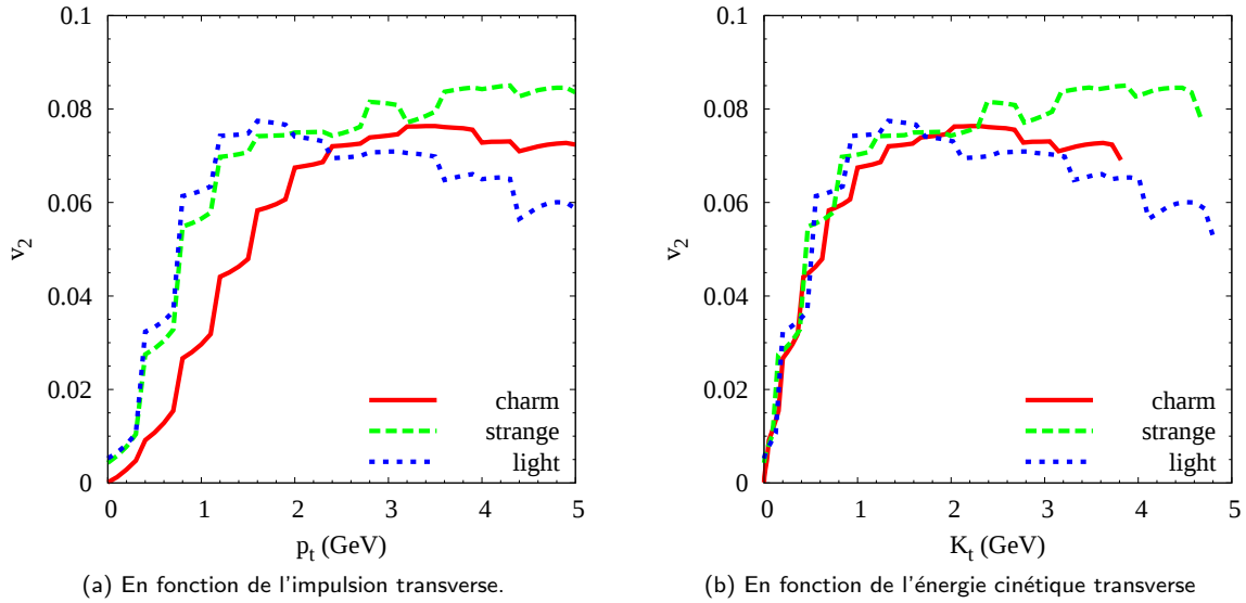
Fig. I.35 – Prédiction du modèle [198] du flot elliptique v_2 des quarks c , s et quarks légers, pour collisions Au+Au à \sqrt{s_{NN}} = 200 GeV et à rapidité nulle.
