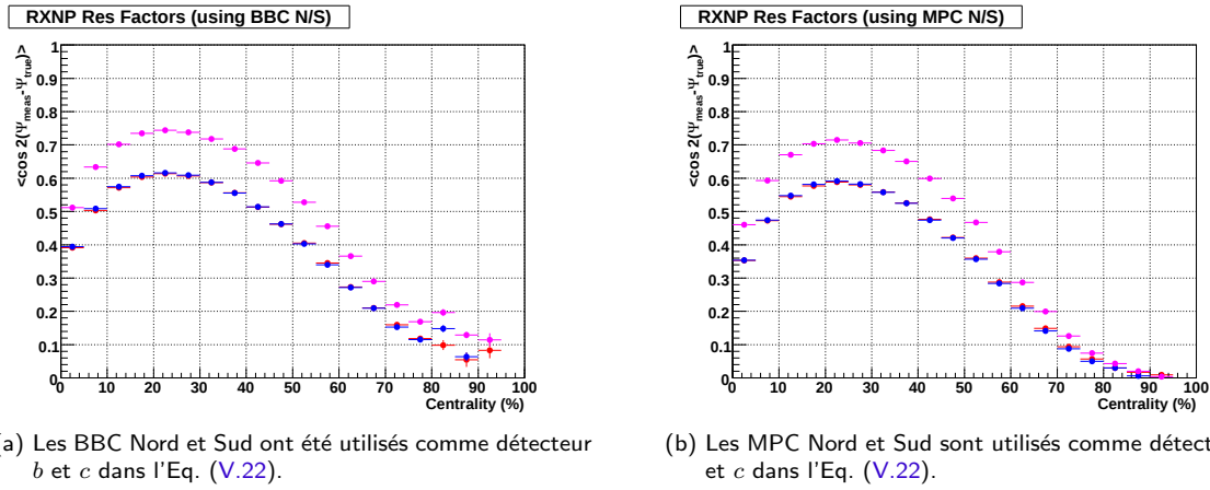
Fig. V.11 – Correction \sigma_{RP} en fonction de la centralité pour le RxnP Nord (bleu), Sud (rouge) et Nord+Sud combinés (magenta).
