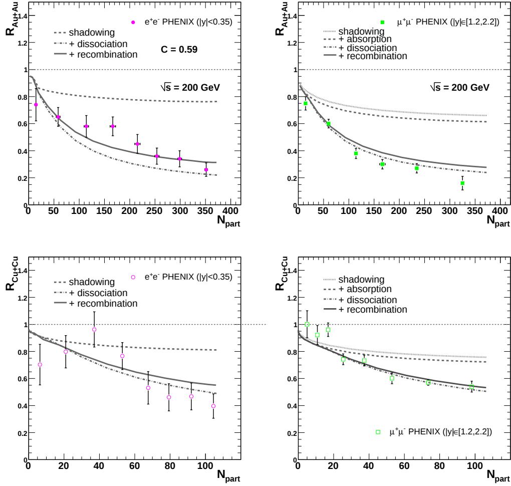
Fig. 1.29 – Facteur de modification nucléaire en fonction du nombre de participants mesuré par PHENIX dans les collisions Au+Au [140] comparé à des prédictions incluant shadowing, absorption, dissociation, et recombinaison [146].
