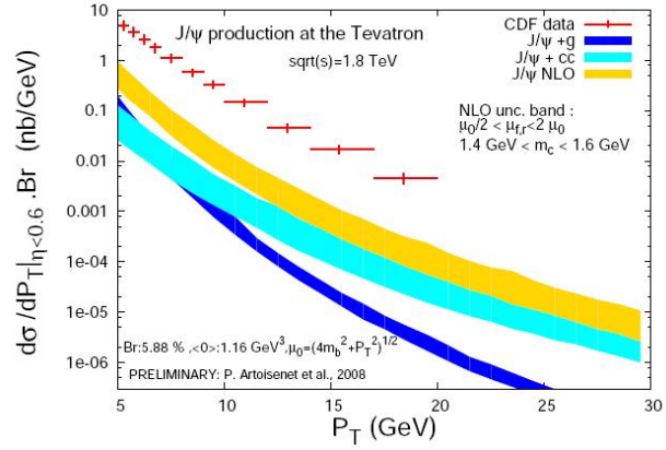
(b) Production du J/\psi mesurée au Tevatron à \sqrt{1.8} TeV comparé à des modèles de singlet de couleur à l'ordre dominant et suivant.
