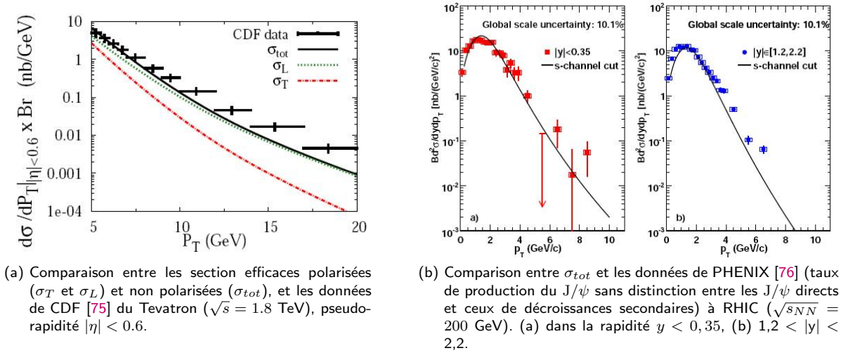
Fig. 1.12 – Résultat de l'ajout de la coupure sur le canal s au CSM.
