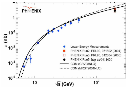
(b) Section efficace totale de production du J/\psi en fonction de l'énergie de la collisions.
