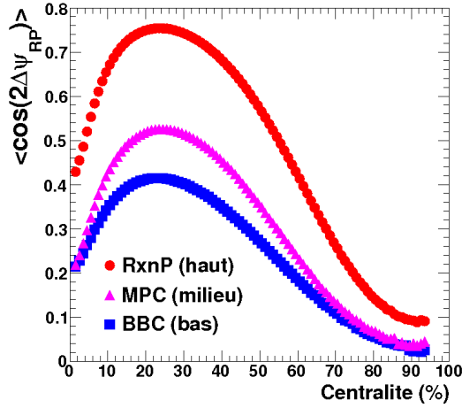
Fig. II.6 – Indicateur de la résolution du plan de réaction mesurée par les BBC (cercles rouges), par les MPC (triangles magenta) et par les RxnP (carrés bleus). Plus \langle \cos(2\Delta_{RP}) \rangle est grand, plus les informations sur le plan de réaction sont précises.
