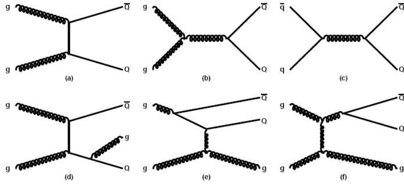
Fig. I.6 – Exemple de diagrammes de production de la paire de quarks lourds. (a),(b) fusion de gluons au premier ordre, (c) annihilation de la paire au premier ordre, (d) création de la paire avec émission de gluon, excitation de couleur, (e) et (f) division de gluon [47]
