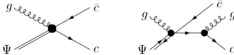
Fig. 1.18 – Réactions de dissociation des charmonia par interactions partoniques. À gauche : dissociation gluonique représentant le processus de QCD à l'ordre dominant LO de gluo-dissociation [124, 125] ; à droite : la dissociation quasi libre qui représente le processus à l'ordre suivant NLO de la dissociation [126].
