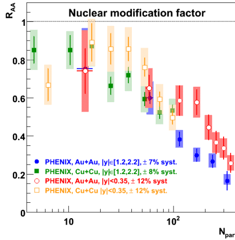
Fig. I.22 – Facteur de modification nucléaire en fonction du nombre de participants N_{part} pour les collisions Cu+Cu [139] et Au+Au [140] à \sqrt{s_{NN}} = 200 GeV à rapidité nulle et à rapidité positive.
