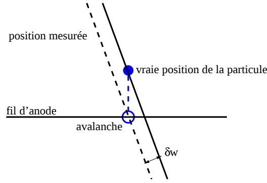
Fig. III.1 – Biais entre la position de la particule (dans la direction perpendiculaire aux pistes) et la position mesurée dans une cathodes où l'orientation des anodes n'est pas perpendiculaire aux pistes.
