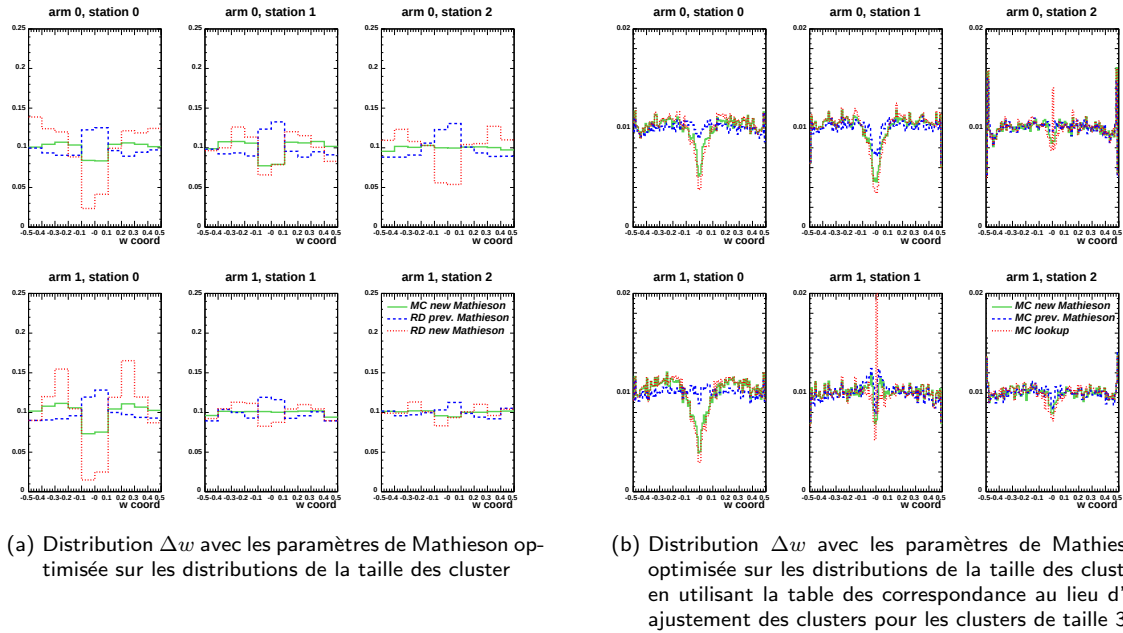
Fig. III.36 – Comparaison de la distribution \Delta w avec les paramètres de Mathieson optimisés sur les distributions de la taille des clusters avec et sans ajustement des clusters.
