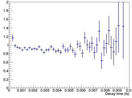
(a) p_\pi/p_{B_c} < 12.5\%
