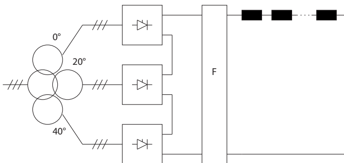
(c) montage à convertisseur de courant 18 pulsations
