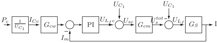
FIG. 6.27: Diagramme structurel du système de chargeur avec sa commande associée
