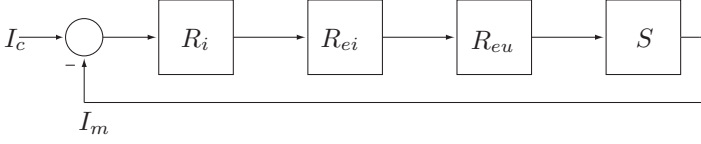
FIG. 4.1: Schéma de réglage comprenant : régulateur de courant principal R_i , régulateur d'équilibrage de courant R_{ei} et de tension R_{eu} pour le système S
