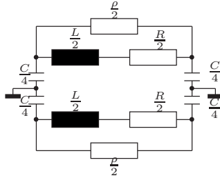
FIG. 1.3: Schéma équivalent d'un aimant du PS
