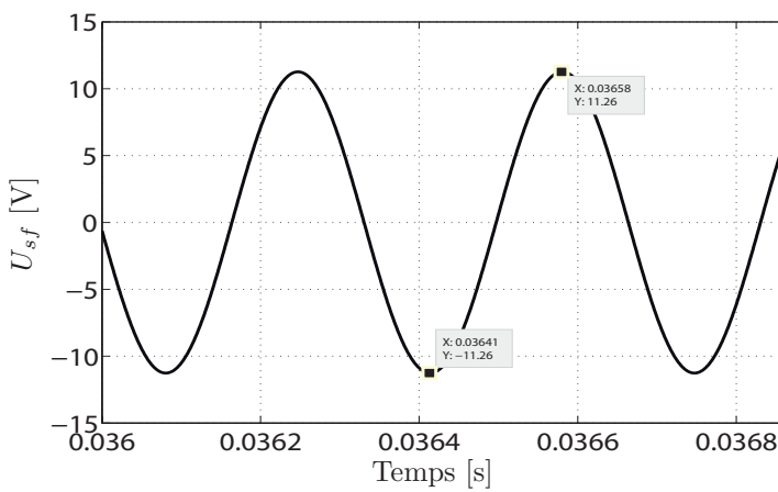
FIG. 3.5: Ondulation de tension
