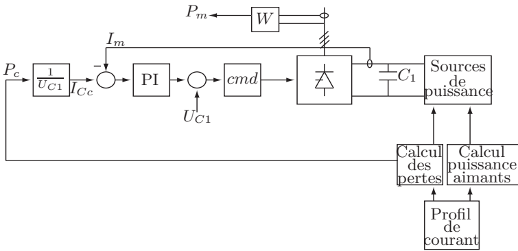
FIG. 6.26: Diagramme structurel de réglage pour l'étude des chargeurs
