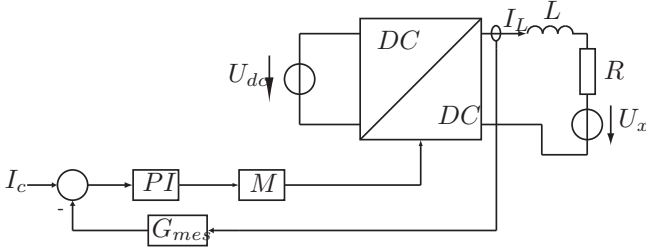
FIG. 5.6: Schéma de simulation pour un seul convertisseur
