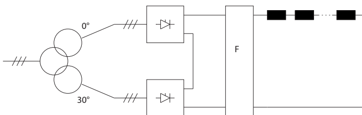
(b) montage à convertisseur de courant 12 pulsations
