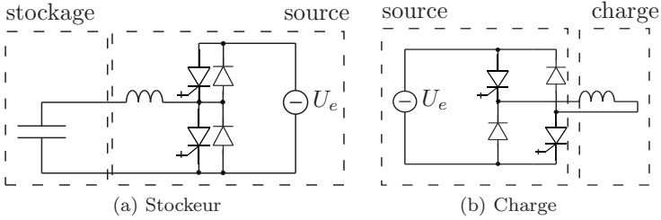
FIG. 2.4: Convertisseurs élémentaires
