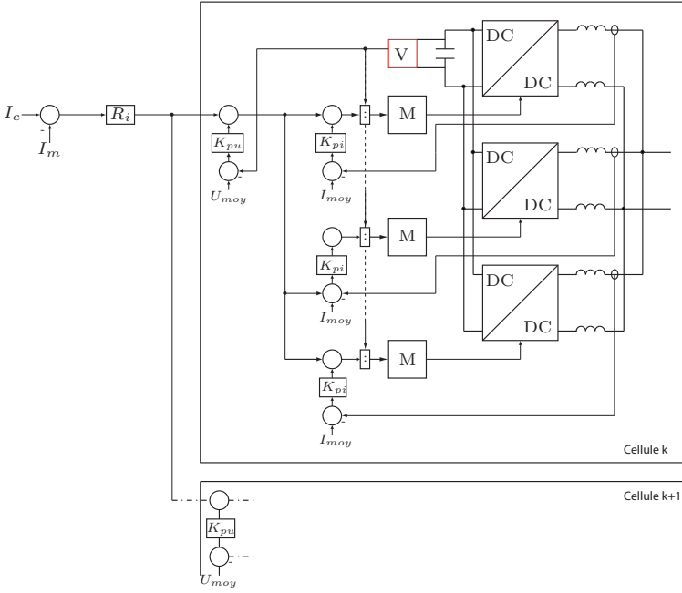
FIG. 4.11: Schéma du système de réglage par cellule
