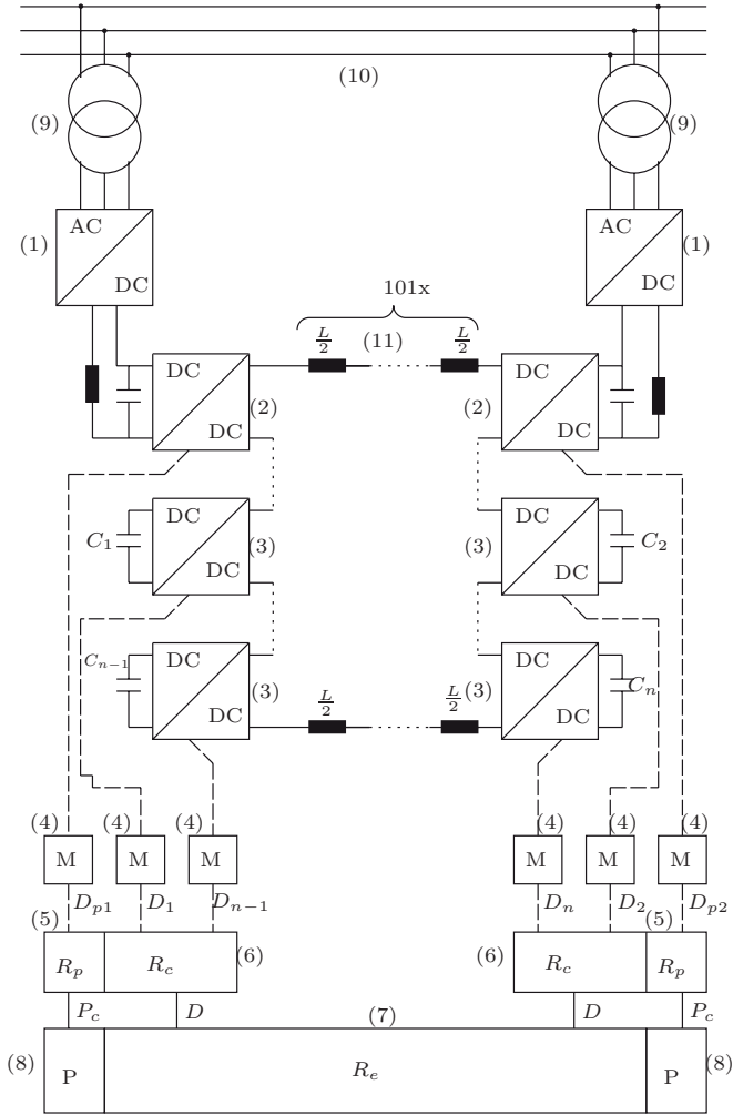
FIG. 2.10: Schéma du système d'alimentation proposé
