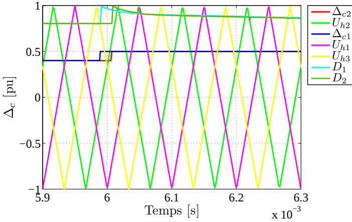
FIG. 5.15: Sauts de consigne décalés
