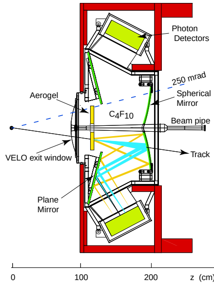
Figura 4.9: Visão esquemática do RICH1, mostrando o caminho dos fótons até os fotodetectores. Os últimos são localizados fora da aceitação do detector para evitar efeitos do campo magnético e livrar a eletrônica de danos causados pela intensa radiação nas proximidades do feixe.
