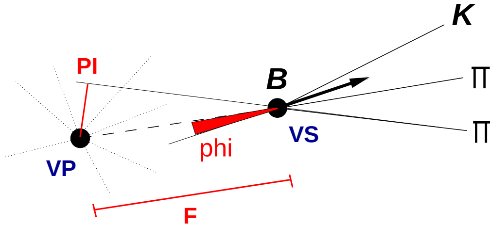
Figura 6.1: Topologia do decaimento B^\pm \rightarrow K^\pm \pi^+ \pi^- . A partícula B criada no vértice primário VP viaja uma distância F antes de decair no vértice secundário VS. Na figura também pode ser visto o parâmetro de impacto PI de uma das partículas filhas e o ângulo \phi entre o 3-momento reconstruído de B e a reta que liga os vértices.
