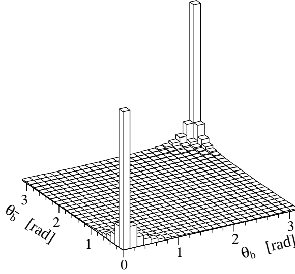
Figura 4.3: Ângulos de produção de b ( \theta_b ) e \bar{b} ( \theta_{\bar{b}} ) nas colisões próton-próton do LHC, calculados pelo gerador de eventos PYTHIA.
