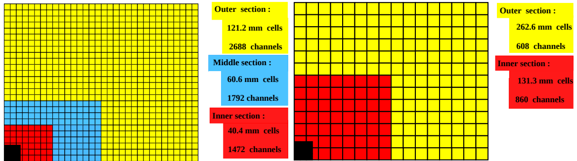
Figura 4.10: Visão esquemática \frac{1}{4} da segmentação das células no ECAL, SPD e PS à esquerda e no HCAL à direita. Os quadros mostram o tamanho das células e a quantidade de canais de leitura em cada região.
