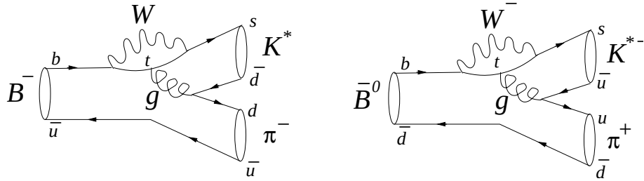
Figura 5.1: Diagramas pingüim de B^- \rightarrow K^*\pi^- e \bar{B}^0 \rightarrow K^{*-}\pi^+ com mesma amplitude a_P e^{i\delta_P} de acordo com a simetria de sabor SU(3).
