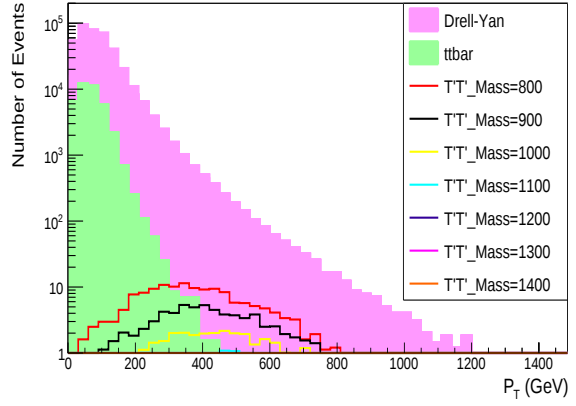
Dimuon p_T .
