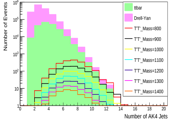
Number of AK4 jets ( e^+e^- + \mu^+\mu^- channel).
