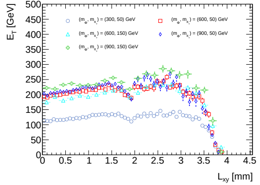
(d) High \Phi masses, non-triggering \pi_v
