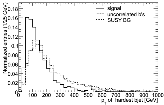
(1) hardest b -jet
