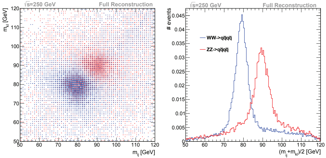
FIGURE 7.7 – (a) : Masse des di-jets reconstruits pour des simulations d'événements e^+e^- \rightarrow W^+W^- (en bleu) et e^+e^- \rightarrow ZZ (en rouge) à \sqrt{s} = 250 GeV. (b) : Distribution de la masse moyenne des di-jets reconstruits (m_{ij} + m_{ik})/2 . Ces distributions sont normalisées aux nombres d'événements. Les événements sont reconstruits dans une simulation complète de l'ILD avec le SDHCAL.
