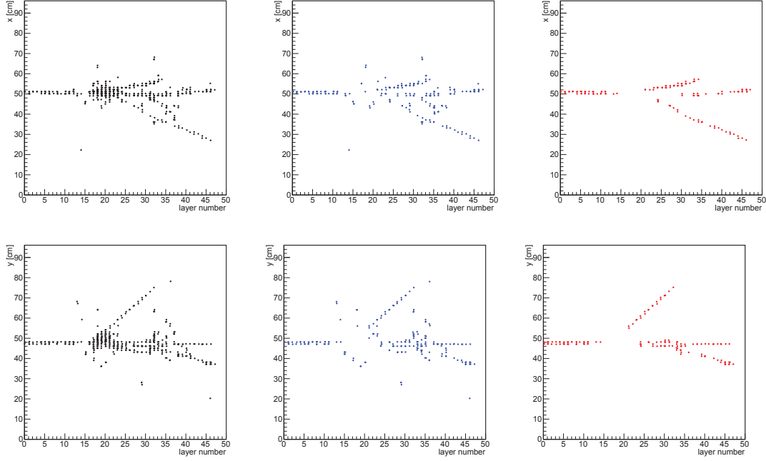
FIGURE 6.12 – Image d’une gerbe hadronique de 30 GeV dans le SDHCAL dans le plan ( xOz ) (en haut) et le plan ( yOz ) (en bas) illustrant les différentes étapes de la reconstruction des traces. La colonne de gauche montre tous les hits de l’événement, la colonne du milieu présente les hits appartenant aux amas de la partie non dense et la colonne de droite présente les hits le long des traces reconstruites par la méthode de transformée de Hough.
