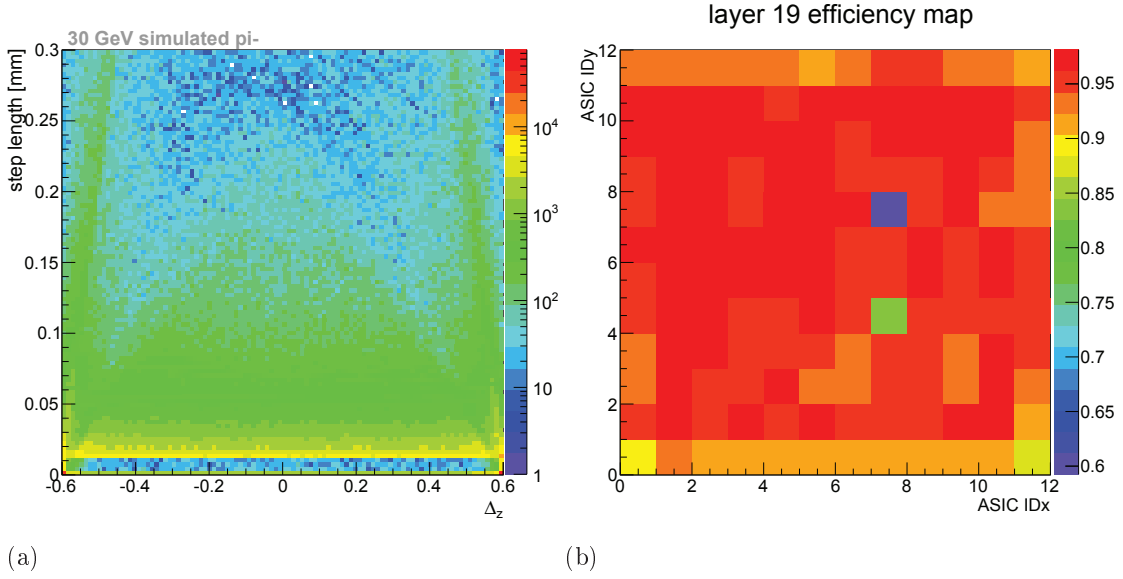
FIGURE 5.4 – (a) : Longueur des segments ( step length ) en mm en fonction de \Delta_z en mm . Cette figure est centrée sur la région des segments de faible longueur pour mettre en évidence le fait que la plupart des segments de longueur nulle (ou presque) sont localisés sur les bords de la couche de gaz ( |\Delta_z| \simeq 0.6 \text{ mm} ). (b) : Exemple d'une carte d'efficacité des ASICs.
