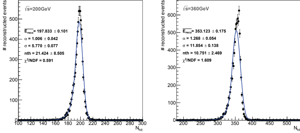
FIGURE 7.4 – Energie totale reconstruite pour des événements e^+e^- \rightarrow Z \rightarrow q\bar{q} à \sqrt{s} = 200 (à gauche) et 360 (à droite) \text{GeV} .
