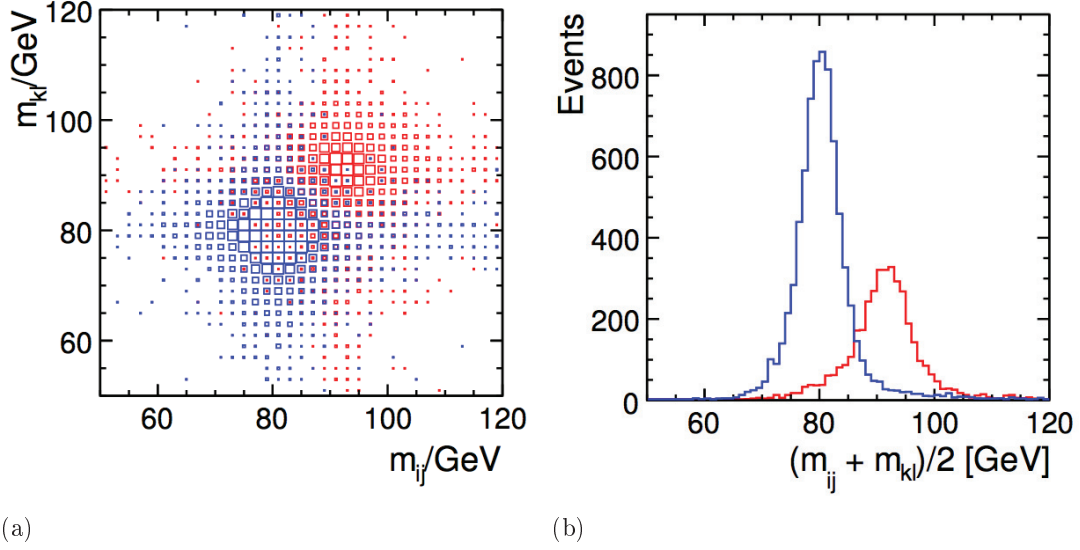
FIGURE 7.2 – (a) : Masse des di-jets reconstruits pour des simulations d'événements e^+e^- \rightarrow \nu_e \bar{\nu}_e W^+W^- (en bleu) et e^+e^- \rightarrow \nu_e \bar{\nu}_e ZZ (en rouge) à \sqrt{s} = 1 \text{ TeV} . (b) : Distribution de la masse moyenne des di-jets reconstruits (m_{ij} + m_{ik})/2 pour les événements e^+e^- \rightarrow \nu_e \bar{\nu}_e W^+W^- (en bleu) et e^+e^- \rightarrow \nu_e \bar{\nu}_e ZZ (en rouge) [5].
