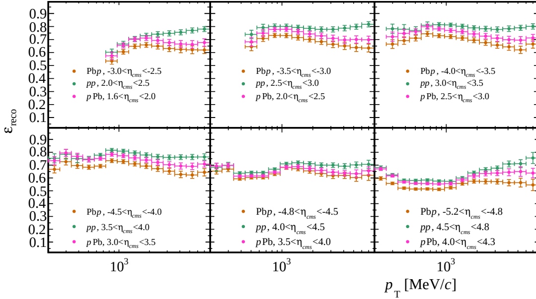
Figure A.1: Eficiencia de reconstrución \varepsilon_{\text{reco}} para colisións Pb p , pPb e pp .
