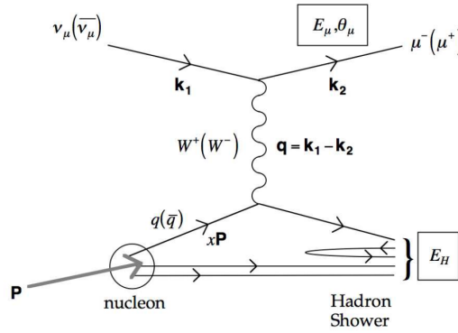
Figure 1.: Diagramme de Feynman pour un processus de DIS de neutrinos CC. Le diagramme est reproduit à partir de [41] .
