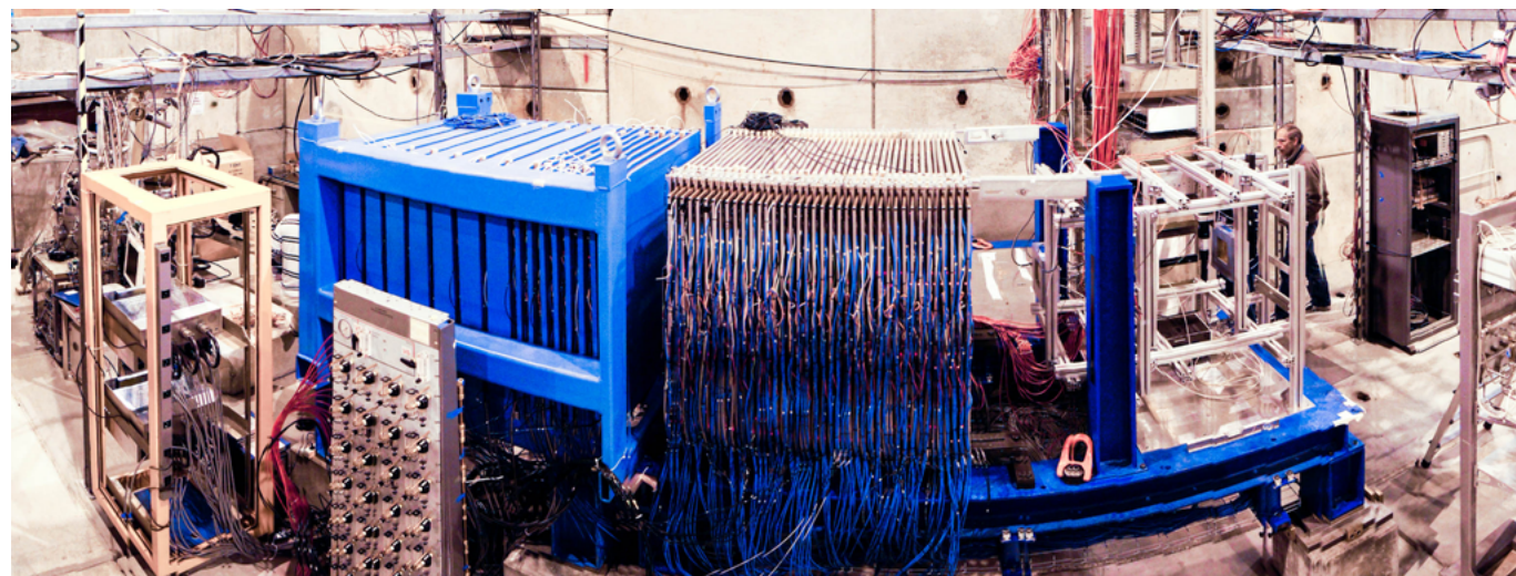
Le prototype de calorimètre en tungstène de CALICE en phase de test au CERN. Ce prototype de calorimètre hadronique d'un mètre cube possède près de 500 000 canaux électroniques à lecture indépendante, soit plus que tous les calorimètres d'ATLAS et de CMS réunis.
