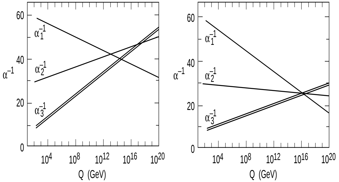
Figure 3: a) Le \overline{MS} n'assure pas l'unification des constantes de couplage électrofaible et forte par contre b) le MSSM permet cette unification.
