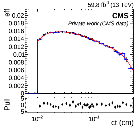
(d) PDL efficiency in dataset_JpsiTrkTrk (2018).
