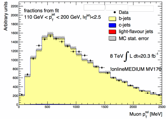
(d) Fit to the \overline{\text{trig}}|\text{tag} -distribution.
