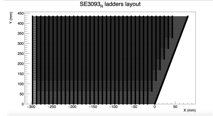
Figure 4.42: Eta PCB ladder layout.
