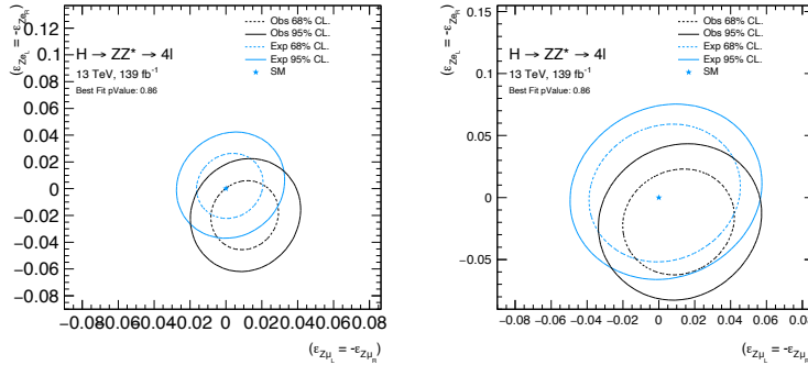
(d) Flavour non-universal axial contact terms
