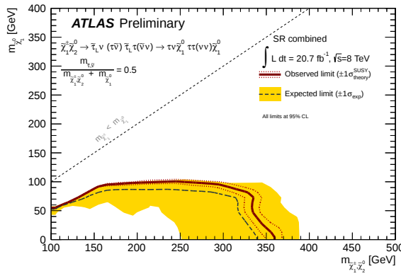
(a) C_1 N_2 production
