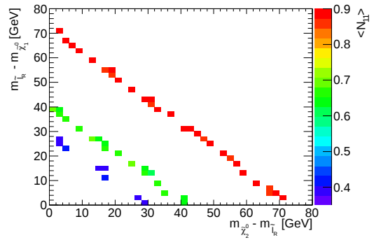
(d) Neutralino and slepton mass differences
