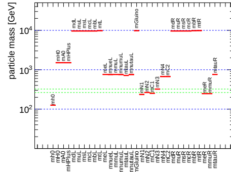
(d) M_1 = 300 GeV, M_2 = 600 GeV, \mu = 250 GeV
