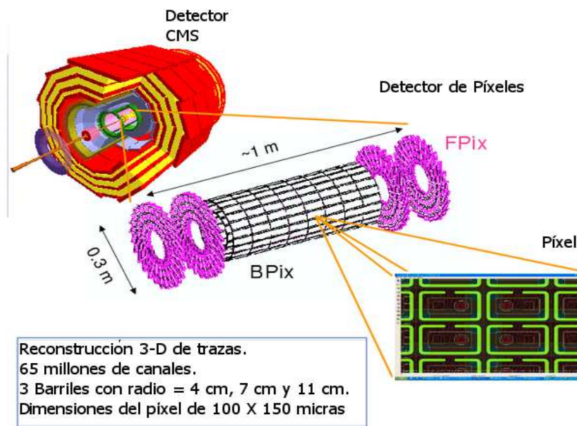
Figura 2-3: configuración del detector de píxeles [2].
