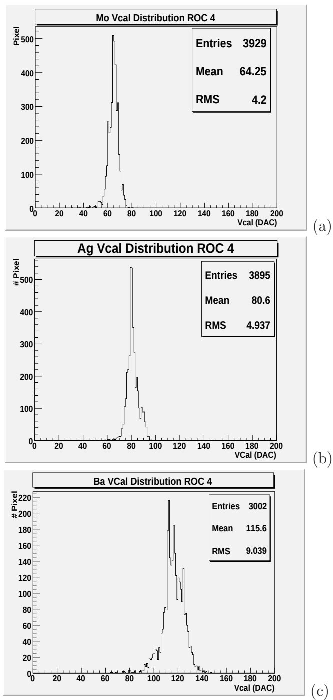
Figura 8-2: Distribuciones de VCal para el ROC 4, (a) Mo, (b) Ag y (c) Ba
