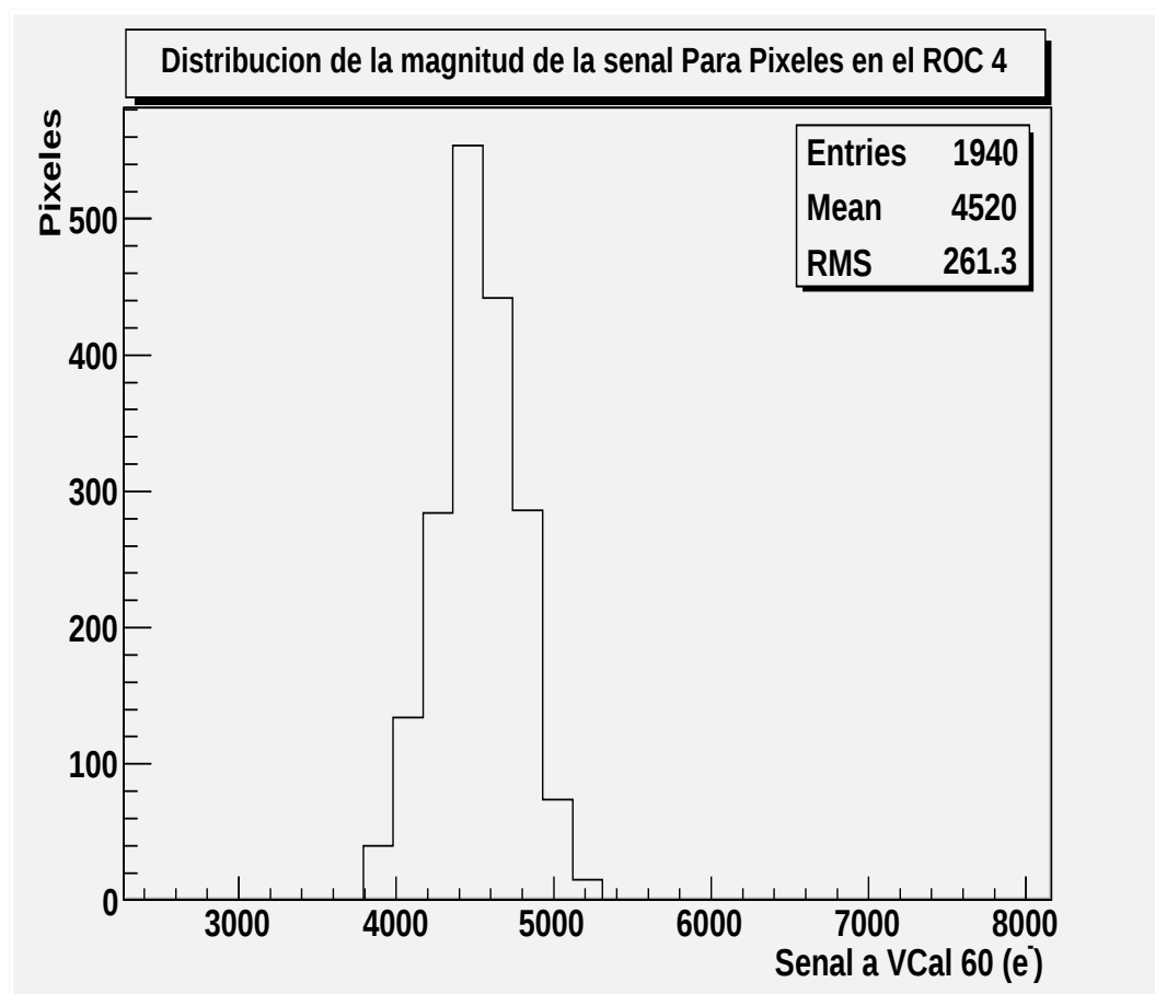
Figura 8–6: Distribución de la magnitud de la señal en electrones para una inyección de carga Vcal 60 en el ROC 4.
