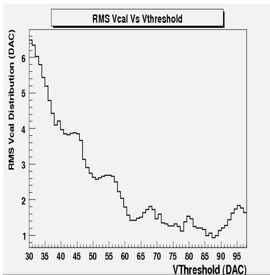
Figura 8-3: La figura muestra como el valor del RMS de las distribuciones de Vcal para los píxeles se hace más grande para valores de VThreshold bajos.
