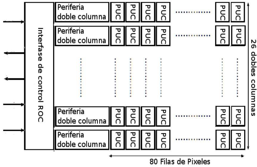
Figura 5-1: Diagrama de bloques del ROC [20]
