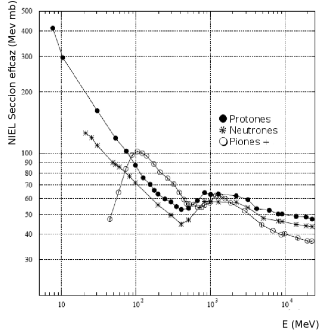
Figura 4-4: Sección eficaz para partículas normalizadas equivalentes al daño producido por neutrones con energía cinética de 1 MeV sobre silicio cristalino. [18].
