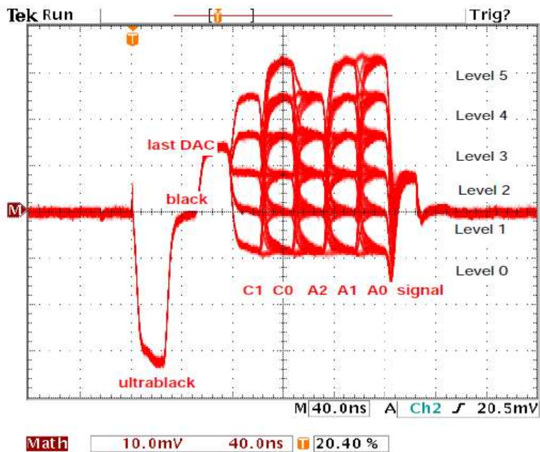
Figura 5-3: Señal analógica [20].
