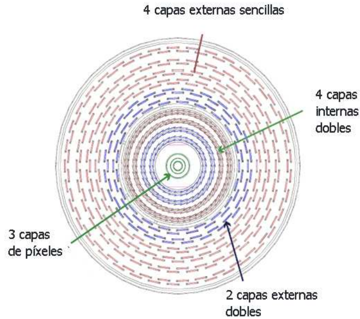
Figura 2-2: Capas del detector de trazas [1].
