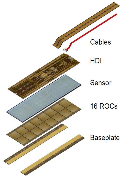
Figura 2-4: Piezas principales de un módulo del detector de píxeles [3].
