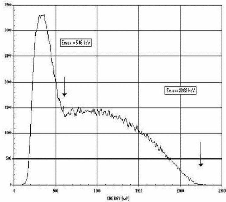
Figura 9-2: Espectro de partículas Beta Sr 90.
