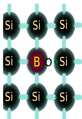
Figura 3-4: Modelo bidimensional del silicio tipo P.
