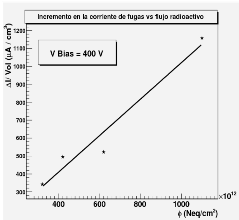
Figura 10-4: Corriente generada por unidad de volumen vs dosis para un voltaje inverso de 400 V.
