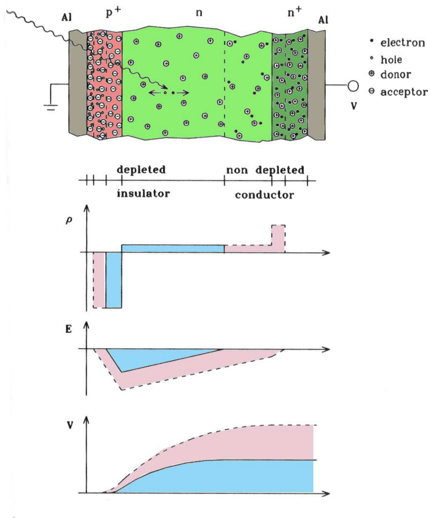
Figura 3-7: Modelo de las uniones en un píxel N en N^+ [6].
