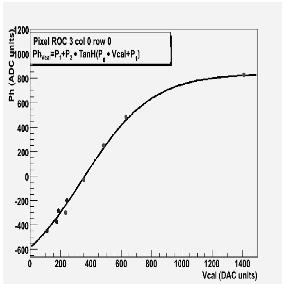
Figura 6-3: Ejemplo de ajuste para un píxel típico.
