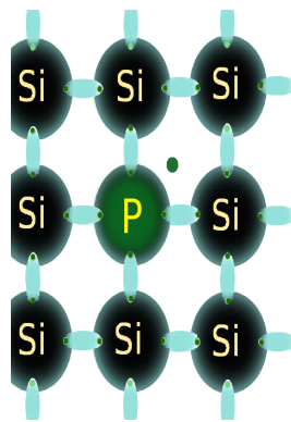
Figura 3-5: Modelo bidimensional del silicio tipo N.
