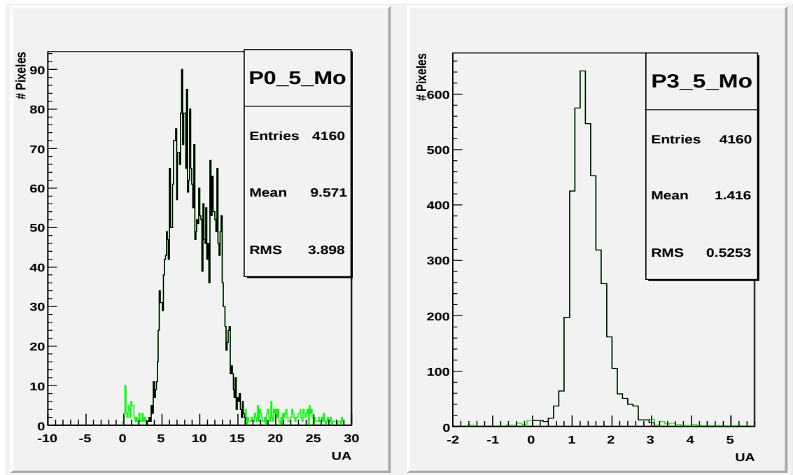
Figura 7-9: Distribuciones de los parámetros obtenidos al realizar el ajuste en el ROC 5. Las distribuciones en verde claro son las distribuciones de los parámetros sin descartar ningún píxel, las distribuciones en negro corresponden a los píxeles utilizados en el análisis.
