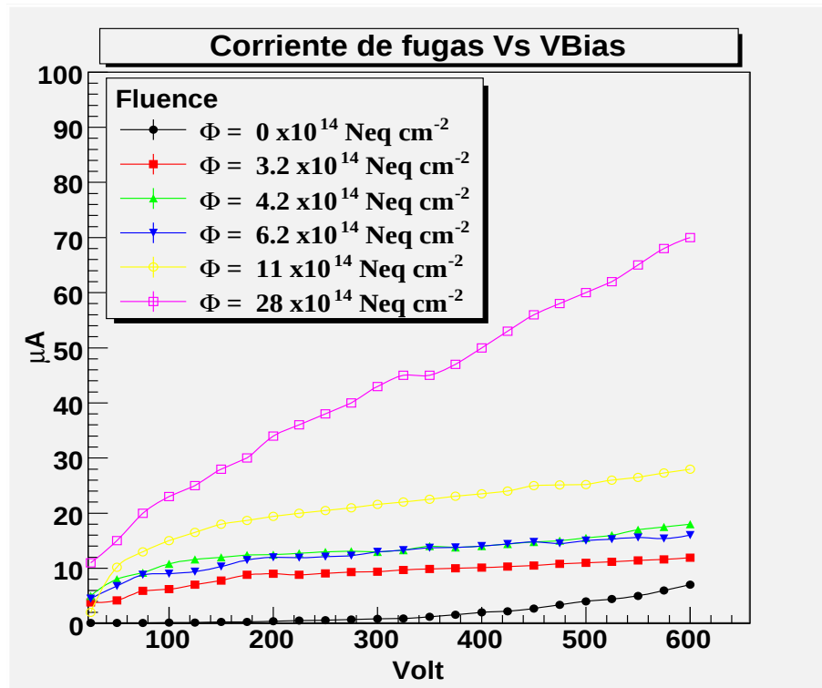
Figura 10–3: Corriente de fugas vs voltaje inverso para ROCs expuestos a diferentes dosis de radiación.
