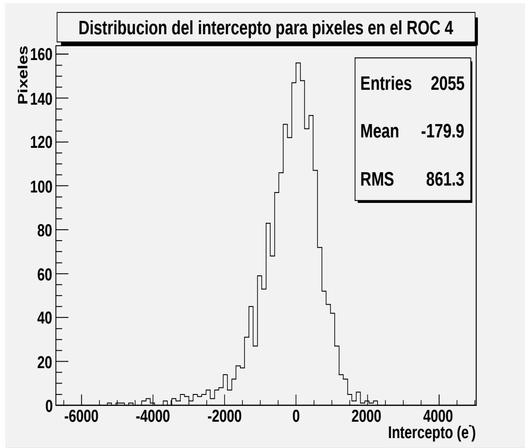
Figura 8-5: Distribución del intercepto para el ROC 4.
