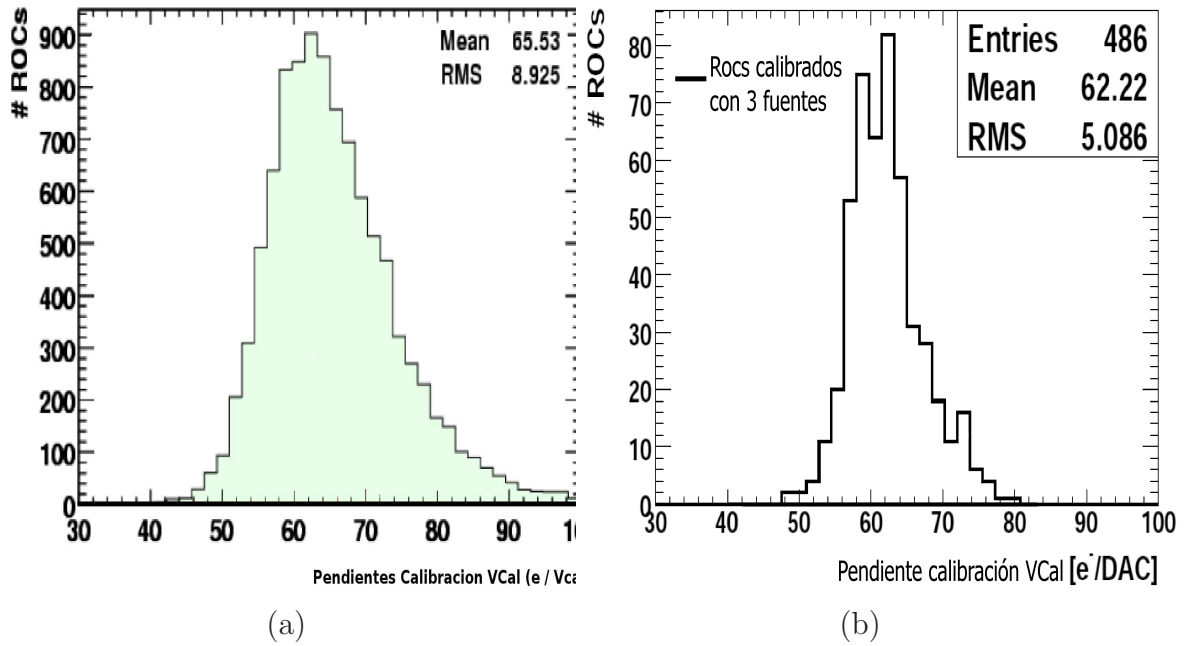
Figura 8-7: Distribución de pendientes calibración V_{Cal} . (a) 2 fuentes (b) 3 fuentes.
