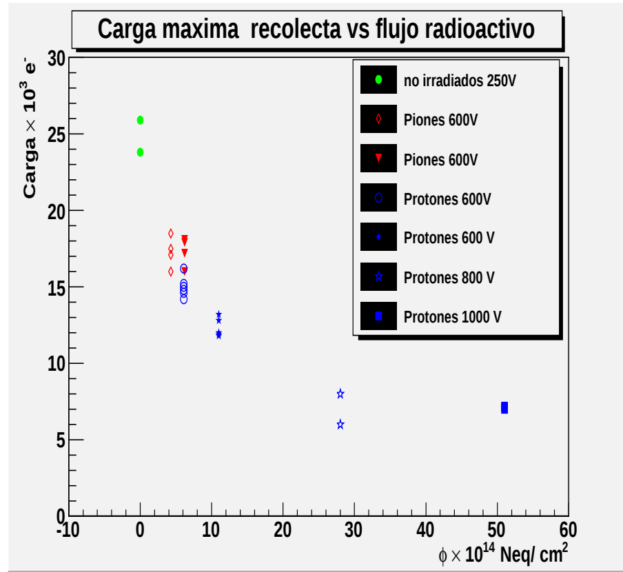
Figura 10-5: Máxima cantidad de carga medida en sensores sometidos a radiación.
