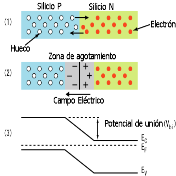
Figura 3-6: Modelo de la unión P-N [5].
