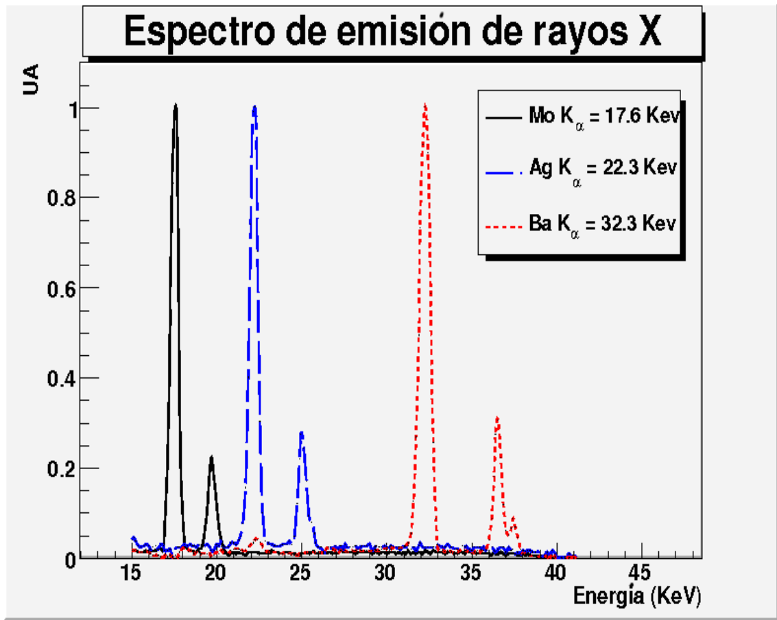
Figura 7-5: Espectro de emisión de los blancos de la fuente de X Am241 [24]
