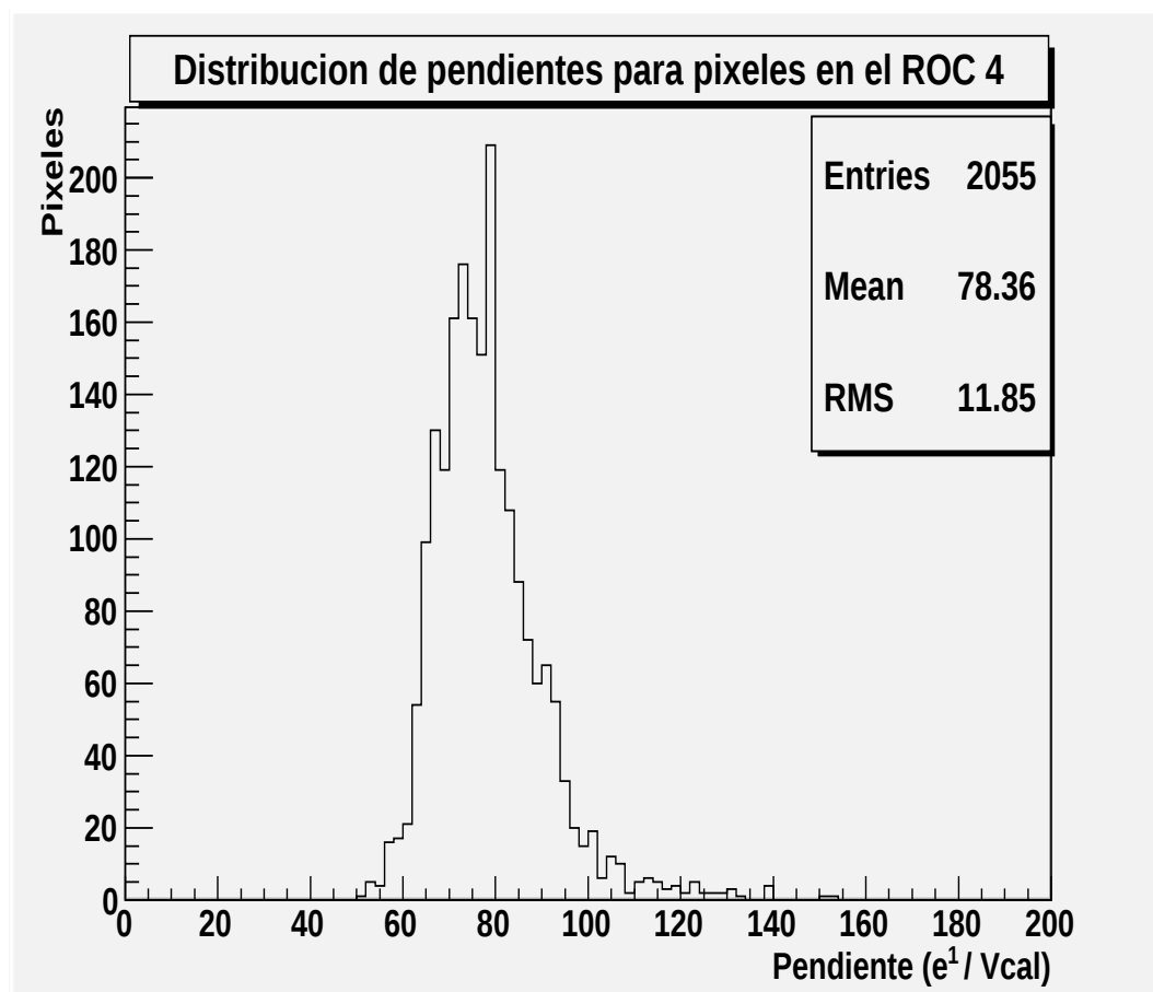
Figura 8-4: Distribución de las pendientes para el ROC 4.
