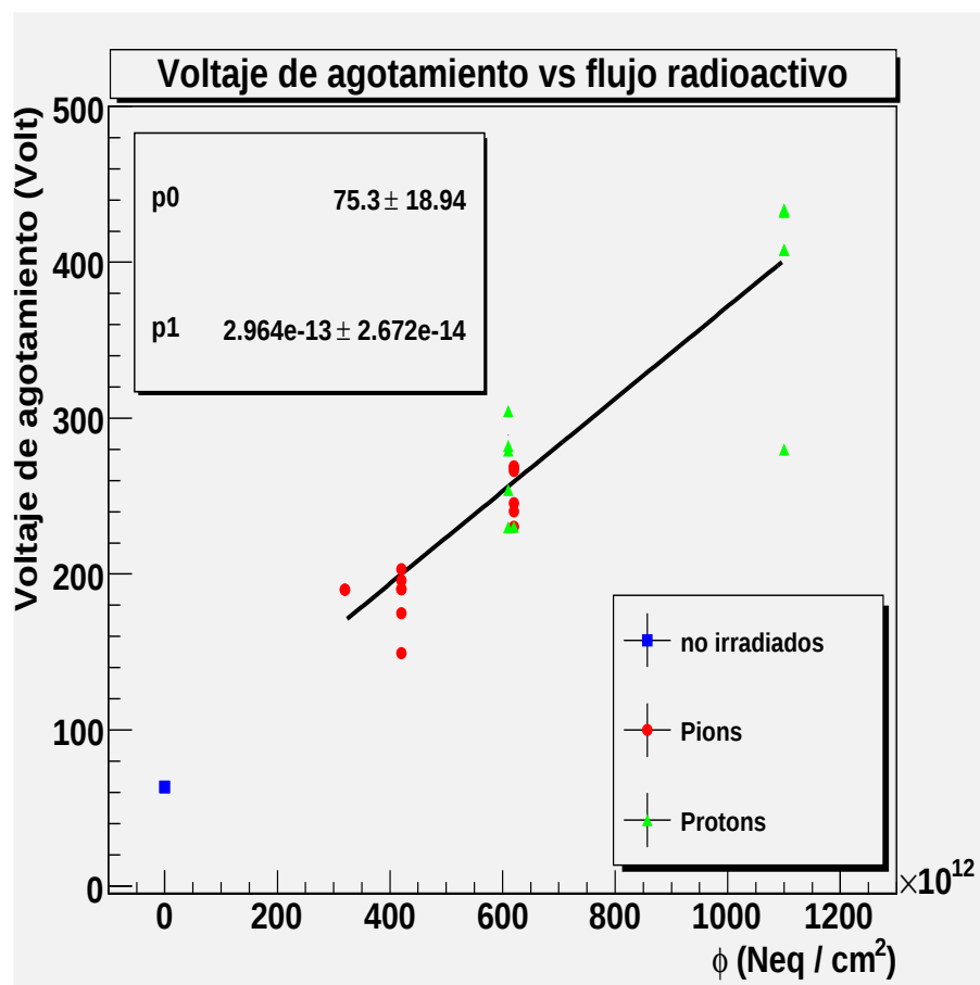
Figura 10-2: Voltaje de agotamiento contra flujo radioactivo.
