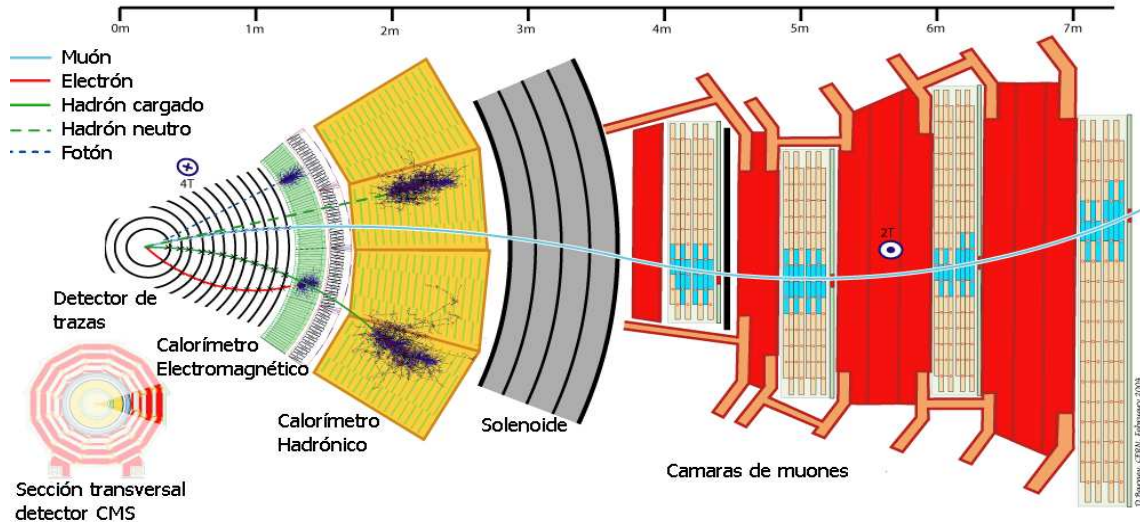
Figura 2-1: Configuración del detector CMS [1].
