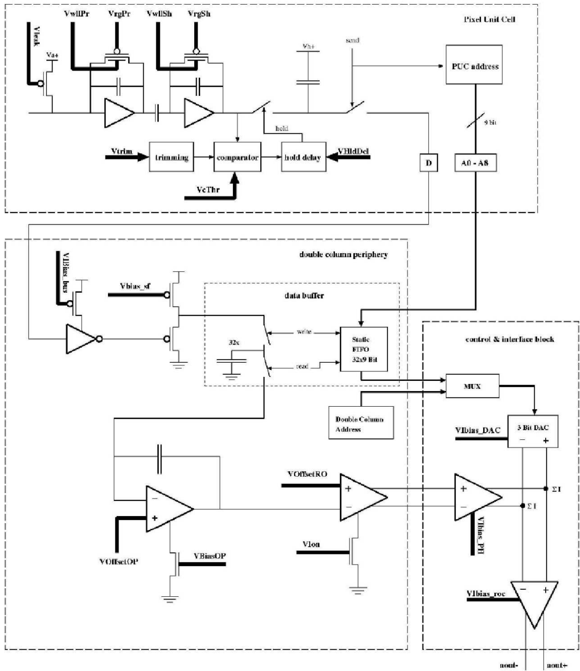
Figura 5-4: Diagrama de bloques PSI46. [20].
