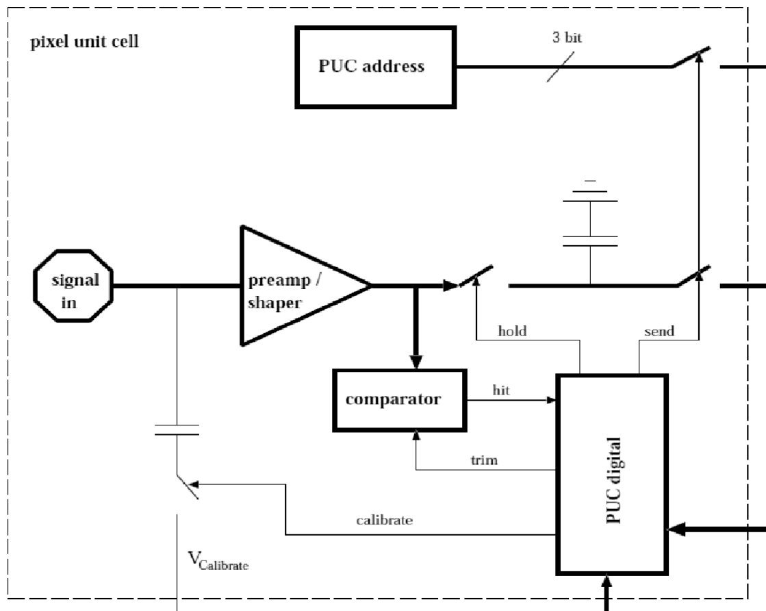
Figura 5-2: Esquema de la electrónica acoplada a cada píxel ( pixel unit cell ) [21].
