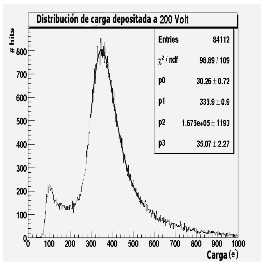
Figura 9-3: Distribución IEL con un voltaje inverso de 200V
