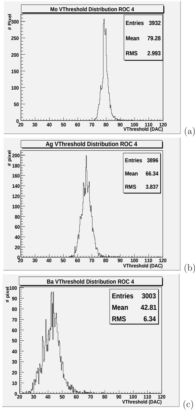
Figura 8-1: Distribuciones de VThreshold equivalente para el ROC 4, (a) Mo,(b) Ag y (c) Ba
