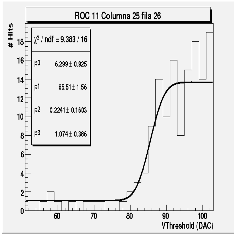
Figura 7-7: Ejemplo de ajuste para un píxel
