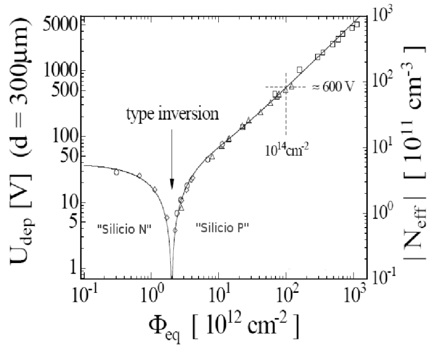
Figura 4-5: Concentración de portadores en función del flujo radioactivo (NIEL). [14].
