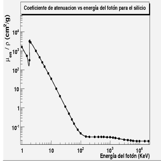
Figura 4-2: Coeficiente de atenuación para silicio ( Z=14 ). El eje horizontal muestra la energía del fotón incidente y el eje vertical la magnitud de coeficiente de atenuación. [14].
