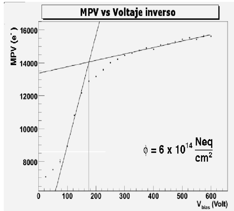
Figura 9–5: Método de intersección en una gráfica MPV vs voltaje inverso.
