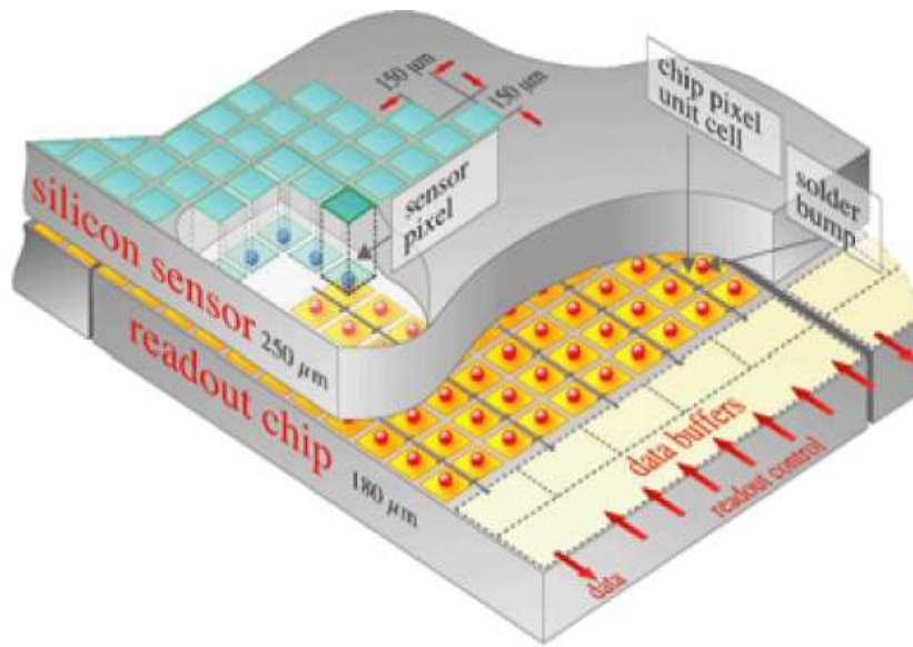
Figura 3-1: Detalle del sensor del detector de píxeles [4].
