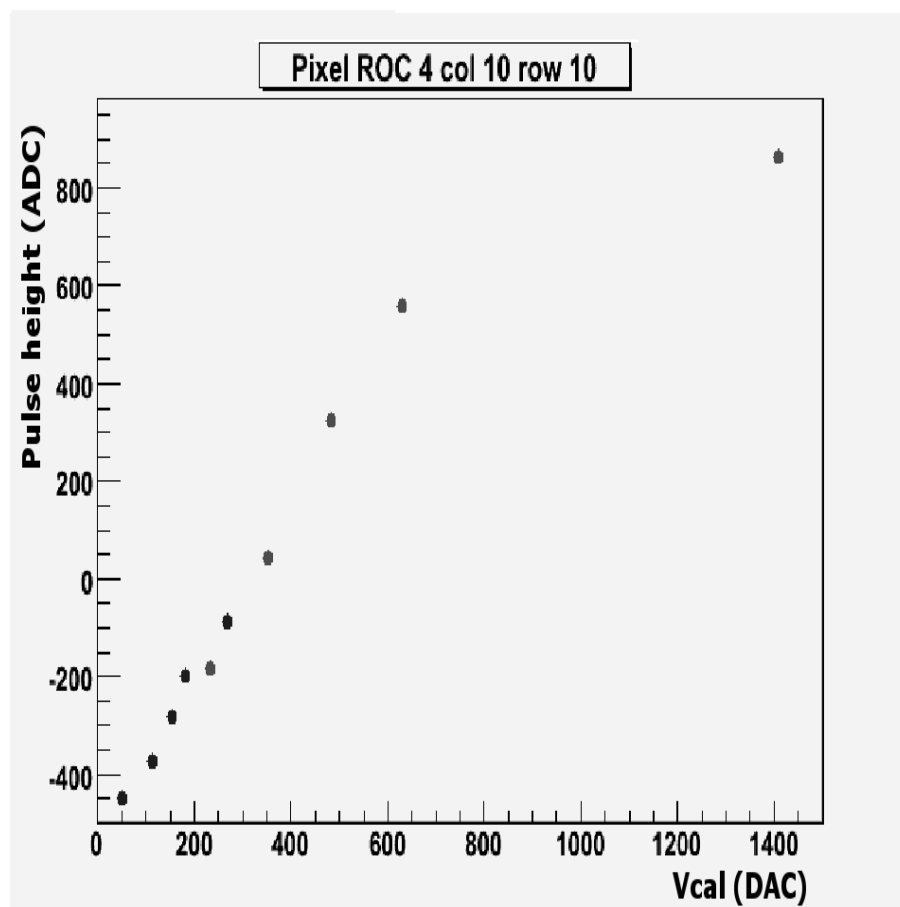
Figura 6-2: Ejemplo de medida para un píxel típico.
