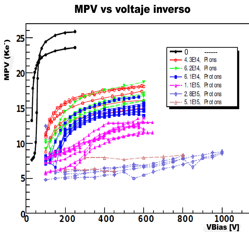
Figura 10-1: Gráfica MPV vs voltaje inverso para todo los sensores estudiados.
