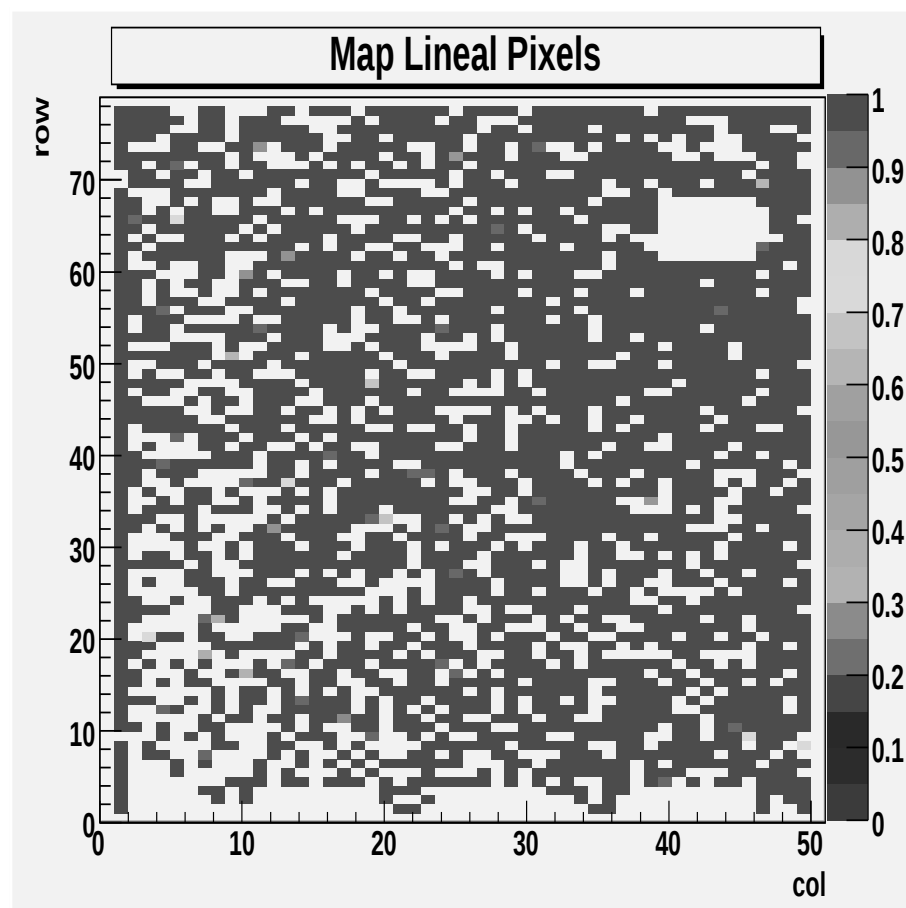
Figura 7-10: Mapa de píxeles que superan los criterios de calidad en el ROC 4.
