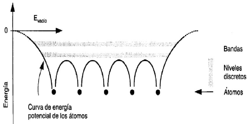
Figura 3–2: Modelo de bandas [5].
