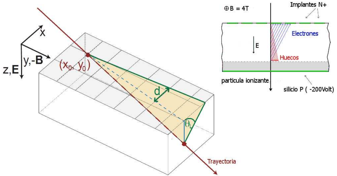
Figura 3-8: Trayectoria probable dentro de un segmento del detector de píxeles [7].
