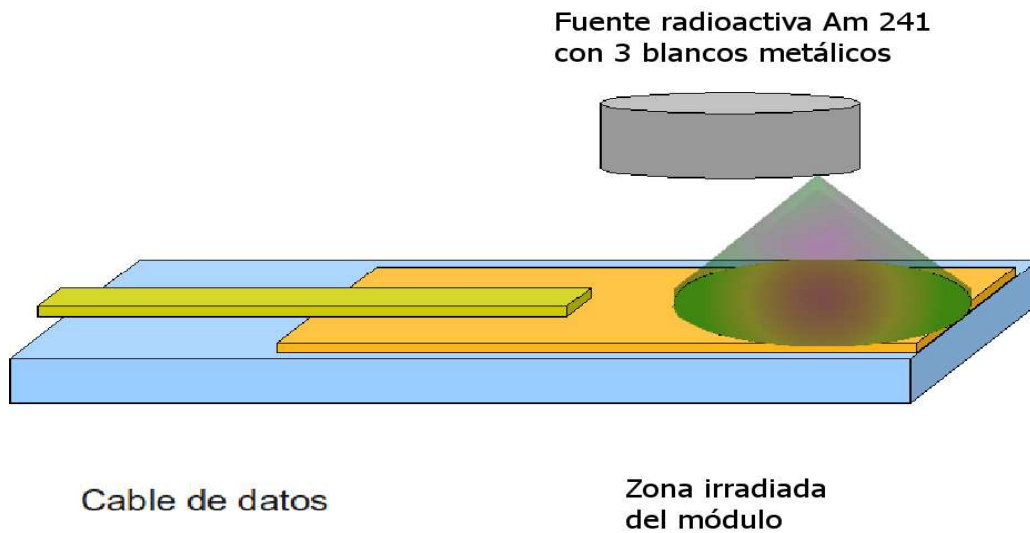
Figura 7-6: Configuración del experimento para la toma de datos
