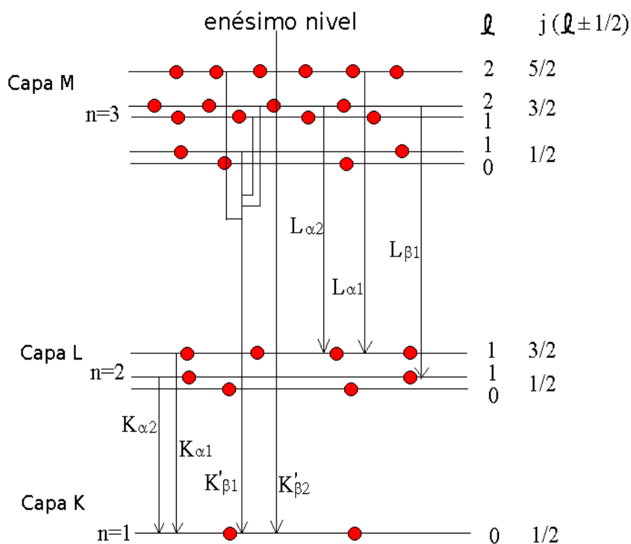
Figura 7-4: Diagrama de niveles de energía accesibles por los electrones en un átomo. Al incrementar n se incrementa la energía. La separación de niveles no está a escala [14].
