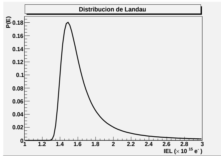
Figura 4-1: Distribución de Landau para 270\mu m de silicio. El eje horizontal muestra la cantidad de pares electrón-hueco generados por ionización y el eje vertical la magnitud de la función de probabilidad.
