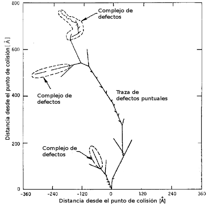
Figura 4-3: Simulación del efecto de un núcleo de silicio de energía cinética de 50 KeV después de ser impactado por un neutrón con energía cinética de 1 MeV. [16].
