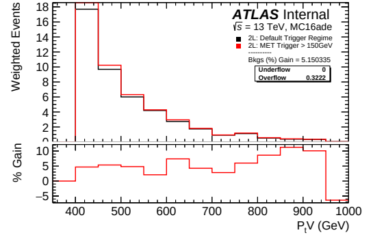
(d) Background yield increase: 5.15%, p_T^V \geq 400 \text{ GeV}
