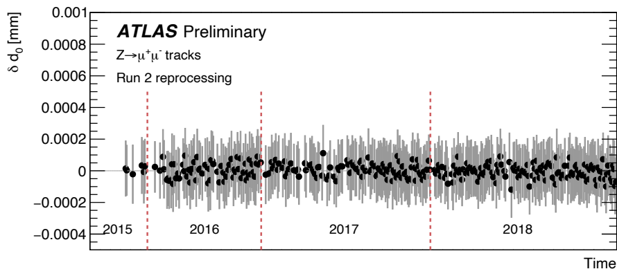
Figura R.6: Diferencia en el parámetro de impacto transversal entre muones positivos y negativos ( \delta d_0 ) en función del tiempo durante el Run 2 del LHC. Cada marcador representa la media del sesgo observado para una inyección del LHC, calculado a partir de mapas (\eta, \phi) divididos en 12 \times 12 sectores. Las barras de error indican la desviación estándar correspondiente.
