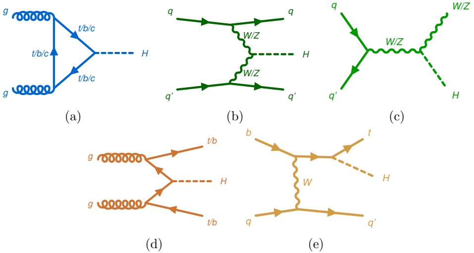
Figura R.2: Ejemplos de diagramas de Feynman a LO correspondientes a los principales modos de producción del bosón de Higgs en el LHC: fusión de (a) gluones o (b) bosones vectoriales, y producción asociada con (c) bosones vectoriales, (d) pares de quarks top o bottom, o (e) un único quark top.
