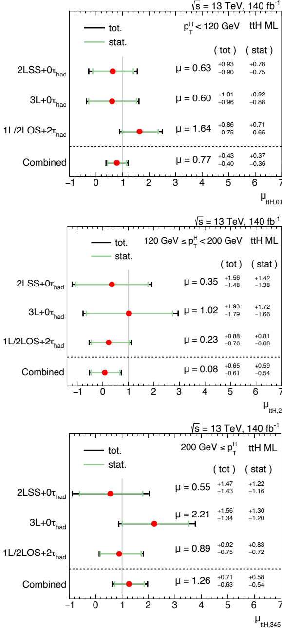
Figura R.16: Valores observados de los tres parámetros de interés y sus incertidumbres para los canales individuales relevantes ( 3\ell + 0\tau_{\text{had}} , 2\ell\text{SS} + 0\tau_{\text{had}} , 1\ell + 2\tau_{\text{had}} y 2\ell\text{OS} + 2\tau_{\text{had}} ) y de forma combinada. En orden descendente: \mu_{\text{t}\bar{\text{t}}\text{H},01} , \mu_{\text{t}\bar{\text{t}}\text{H},2} , y \mu_{\text{t}\bar{\text{t}}\text{H},345} , que corresponden a los intervalos p_T^H [\text{GeV}] \in [0, 120) , [120, 200) , y [200, \infty) , respectivamente. La predicción del ME corresponde a \mu_{\text{t}\bar{\text{t}}\text{H}} = 1 .
