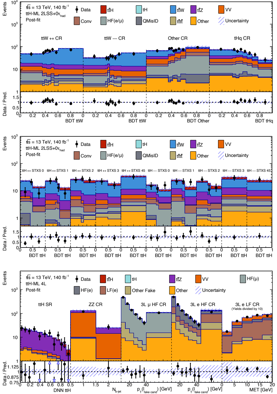
Figura R.13: Comparación entre los eventos observados y los predichos en todas las regiones para los canales 2\ell SS + 0\tau_{\text{had}} y 4\ell . La banda de incertidumbre incluye todas las incertidumbres y sus correlaciones.
