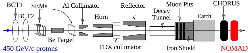
Рис. 3.3: Схематический вид основных элементов, служащих для создания нейтринного пучка.
