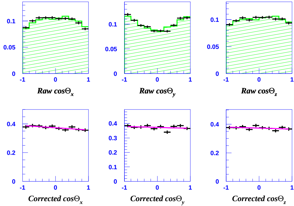
Рис. 6.6: Верхние рисунки: нескорректированные нормализованные распределения пионов по \cos \theta_i , образовавшиеся из распада K_S^0 в реконструированных событиях МК (гистограммы) и в реальных данных (точки с допустимыми интервалами ошибок). Нижние рисунки: те же самые распределения после коррекции на угловое разрешение детектора; поляризация определяется наклоном линии, проведенной через эти точки.
