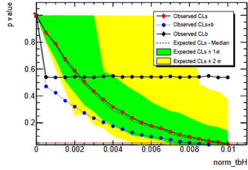
(d) P-value from Toy Model for a 2000 GeV signal.
