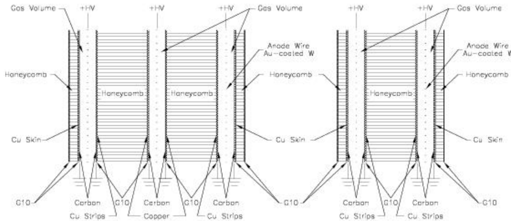
FIG. II.2.23 – Vue schématique en coupe d'un triplet (à gauche) et d'un doublet (à droite) de TGC. La largeur de l'espacement de gaz est représentée agrandie.
