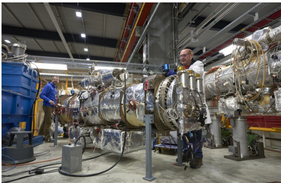
Le nouvel aimant de déflexion rapide prototype en cours de préparation sur le site de Prévessin. Il sera installé au point 8 pour améliorer les performances lors de l'injection des particules dans le LHC. (Image : Maximilien Brice/CERN)
