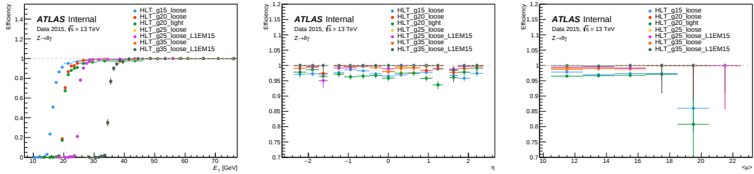
Figura 4.5: Eficiencias de los triggers de fotones para el año 2015 en función del E_T (izquierda), \eta (centro) y \langle\mu\rangle (derecha).
