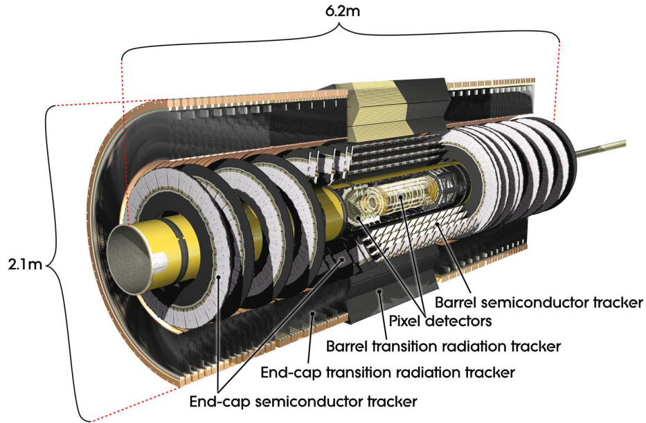
Figura 2.8: Esquema del detector interno de ATLAS, donde se señalan los diferentes módulos [64].
