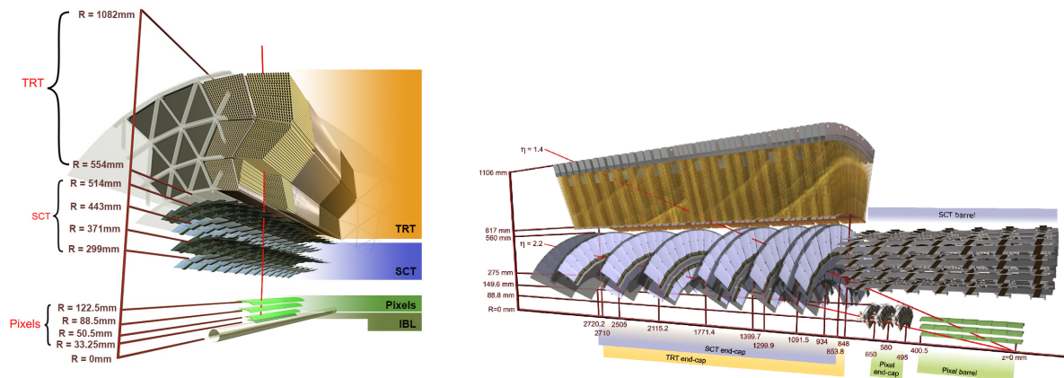
Figura 2.9: Vista lateral y frontal del detector interno de ATLAS junto con sus módulos [64, 65].
