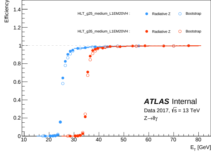
Figura 4.4: Comparación de las eficiencias utilizando el método Bootstrap y el método del bosón Z radiativo para dos triggers del 2017.
