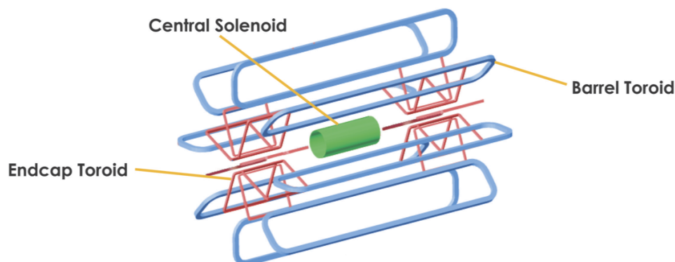
Figura 2.7: Sistema de imanes del detector ATLAS [63].
