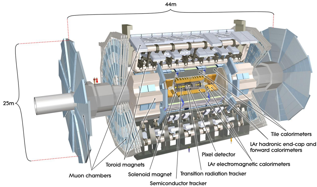
Figura 2.5: Esquema del detector ATLAS, indicando cada uno de los subdetectores que lo componen [60].
