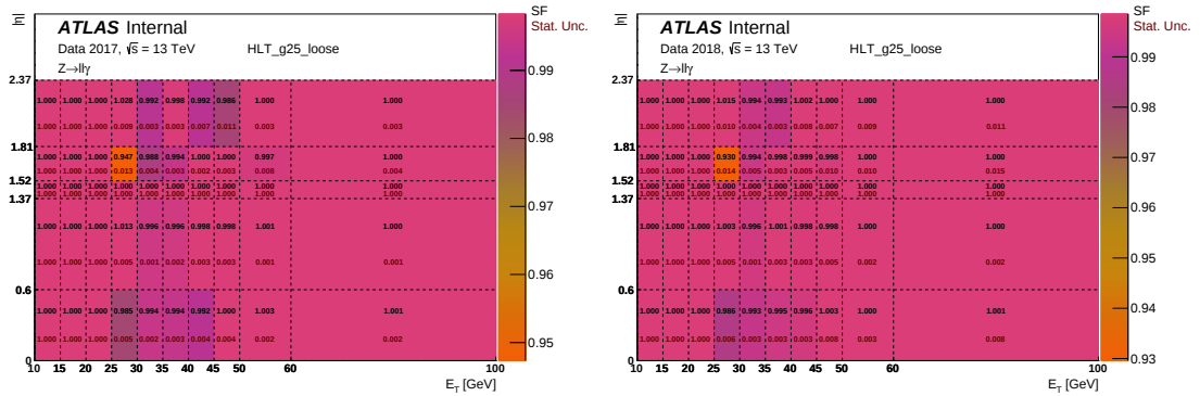
Figura 4.10: Scale Factors para el trigger HLT_g25_loose en función de E_T y \eta con un WP de aislamiento FixedCutTightCaloOnly , para el año 2017 (izquierda) y 2018 (derecha). En rojo las incertezas estadísticas.
