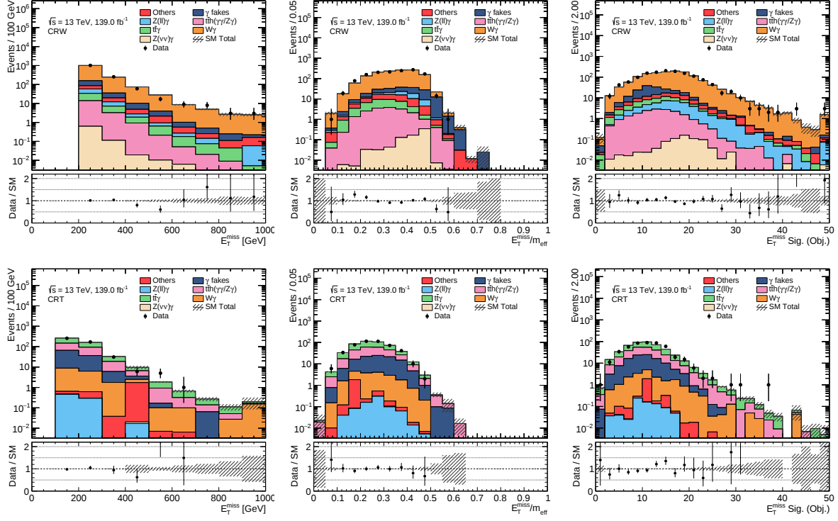
Figura 7.4: Distribuciones preliminares en la región de control CRW y CRT luego del ajuste de solo fondo, para el análisis de producción electrodébil. Las incertezas mostradas son sólo estadísticas.
