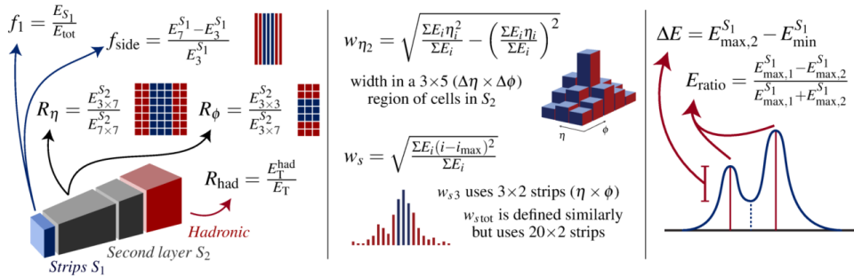
Figura 3.5: Esquema de algunas de las variables empleadas para la identificación de fotones. E_C^{S_N} representa la energía en la capa N del ECAL en un cluster C [101].
