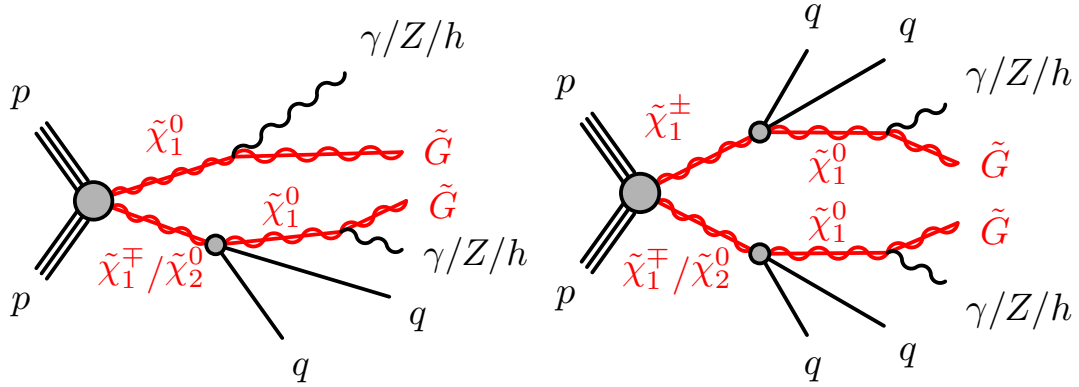
Figura 7.1: Diagramas de producción de gauginos con estado final de fotones, bosones Z, Higgs y gravitinos
