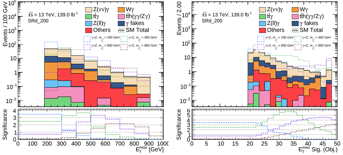
Figura 7.7: Distribuciones preliminares de E_T^{\text{miss}} y \mathcal{S} en la región de señal SRd_200 luego del ajuste de solo fondo para el análisis de producción electrodébil, donde se incluyen algunas distribuciones de señal. Las incertezas mostradas son sólo estadísticas.
