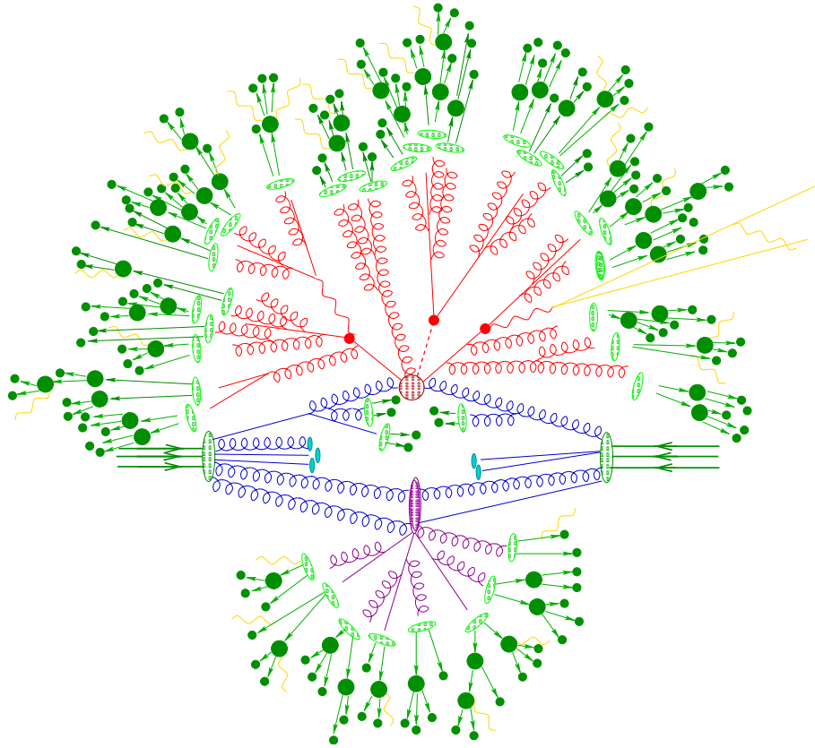
Figura 2.15: Esquema de una colisión protón-protón simulada por un generador de eventos de Monte Carlo. La región roja en el centro representa la dispersión dura, rodeada por una estructura que representa la radiación de QCD simulada por los PS. La parte violeta indica un evento subyacente de dispersión dura. Las transiciones de partones a hadrones están representadas por las partes verdes claras, mientras que las partes verdes oscuras indican el decaimiento de los hadrones. Finalmente, las líneas amarillas señalan la radiación de fotones [83].
