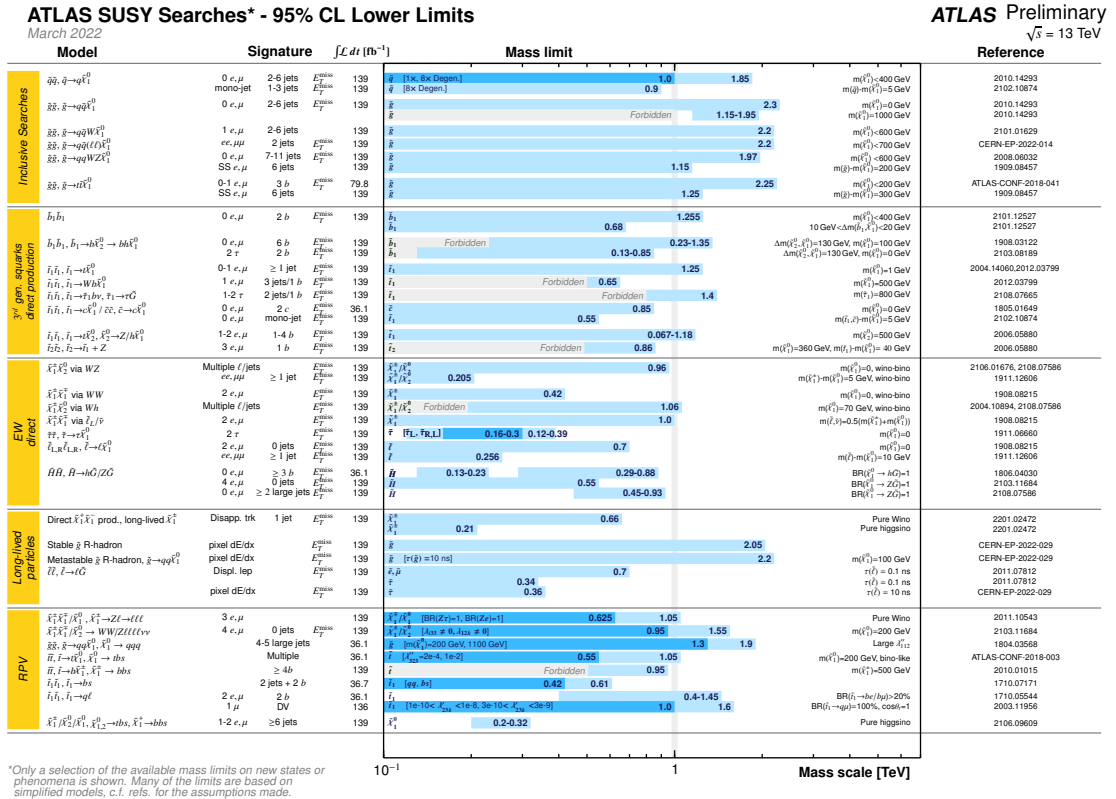
Figura 1.10: Estado actual de los límites obtenidos para las masas de las partículas supersimétricas, considerando diferentes tipos de producción y canales de decaimiento [47].
