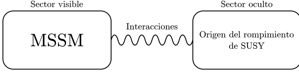
Figura 1.5: Estructura esquemática de la ruptura de supersimetría.
