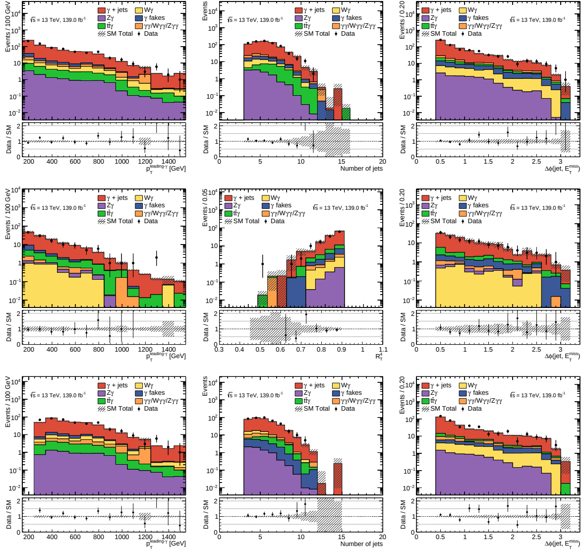
Figura 6.12: Distribuciones de algunas variables significativas en las regiones de validación VRQ (arriba), VRM1H (medio) y VRM1L (abajo) luego del ajuste de solo fondo. Las incertezas mostradas son sólo estadísticas.
