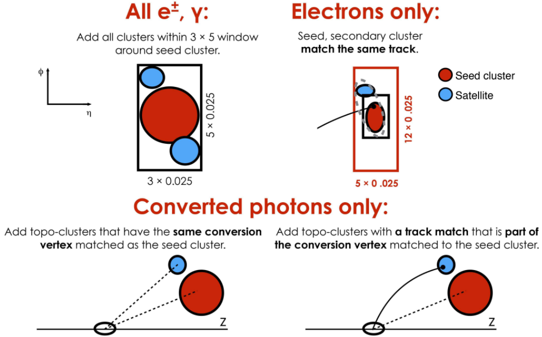
Figura 3.3: Esquema de formación de superclusters de para electrones y fotones. En rojo se muestran los topo-clusters semilla, y en celeste los satélites [94].
