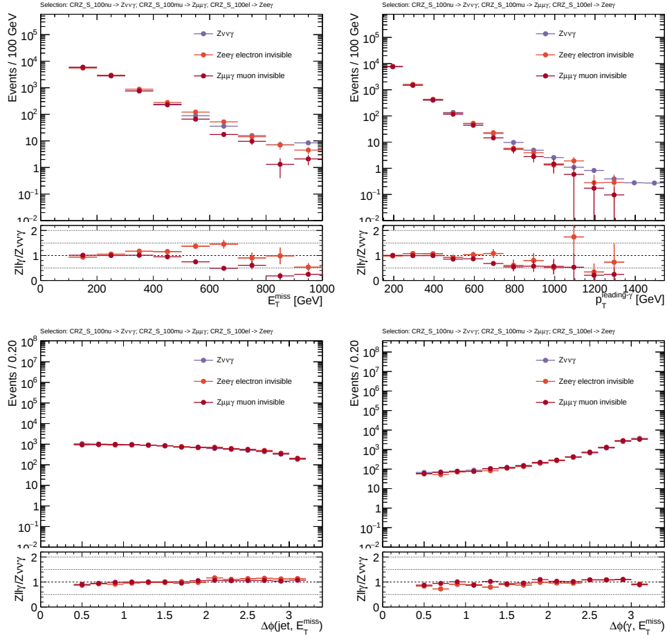
Figura 7.3: Comparación de E_T^{\text{miss}} en el fondo de Z(\nu\nu)\gamma y la reconstruida para los fondos de Z(ee)\gamma y Z(\mu\mu)\gamma .
