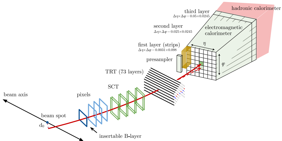
Figura 3.2: Esquema del paso de un electrón a través del detector. La línea roja muestra el trayecto hipotético del electrón, el cual atraviesa primero el detector interno, para luego llegar al calorímetro. La línea roja punteada representa el trayecto de un fotón producido por la interacción del electrón con el material [69].
