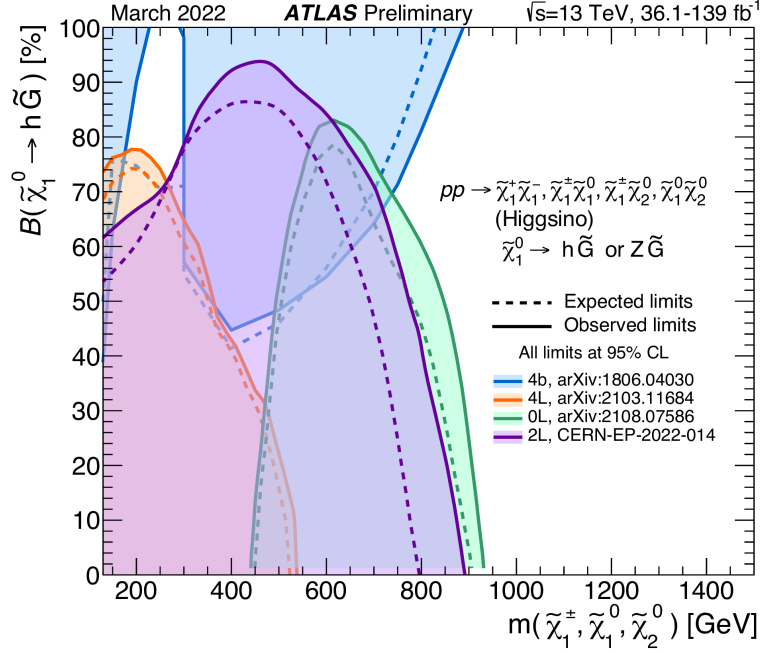
Figura 7.9: Últimos límites impuestos a la masa de los gauginos para modelos GGM en función de su fracción de decaimiento a Higgs, combinando distintos resultados observados por la colaboración ATLAS [189].
