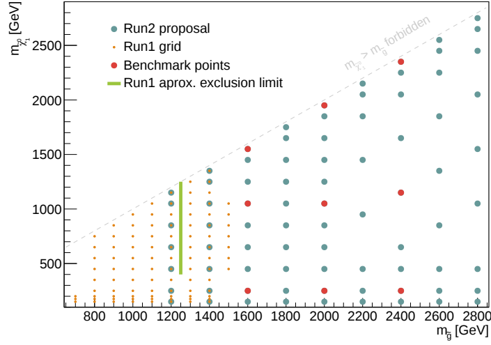
Figura 6.5: Arreglo de muestras de señal generados en función de la masa del \tilde{\chi}_1^0 y \tilde{g} (celeste). La densidad del mismo disminuye al aumentar m_{\tilde{g}} debido a que la sensibilidad del análisis se estimó ser menor a los 2 TeV. En rojo se muestran los puntos empleados para realizar pruebas preliminares de sensibilidad para el presente análisis. En naranja los puntos de señal simulados para un análisis equivalente realizado durante el Run 1, que excluye las masas marcadas por la línea verde.
