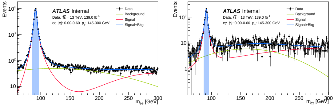
Figura 6.8: Distribución de la masa invariante para los pares ee (izquierda) and e\gamma (derecha) con |\eta| \in [0 - 0.6] , junto con las funciones ajustadas de señal (rojo) y fondo (verde). La región celeste representa la ventana de integración empleada para calcular los FFs. A alto p_T , una Gaussiana adicional es incluida para tener en cuenta el sesgo al aplicar un corte en dicha variable, que resulta despreciable su contribución en el número de eventos cerca del pico del Z.
