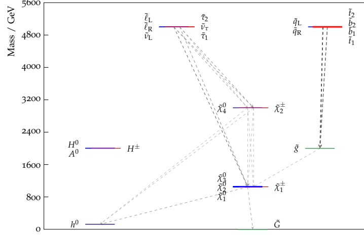
Figura 6.3: Espectro de masas de las partículas supersimétricas para el punto de señal con (M_3, \mu) = (2000 \text{ GeV}, -1050 \text{ GeV}) . En gris se muestran algunos de los posibles decaimientos de dichas partículas.
