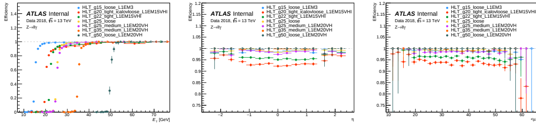
Figura 4.8: Eficiencias de los triggers de fotones para el año 2018 en función del E_T (izquierda), \eta (centro) y \langle\mu\rangle (derecha).
