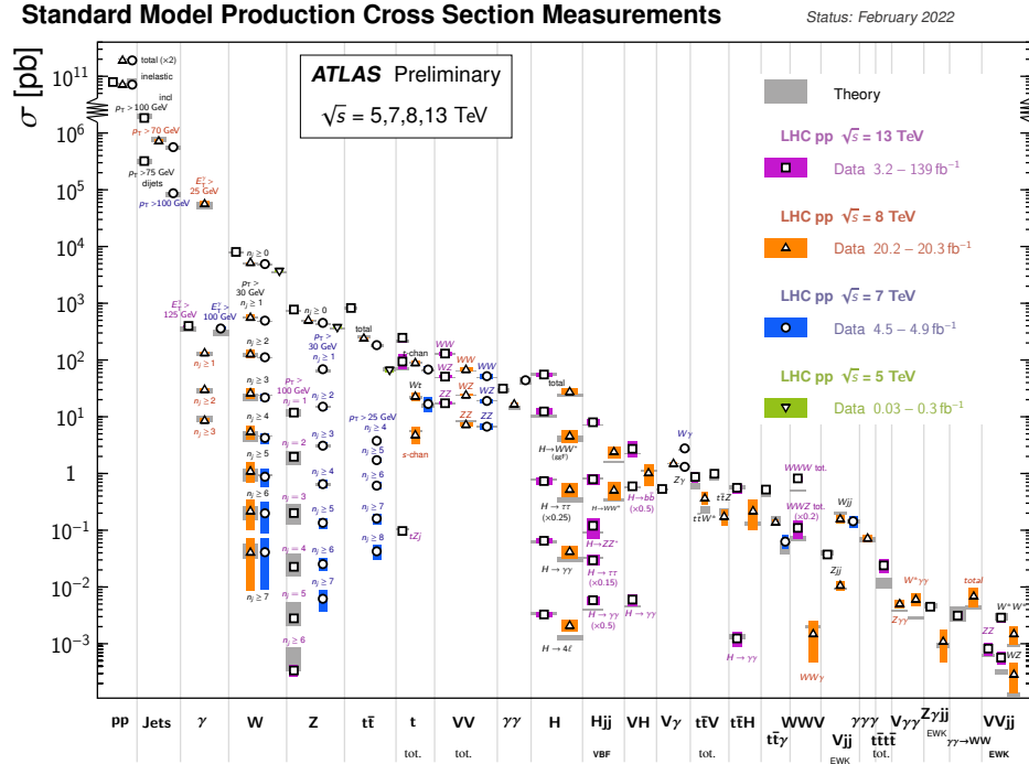
Figura 1.3: Resumen de las distintas medidas de sección eficaz de algunos procesos del SM, comparadas con sus valores teóricos esperados [34].
