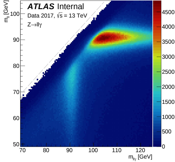
Figura 4.3: Masa invariante de dos leptones en función de la masa invariante de ambos leptones junto con un fotón. Las regiones con mayor concentración de eventos representan el decaimiento de un bosón Z a leptones o de forma radiativa.
