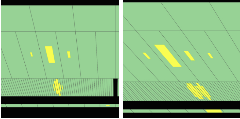
Figura 3.4: Depósitos de energía característicos de un fotón aislado (izquierda) y un \pi^0 (derecha). Se puede observar que la granularidad de la primera capa del ECAL permite discriminar dichos procesos [108].
