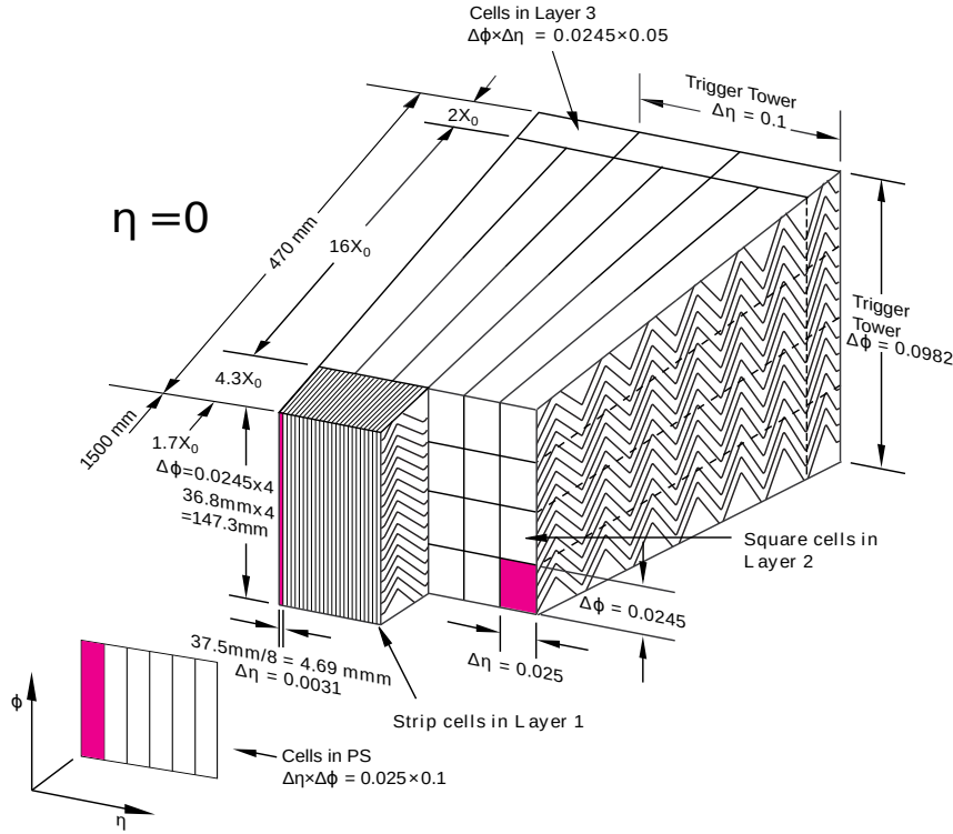
Figura 2.12: Segmento del ECAL del detector ATLAS en la región con \eta = 0 [69].
