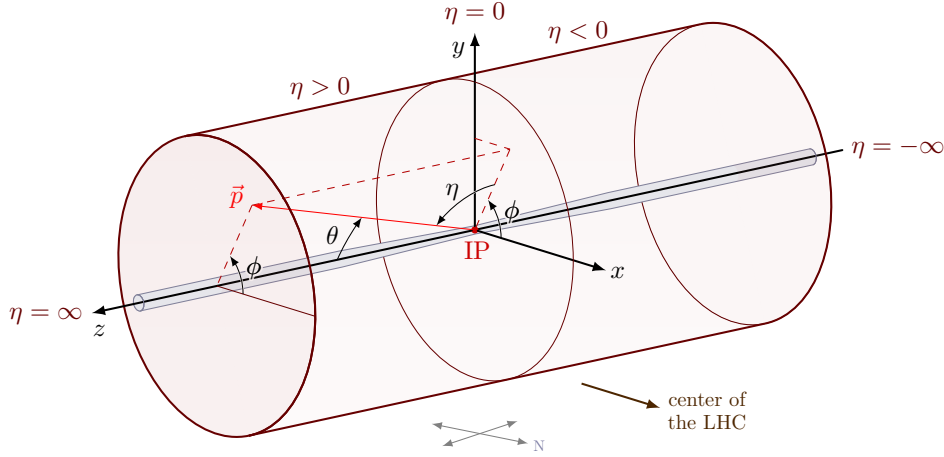
Figura 2.6: Diagrama del sistema de coordenadas del detector ATLAS [61].
