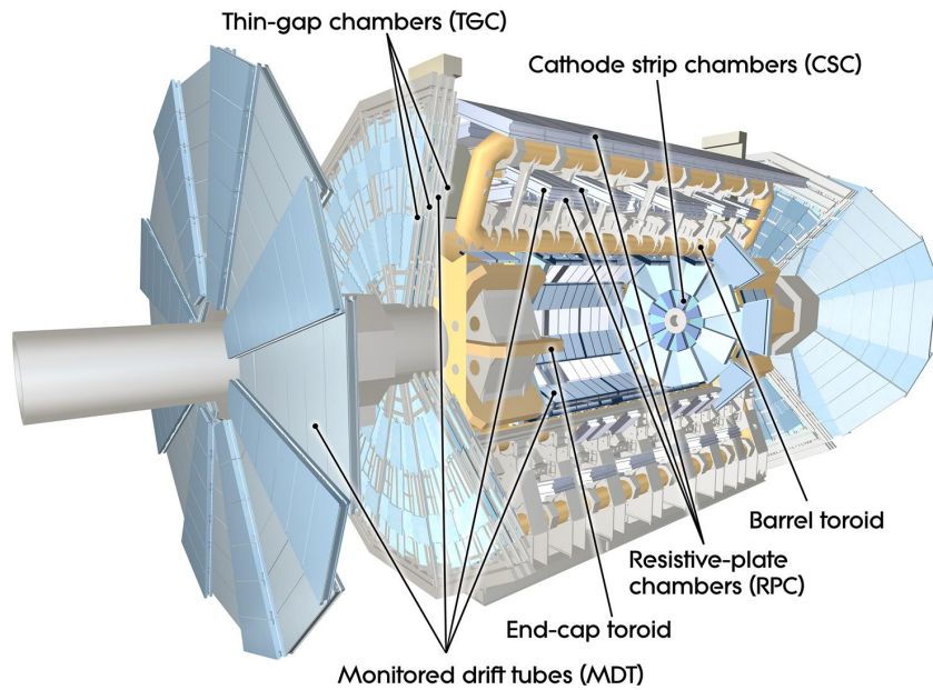
Figura 2.13: Espetrómetro de muones junto con el sistema de imanes toroidales (amarillo) del detector ATLAS [70].
