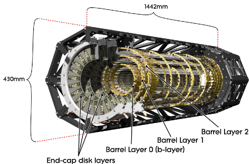
Figura 2.10: Esquema del detector de píxeles de ATLAS [67].
