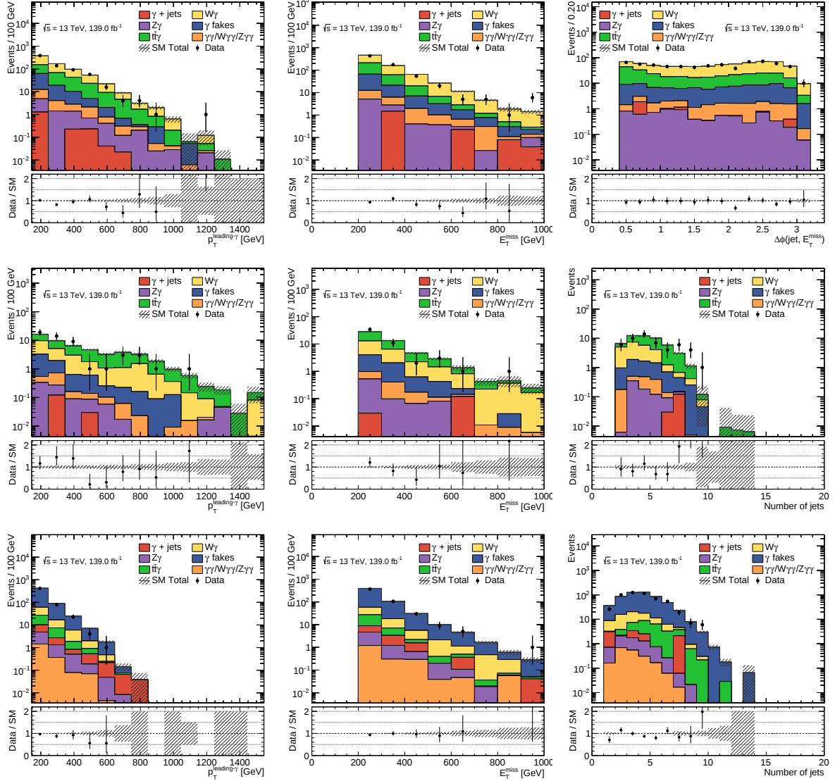
Figura 6.13: Distribuciones de algunas variables significativas en las regiones de validación VRL3 (arriba), VRL4 (medio) y VRE (abajo) luego del ajuste de solo fondo. Las incertezas mostradas son sólo estadísticas.
