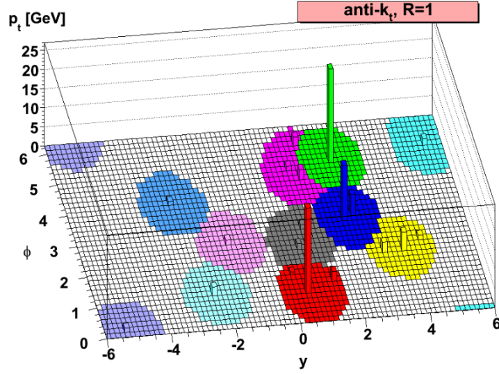
Figura 3.7: Esquema de agrupamiento de topo-clusters realizado por el algoritmo anti-k_t [116].
