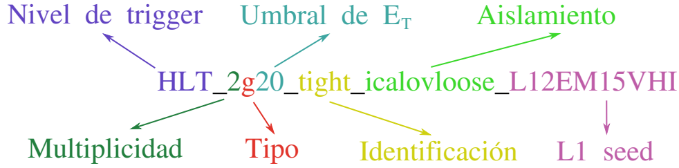
Figura 4.2: Convención para la nomenclatura de los triggers en ATLAS.
