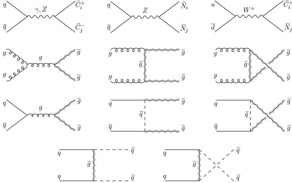
Figura 1.8: Algunos ejemplos de diagramas de Feynman de producción de partículas supersimétricas en colisionadores de hadrones. Las tres de arriba representan la producción electrodébil de gauginos, mientras que el resto la producción fuerte de gluinos y squarks.
