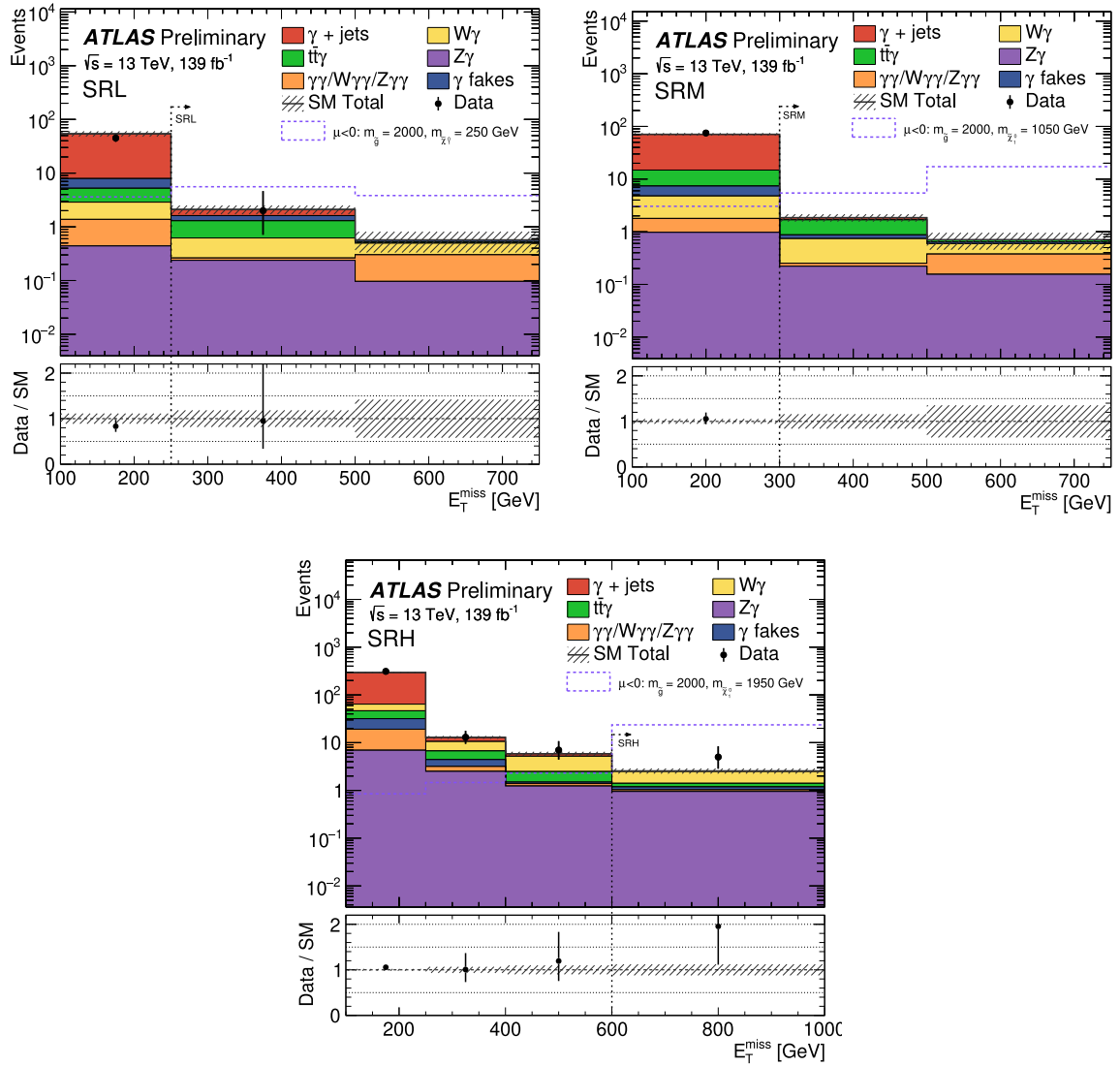
Figura 6.15: Distribución de E_T^{\text{miss}} para los datos observados y la estimación de los fondos, en las regiones de señal SRL (izquierda), SRM (derecha) y SRH (abajo), omitiendo el corte en esa misma variable (N-1). Se incluye además la distribución del punto de señal más significativo para cada región.
