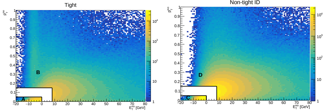
Figura 6.6: Distribución de datos en las variables de aislamiento para las regiones A, B, C y D.
