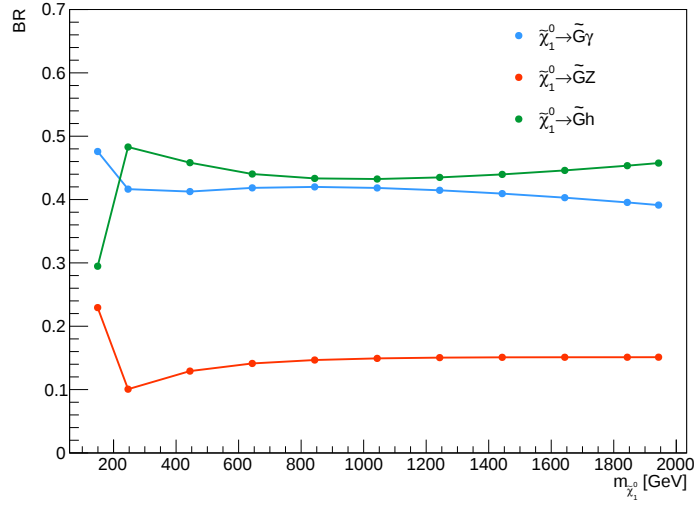
Figura 6.2: Fracción de decaimiento (BR) del \tilde{\chi}_1^0 en función de la masa del mismo.
