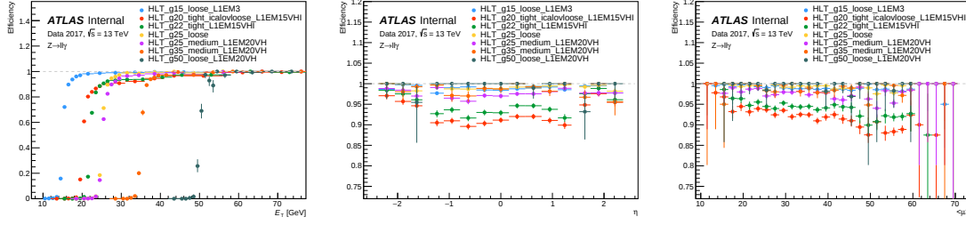
Figura 4.7: Eficiencias de los triggers de fotones para el año 2017 en función del E_T (izquierda), \eta (centro) y \langle\mu\rangle (derecha).
