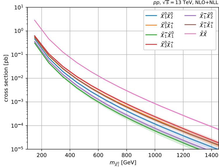
Figura 7.2: Sección eficaz de la producción de gauginos en función de la masa de \tilde{\chi}_1^0 . En rosa la sección eficaz total considerando todos los procesos.
