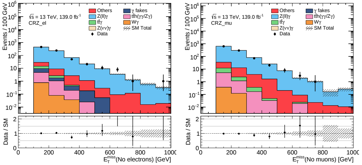
Figura 7.5: Distribuciones preliminares de E_T^{\text{miss}} en las regiones de control CRZ_el y CRZ_mu luego del ajuste de solo fondo, para el análisis de producción electrodébil. En el cálculo de dicha variable se remueven los correspondientes leptones. Las incertezas mostradas son sólo estadísticas.
