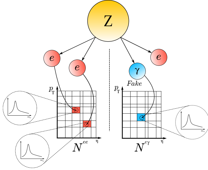
Figura 6.7: Esquema de reconstrucción de las distintas distribuciones de masa invariante utilizadas en el método. La clasificación en p_T de la imagen proviene de un método similar anterior, y actualmente solo se emplea una clasificación en |\eta| . Tanto las distribuciones de pares con fotón leading como de los pares con fotón sub-leading son almacenadas, pero no se hace explícito en la imagen.
