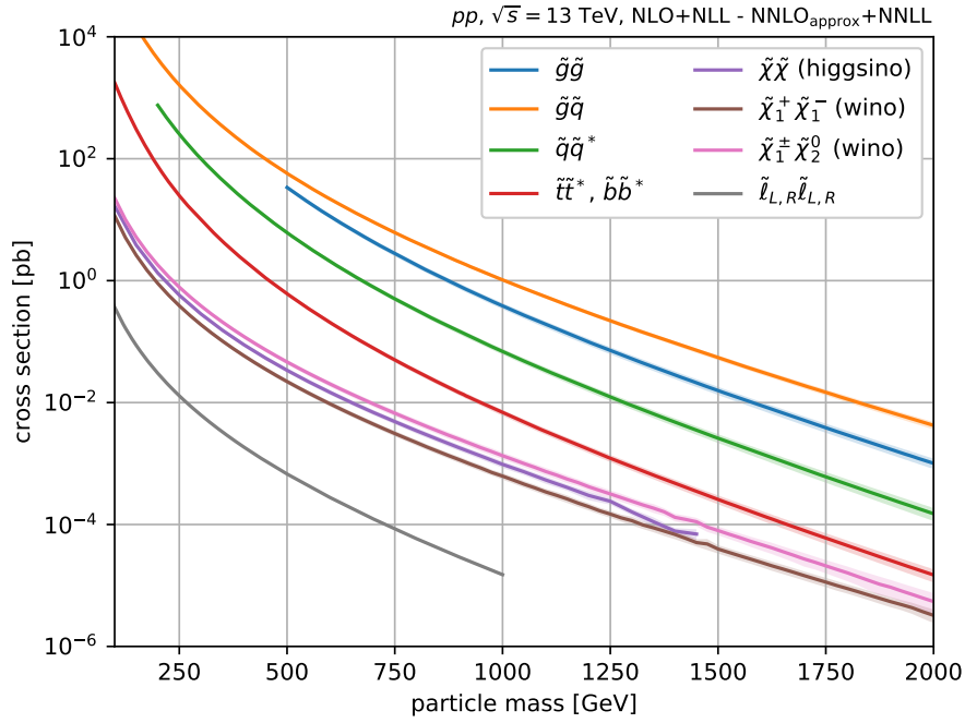
Figura 1.9: Sección eficaz de producción de partículas supersimétricas en colisiones pp [46].
