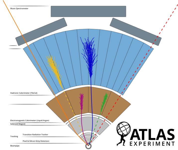
Figura 3.1: Esquema de los distintos tipos de señal que pueden dejar las partículas en el detector ATLAS. A grandes rasgos, los electrones dejan su depósito en el ECAL y una traza curvada en el ID, a diferencia de los fotones que no dejan traza. De la misma forma, los protones dejan su depósito en el HCAL y una traza curvada en el ID, mientras que los neutrones no dejan traza. Los muones escapan al detector pero dejan traza en el ID y el MS. Los neutrinos escapan del detector sin dejar ningún tipo de señal [93].
