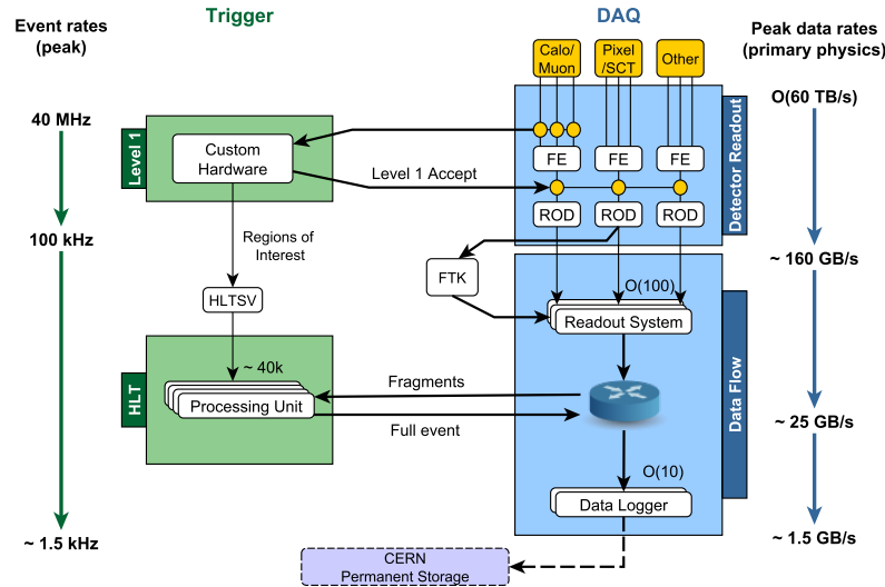
Figura 2.14: Esquema del sistema de trigger y el sistema de adquisición de datos de ATLAS [72].
