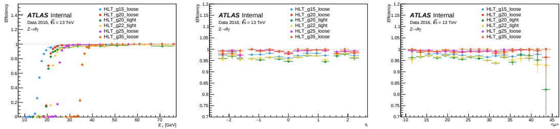
Figura 4.6: Eficiencias de los triggers de fotones para el año 2016 en función del E_T (izquierda), \eta (centro) y \langle\mu\rangle (derecha).
