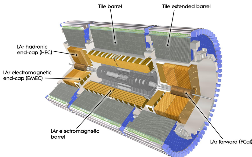
Figura 2.11: Esquema de los calorímetros del detector ATLAS [68].
