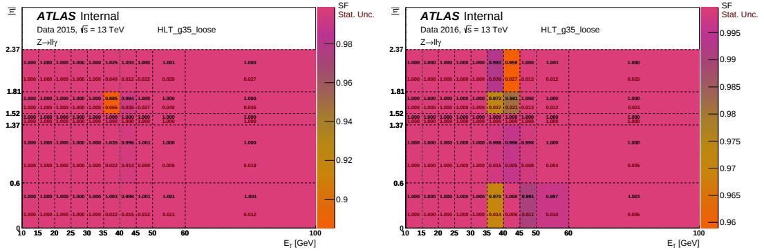
Figura 4.9: Scale Factors para el trigger HLT_g35_loose en función de E_T y \eta con un WP de aislamiento FixedCutTightCaloOnly , para el año 2015 (izquierda) y 2016 (derecha). En rojo las incertezas estadísticas.
