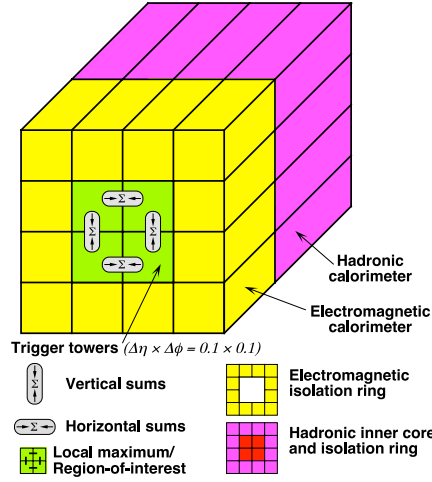
Figura 4.1: Esquema de torre de trigger empleada por los algoritmos del L1 [71].
