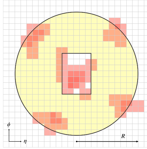
Figura 3.6: Esquema del cono utilizado para el cálculo de la variable de aislamiento calorimétrico.
