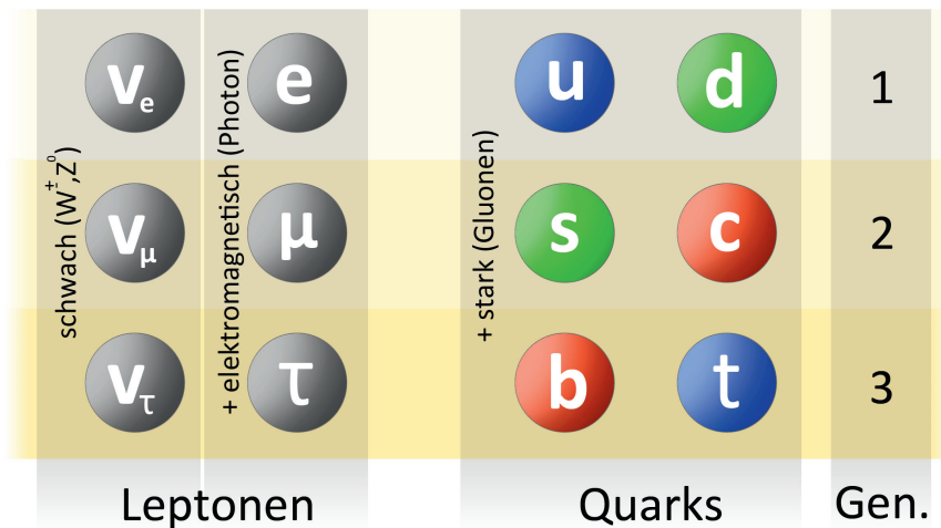
Abb. 1 Die Elementarteilchen des Standardmodells: Fermionen werden als Kugeln dargestellt. Vektorbosonen stehen in Klammern hinter den jeweiligen Kräften. Alle Fermionen, die rechts von einer Kraft (schwach, elektromagnetisch, stark) stehen, nehmen an dieser teil. So nimmt das Topquark „t“ zum Beispiel gleichzeitig an der schwachen, elektromagnetischen und starken Wechselwirkung teil.
