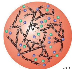
Abb. 12 Quark-Gluon-Wolke. Quelle: www.desy.de
