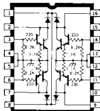
ULN 2064A
