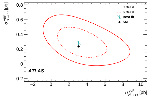
Figura R.3: Contorns de probabilitat per a la suma de tots els canals al pla (\sigma_{H \rightarrow \tau\tau}^{VBF}, \sigma_{H \rightarrow \tau\tau}^{ggF}) . La línia discontinua i la línia sòlida són el 68% i el 95% de nivell de confiança, respectivament, per a un bosó de Higgs amb una massa de m_H = 125 GeV. La predicció del model estàndard s'indica com a símbol '+', mentre que el millor valor de l'ajust a les dades és el símbol '*'
