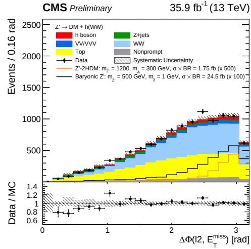
(d) \Delta\phi(E_T^{miss}, \ell_2) .
