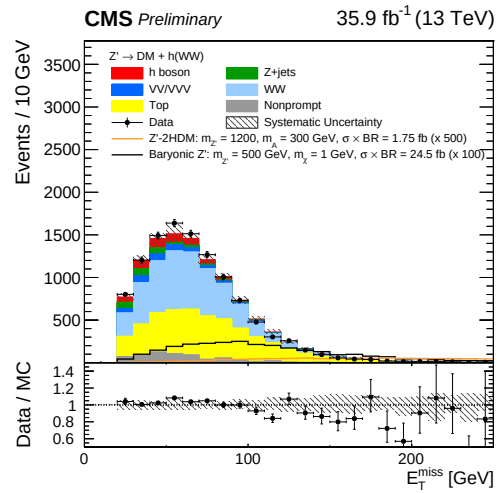
(f) P.F.Type I E_T^{miss} .
