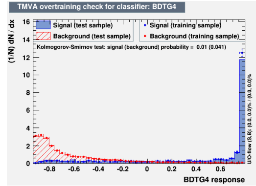
(d) nodeSize = 1.5%.
