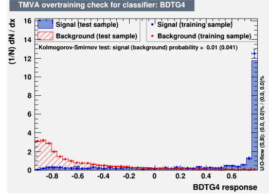
(d) baggingFraction = 0.5.
