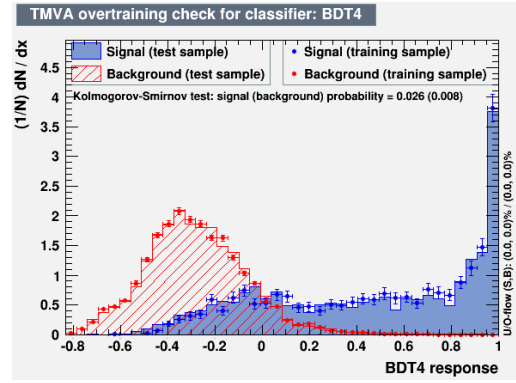
(d) adaBoostBeta = 0.1.
