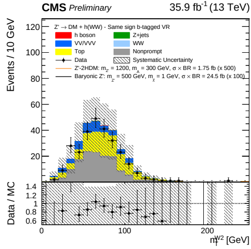
(b) m_T^{W2} .
