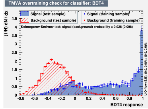
(d) nTrees = 500 .
