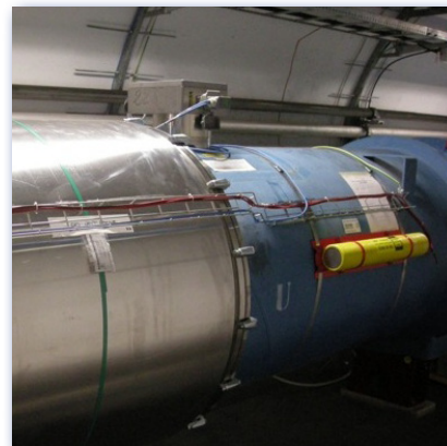
Un échantillon de matériaux organiques est fixé au tube du LHC (le sac blanc collé sur la ligne verte), pour des mesures ultérieures des doses de radiation.
