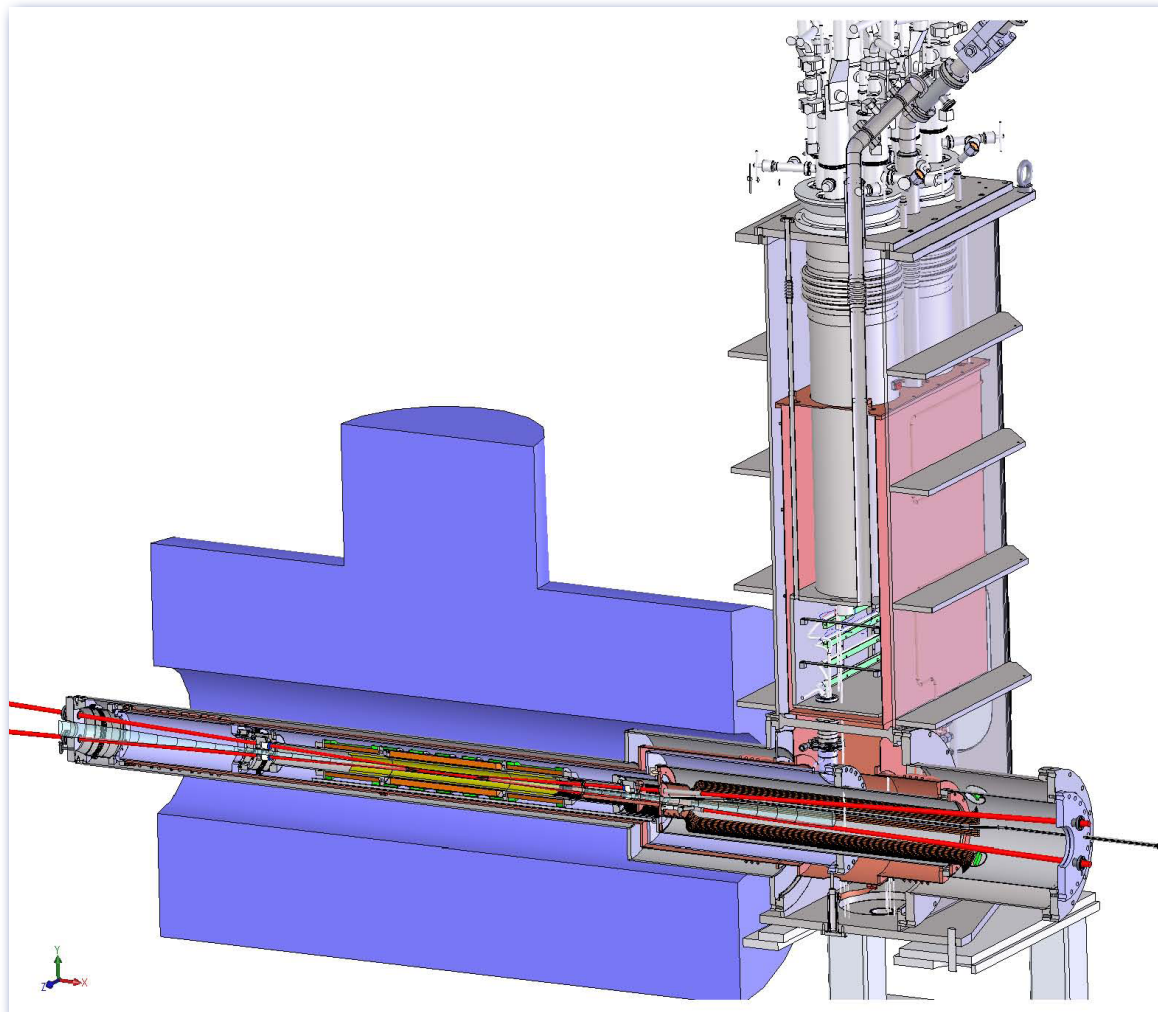
Une vue 3D du nouvel aimant (en violet) et du cryostat. Les lignes rouges montrent la trajectoire des faisceaux laser. Les lignes de courant pour les aimants supraconducteurs, du type de ceux du LHC, sont visibles en haut à droite de l'image.
