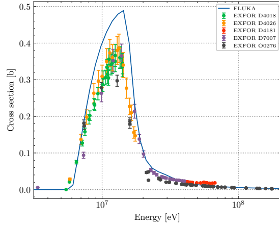
(d) ^{\text{nat}}\text{Fe}(p, x)^{56}\text{Co}
