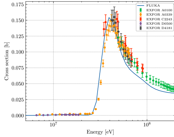
(f) ^{\text{nat}}\text{Fe}(p, x)^{54}\text{Mn}
