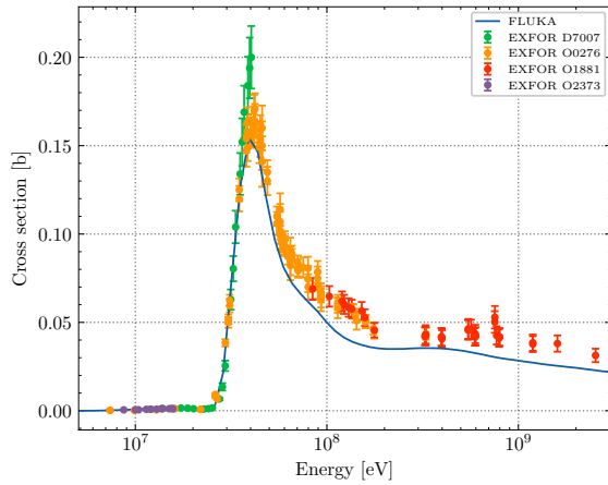
(g) ^{\text{nat}}\text{Fe}(p, x)^{54}\text{Mn} (cont.)
