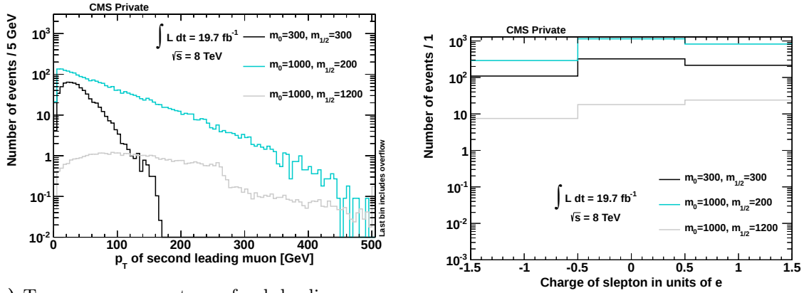
(c) Transverse momentum of sub-leading muon, p_{T,st\mu} > 5 GeV. (d) Charge of slepton.
