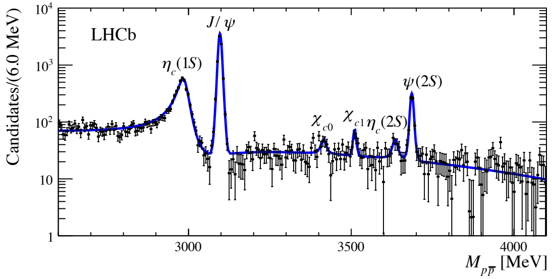
Figura 3.1: Grafici riportati nell'articolo della collaborazione LHCb per l'osservazione del decadimento \eta_c(2S) \rightarrow p\bar{p} [20].
