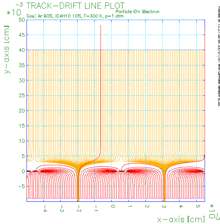
FIG. 4.5: Lignes de champ électrique dans Micromégas [33].
