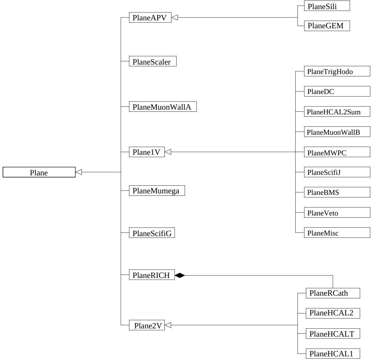
FIG. 3.4: Arbre généalogique des classes de plans. les flèches à pointe blanche signifient “ hérite de ”. On y retrouve Plane1V ainsi que deux autres familles. PlaneAPV regroupe les GEM et les détecteurs au silicium, des détecteurs de traces utilisant une électronique de lecture identique. Plane2V comprend les détecteurs à damier, pour lesquels le canal est repéré par un couple de coordonnées entières. Ces détecteurs sont les calorimètres hadroniques HCAL1 et HCAL2, ainsi que les photocathodes du RICH. À l’arrivée du calorimètre électromagnétique ECAL1, il suffira de créer une classe vide PlaneECAL1 , et de la placer également sous Plane2V . Certaines classes sont isolées : il s’agit des Micromégas et des fibres scintillantes allemandes dont le système de lecture est particulier, ainsi que du RICH. Celui-ci est un plan composite possédant comme variables 16 objets appartenant à la classe PlaneRCath , qui décrivent les 16 photocathodes (la flèche à losange noir signifie “ appartient à ”).
