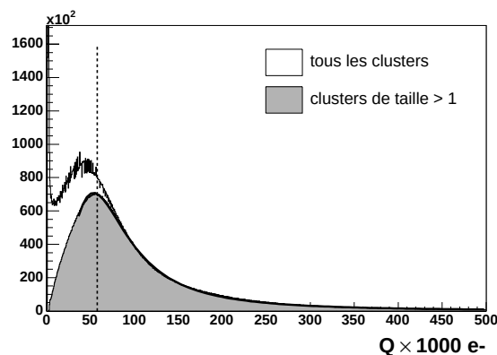
FIG. 5.20: Extraction de l'amplitude moyenne des clusters d'un Micromégas. La ligne verticale indique l'amplitude moyenne.
