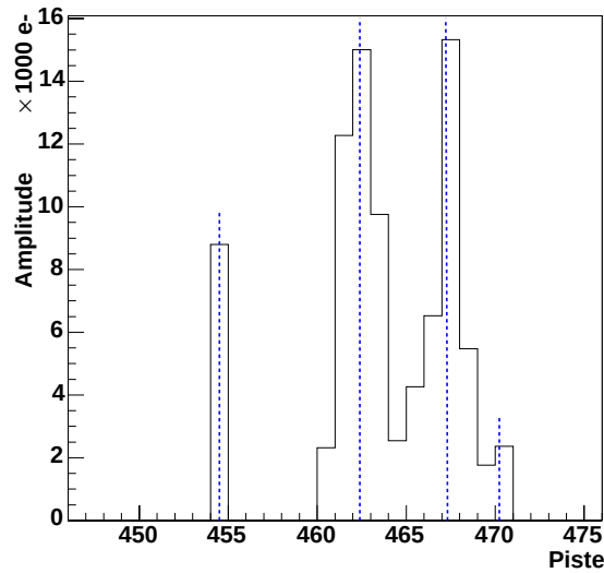
FIG. 5.17: Séparation des clusters. Un cluster de taille 11 (pistes 460→470) est séparé en trois clusters dont les positions sont repérées par les lignes pointillées.
