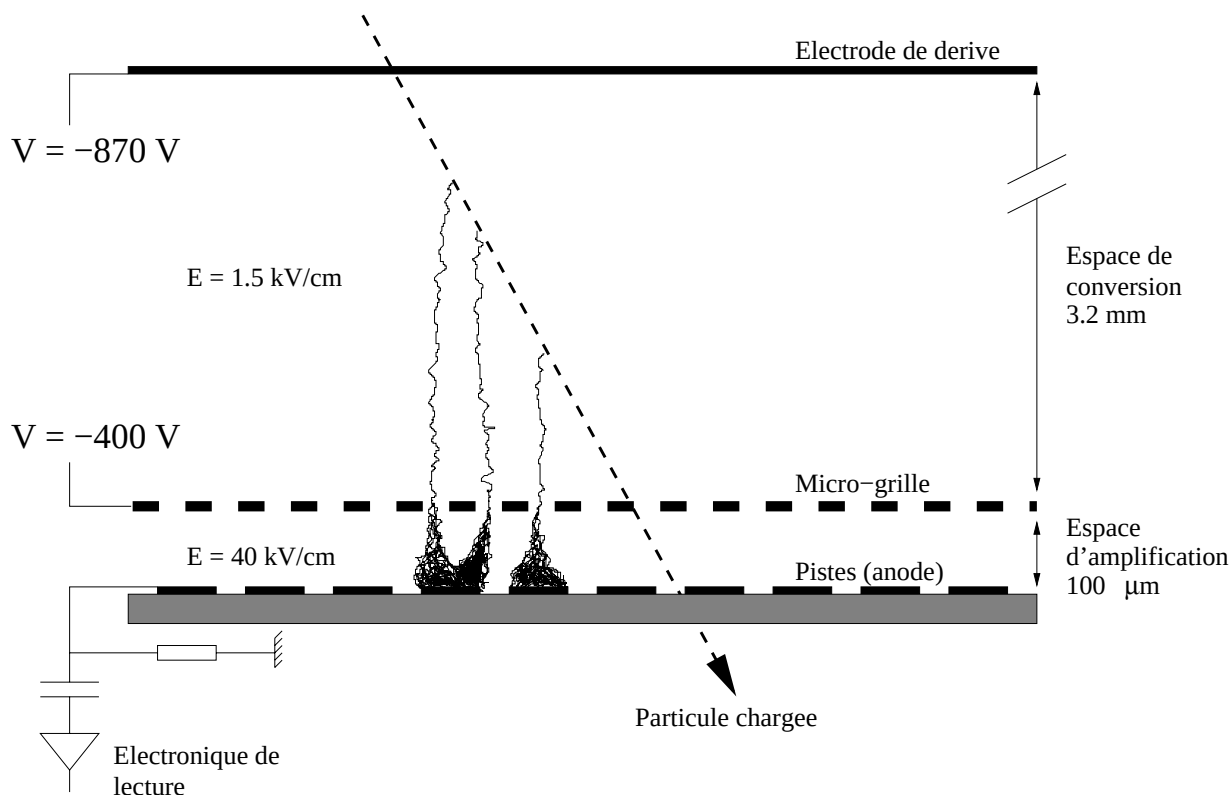
FIG. 4.4: Principe de fonctionnement d'un détecteur Micromégas.
