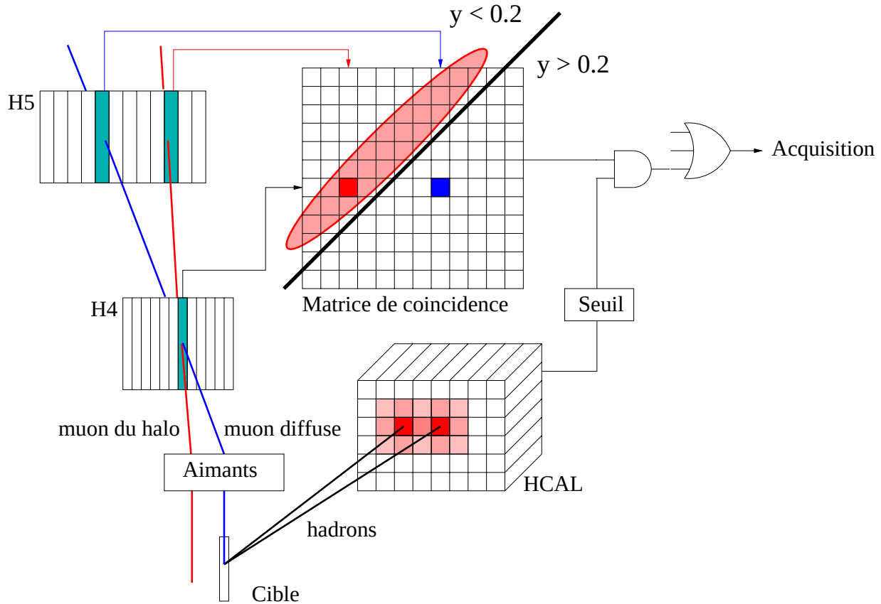
FIG. 2.13: Principe du trigger de COMPASS. Les signaux provenant des canaux de H4 et H5 sont envoyés vers une matrice de coïncidence qui génère un signal seulement si l'inclinaison du muon après le passage des dipôles SM1 et SM2 est suffisante pour correspondre à y > 0.2 . Cette coupure élimine la majeure partie du halo du faisceau. Afin de réduire le bruit de fond, on requiert une coïncidence entre le signal produit par la matrice et le signal des calorimètres.
