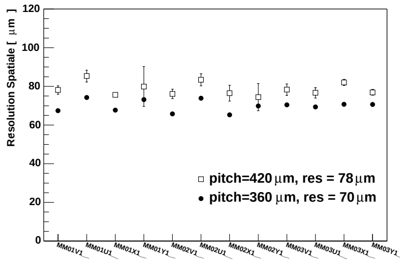
FIG. 5.13: Effet du pas des pistes sur la résolution spatiale, pour chacun des Micromégas.
