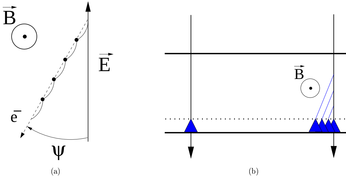
FIG. 5.15: (a) Mouvement d'un électron sous un champ électrique et un champ magnétique perpendiculaires. Les points symbolisent les interactions avec les atomes du gaz. (b) Effet du champ sur les électrons résultant du passage d'une particule dans un Micromégas. En présence de champ, les électrons atteignent la micro-grille d'autant plus loin du point d'impact de la particule que la distance à parcourir depuis le lieu de l'ionisation est grande.
