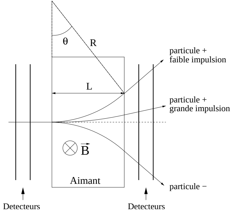
FIG. 2.8: Principe d'un spectromètre.
