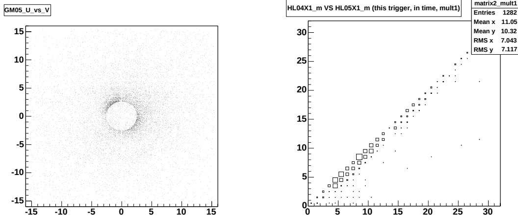
FIG. 3.5: Exemples d'application des groupes de plans. À droite, profil 2D d'un objet de classe GroupGEM . À gauche, matrice de coïncidence d'un objet de classe GroupTrigHodo .
