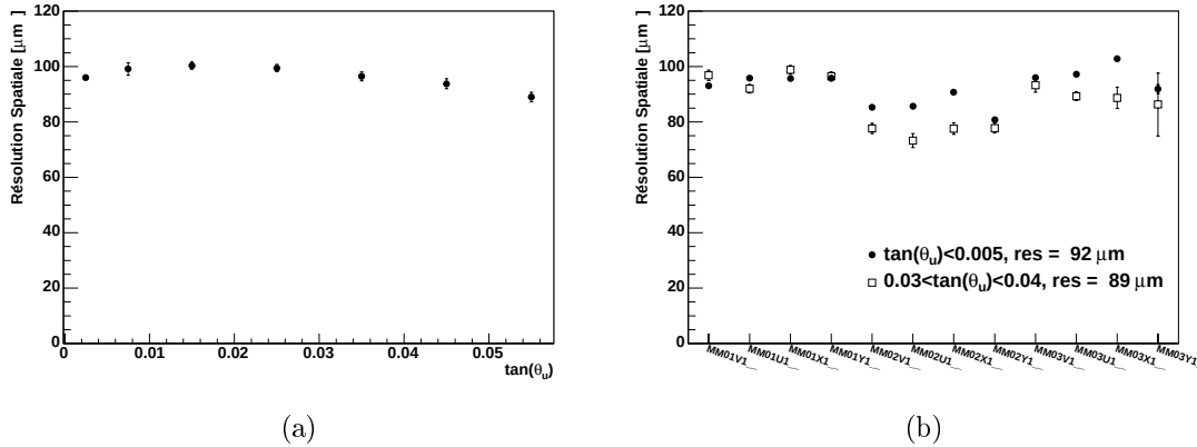
FIG. 5.19: (a) Résolution en fonction de l'inclinaison des traces pour MM01Y1. (b) Effet de l'angle sur la résolution des 12 Micromégas.
