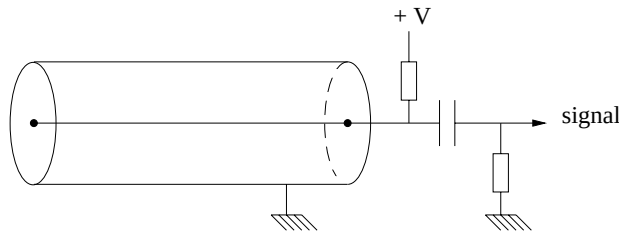
FIG. 4.1: Le compteur à fil.
