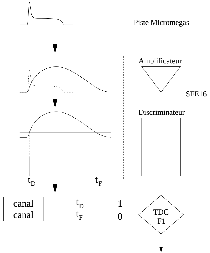
FIG. 4.7: Principe de fonctionnement de l'électronique frontale des Micromégas.
