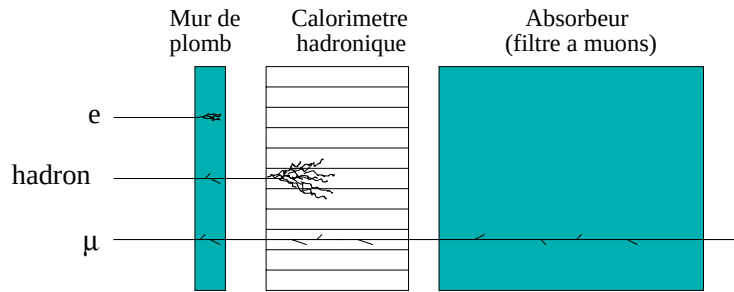
FIG. 2.10: Perméabilité aux différentes particules du mur de plomb, du calorimètre hadronique et du filtre à muons.
