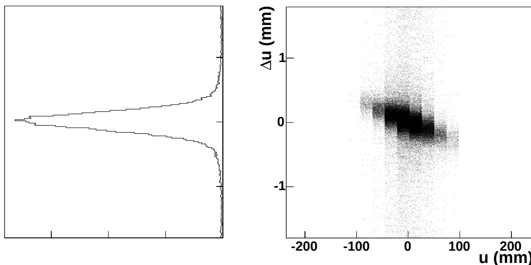
FIG. 5.11: À gauche : distribution des résiduels pour le détecteur MM01Y1. À droite : histogramme \Delta u vs u . Dans cet histogramme, la pente est due à une mauvaise description du pas des pistes de ce détecteur. La distribution des résiduels, obtenue en projetant cet histogramme sur son axe vertical, est par conséquent élargie.
