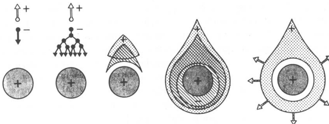
FIG. 4.3: Développement au cours du temps de l'avalanche au voisinage d'un fil d'anode. Du fait de la diffusion latérale, une avalanche en forme de goutte entoure le fil. Les électrons sont collectés en \sim 1 ns, laissant un nuage d'ions positifs qui se dirigent lentement vers les cathodes [27].
