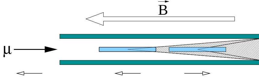
FIG. 2.6: L'acceptance de la cellule amont est plus faible que celle de la cellule aval. Les flèches à pointe blanche indiquent le sens de la polarisation du faisceau et de chacune des cellules.
