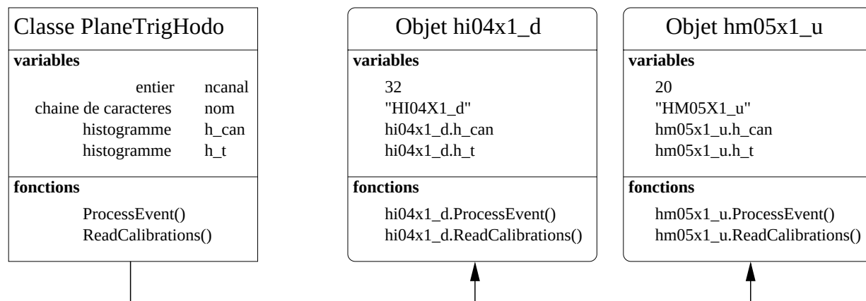
FIG. 3.2: Création de deux objets de classe PlaneTrigHodo . La notation hi04x1_d.h_can signifie : histogramme h_can appartenant au plan hi04x1_d . De même, la fonction hi04x_d.ProcessEvent() traite les données du plan hi04x1_d et remplit ses histogrammes.
