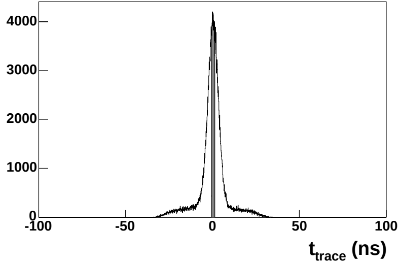
FIG. 5.9: Distribution temporelle des traces. En gris : sélection des traces fortement corrélées au trigger.
