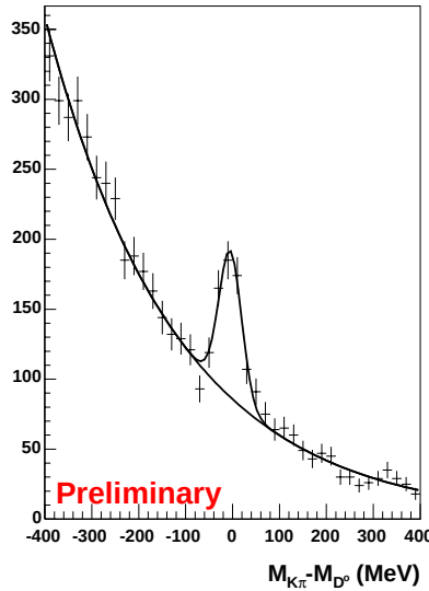
FIG. 2.2: Distribution de masse invariante des paires K^-\pi^+ et K^+\pi^- provenant du D^* , obtenue    partir de 909 runs acquis en 2002.
