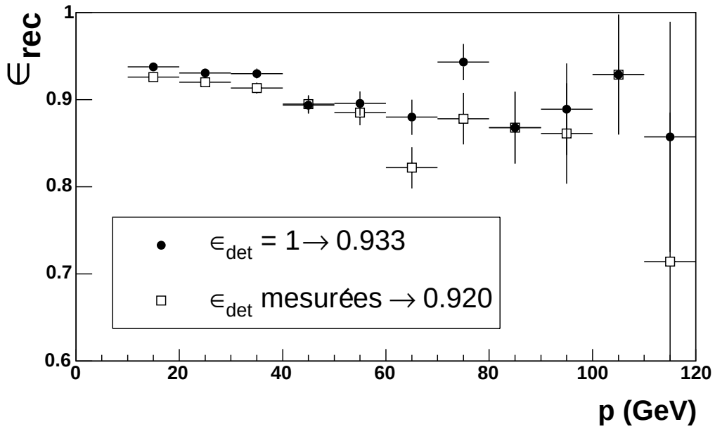
FIG. A.1: Efficacité de reconstruction du premier hadron en fonction de son impulsion, avec et sans la prise en compte des efficacités des détecteurs.
