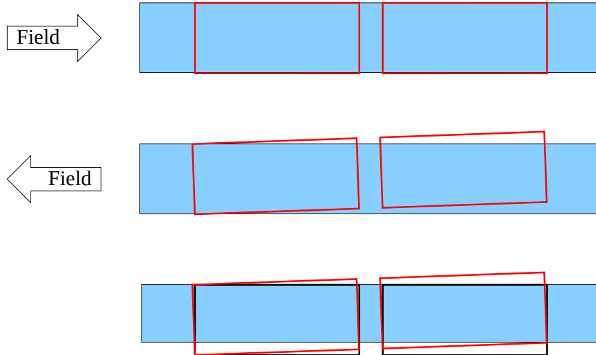
FIG. 6.14: Haut et centre : le mouvement de la cible lors de la rotation de champ induit une variation du rapport n_m/n_v . Bas : Des coupures plus étroites autour de la cible permettent de s'affranchir de cette variation.
