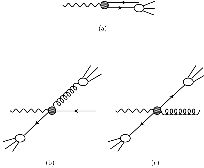
FIG. 2.3: Principe de la sélection de PGF par la leptoproduction de hadrons à grande impulsion transverse. Le DIS à l'ordre 0 (a) est un processus 2 \rightarrow 1 (2 particules dans l'état initial, 1 dans l'état final) : l'impulsion transverse du quark final est donc nulle. La diffusion Compton QCD (b) et la fusion photon-gluon (c) sont des processus 2 \rightarrow 2 : les particules de l'état final peuvent posséder une impulsion transverse. Comme les hadrons résultant de la fragmentation partent approximativement dans la direction du quark ou du gluon dont ils sont issus, sélectionner les événements contenant deux hadrons à grande impulsion transverse permet donc de réduire la contribution du DIS à l'ordre 0 à la section efficace.
