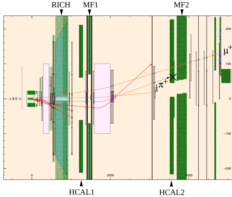
FIG. 2.11: Identification des muons. La quantité de matière présente sur le spectromètre est représentée en vert. Le RICH, rempli d'un gaz lourd ( C_4F_{10} ) apporte une quantité de matière non négligeable mais reste néanmoins perméable à toutes les particules. Le muon diffusé est détecté derrière le deuxième filtre à muons (MF2) alors que le pion est absorbé.
