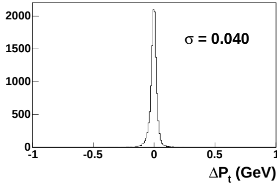
FIG. 7.6: Résolution sur la reconstruction de l'impulsion transverse des deux premiers hadrons, pour les événements grand p T .
