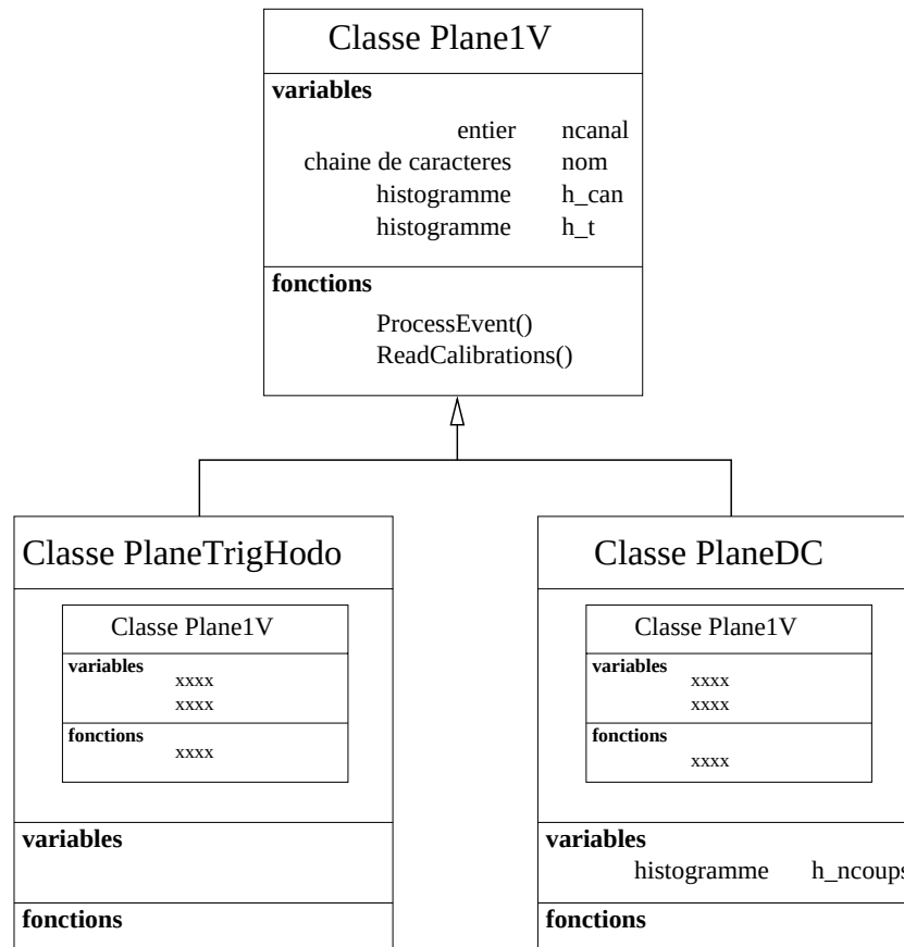
FIG. 3.3: Les classes PlaneTrigHodo et PlaneDC héritent de Plane1V , qui contient le code en commun. On a ajouté, à titre d'exemple, un histogramme à la classe PlaneDC , il apparaîtra dans tous les objets de cette classe.
