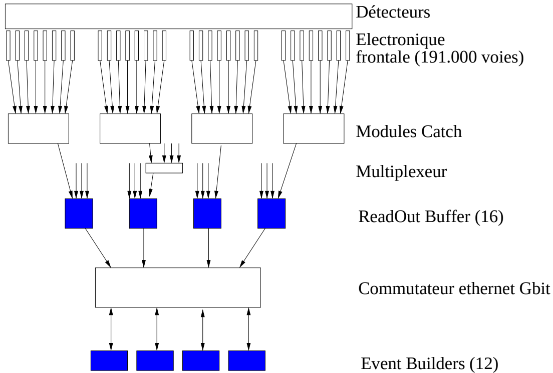
FIG. 2.14: Le système d'acquisition
