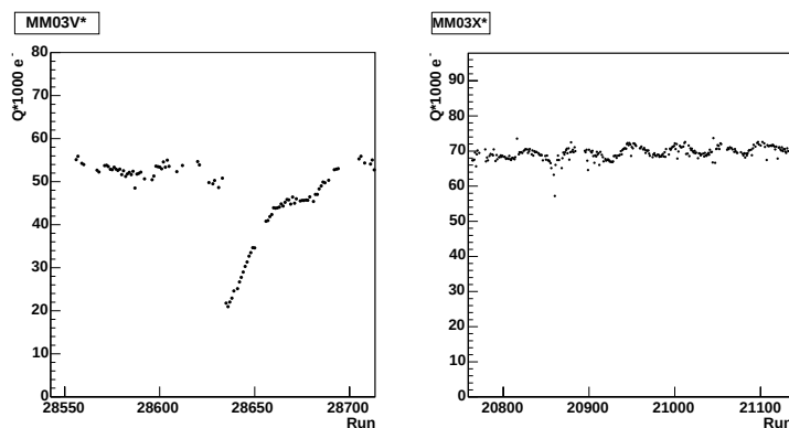
FIG. 5.21: à gauche : corruption du mélange gazeux après l'échange d'une bouteille de néon. À droite : oscillation de l'amplitude moyenne mesurée, avec une période de 24 h.
