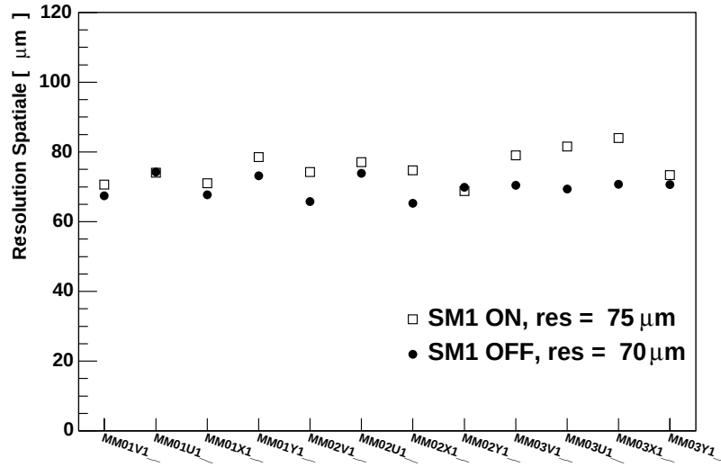
FIG. 5.14: Effet du champ de fuite de SM1 sur la résolution spatiale, pour chacun des Micromégas.
