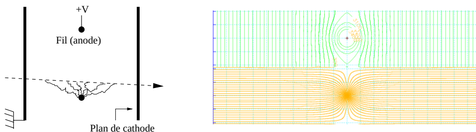
FIG. 4.2: La chambre proportionnelle multifils. À gauche, schéma de principe. À droite, configuration électrostatique : lignes équipotentiels en haut et lignes de champ en bas [26].
