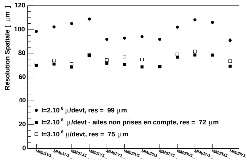
FIG. 5.16: Effet de l'intensité sur la résolution spatiale et rôle joué par les ailes de la distribution des résiduels dans la dégradation de la résolution spatiale à haute intensité.
