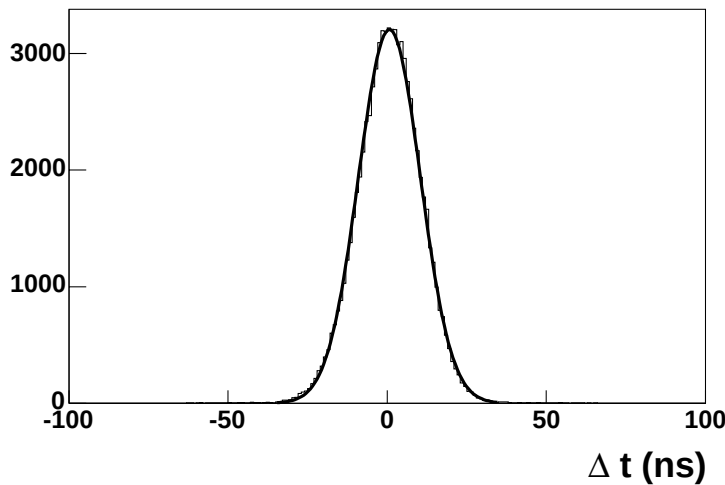
FIG. 5.8: Distribution des \Delta t = t_{\text{cluster}} - t_{\text{trace}} dans MM01V1, à basse intensité. Cette distribution est presque parfaitement gaussienne.
