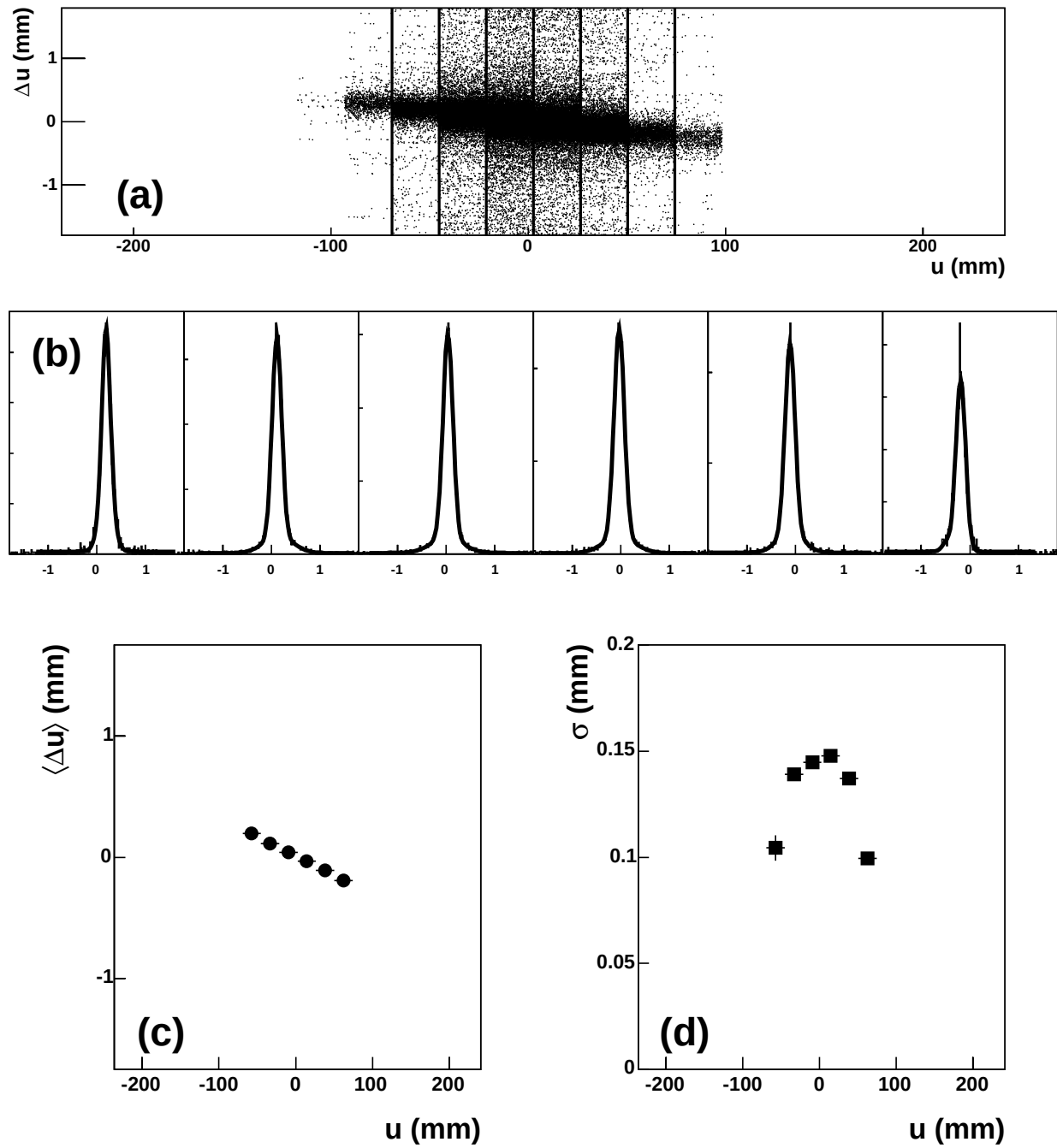
FIG. 5.12: Extraction de \sigma . De haut en bas : histogramme \Delta u vs u pour MM01Y1 ; ajustements de chacun des canaux de \Delta u vs u ; position de la moyenne pour chaque canal ; \sigma(u) pour chaque canal. \sigma(u) est plus élevé au centre du détecteur car la résolution spatiale est moins bonne à haut flux, comme nous le verrons dans la section 5.5.4.
