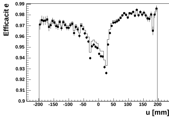
FIG. 5.6: Profil d'efficacité du détecteur MM02V dans la direction perpendiculaire aux pistes. Le trait plein correspond à l'expression naïve de l'efficacité, les points incluent la correction des effets de flux.
