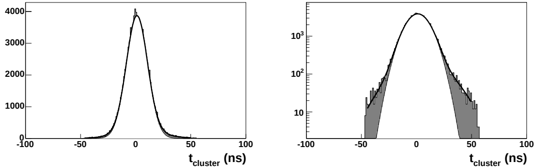
FIG. 5.10: Distribution des t_{cluster} dans MM01V1 (échelles linéaire et logarithmique). En gris, la deuxième composante gaussienne, présente uniquement à haute intensité.
