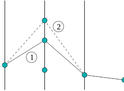
FIG. 3.6: Accélération de LSTRACK. Lors du test de la combinaison de clusters 1 (trait plein), il est possible de rejeter également la combinaison 2 (trait pointillé).
