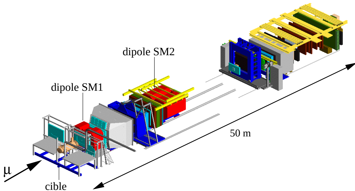
FIG. 2.4: Vue d'ensemble de COMPASS.
