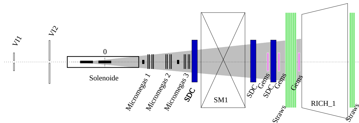
FIG. 5.1: Implantation des 3 stations de Micromégas dans le LAS.
