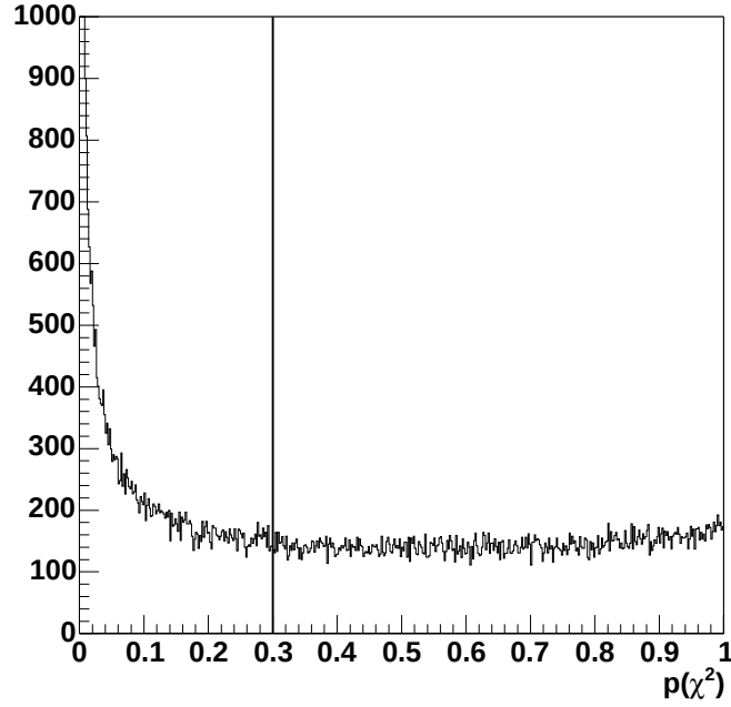
FIG. 5.3: Distribution de probabilité de \chi^2 après alignement. On conservera uniquement les traces telles que p(\chi^2) > 0.3 .
