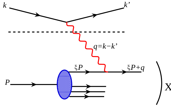
FIG. 1.2: Diffusion lepton-nucléon dans le modèle des partons.
