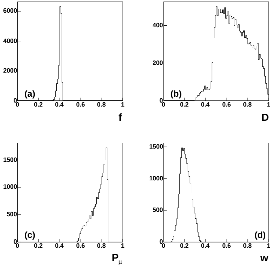
FIG. 6.1: Distributions de f , D , P_\mu et w = fDP_\mu pour un échantillon d'événements grand p_T . La rupture observée dans la distribution de D est due à la coupure y > 0.4 (voir la sélection des événements grand p_T , section 6.2). De plus, cette distribution comporte visiblement deux populations d'événements ( D \simeq 0.4 et D > 0.5 ), ce qui sera expliqué dans la section 6.1.3.
