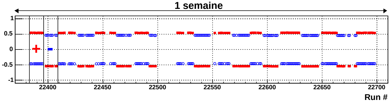
FIG. 6.2: Période P2E . La ligne grisée indique l'orientation des spins dans la cellule amont, les cercles vides l'orientation dans la cellule aval.
