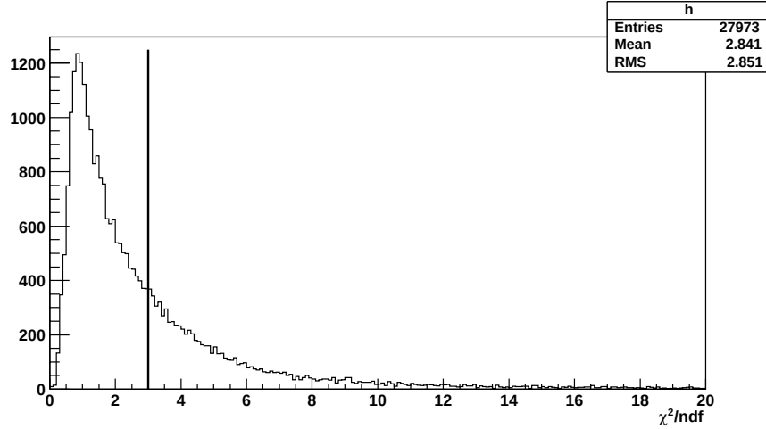
FIG. 5.2: Distribution en \chi^2/n_{df} des traces sélectionnées pour les mesures d'efficacité et de résolution en conditions nominales. Seules les traces de \chi^2/n_{df} < 3 sont conservées.
