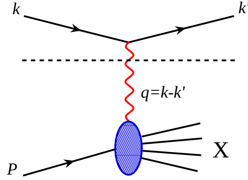
FIG. 1.1: Diffusion lepton-nucléon.
