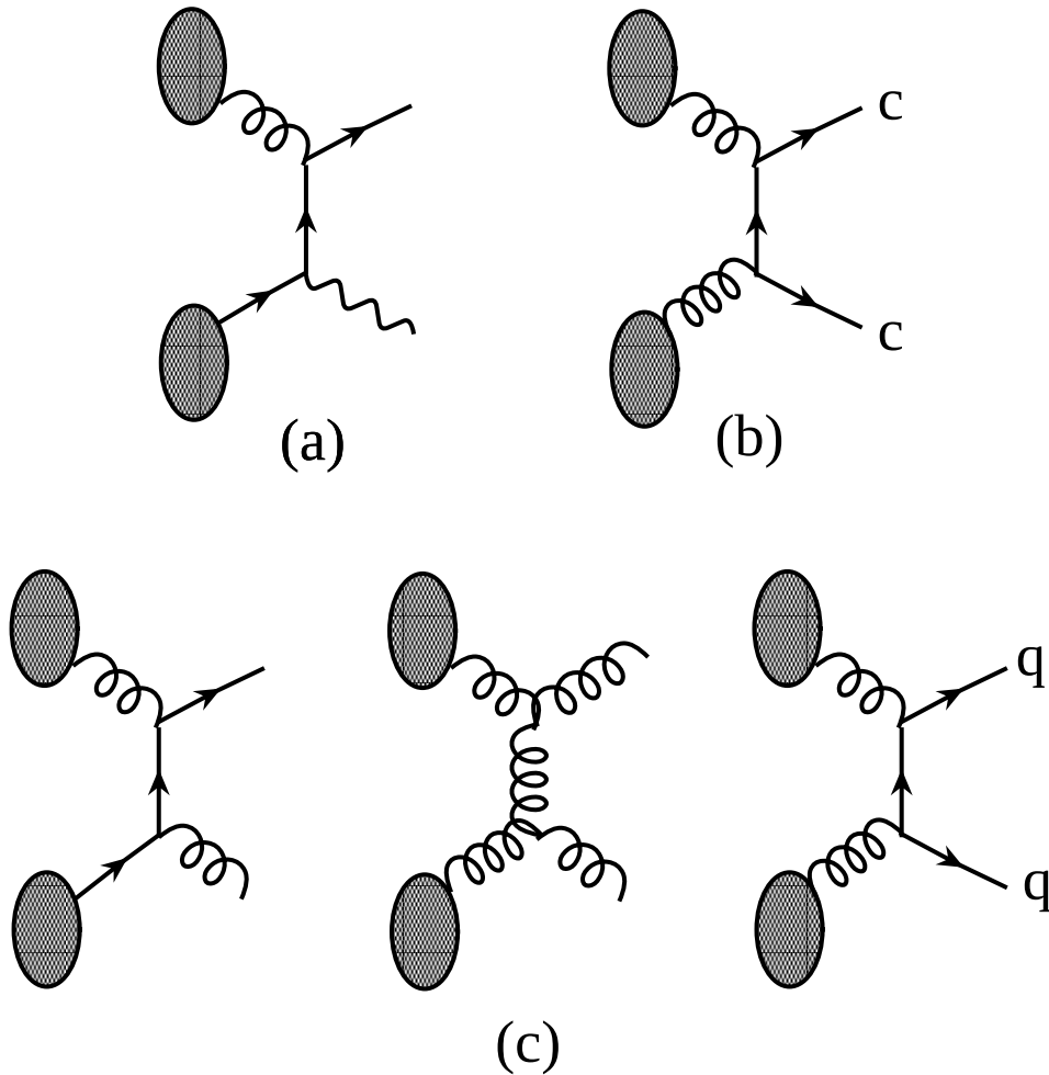
FIG. 1.7: Expérience STAR : sélection des réactions impliquant des gluons. (a) \gamma -jet. (b) production de charme ouvert. (c) deux jets.
