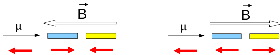
FIG. 6.9: Le réglage micro-ondes négatif correspond à une polarisation négative de la cellule amont. L'asymétrie est calculée par l'équation (6.21).
