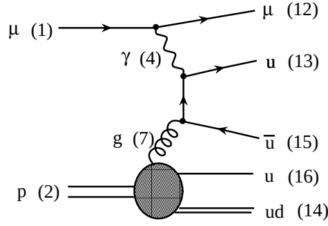
FIG. 7.3: Diagramme de Feynman correspondant à l'événement de la figure 7.2.
