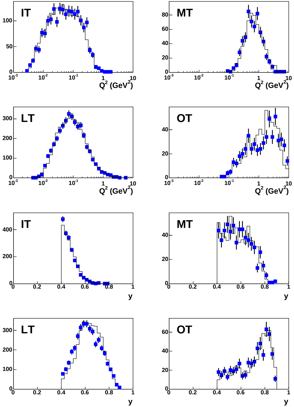
FIG. 7.10: Comparaison entre les données (histogramme) et la simulation (points). Distribution des variables cinématiques inclusives Q^2 et y , pour les quatre triggers IT, MT, LT et OT.
