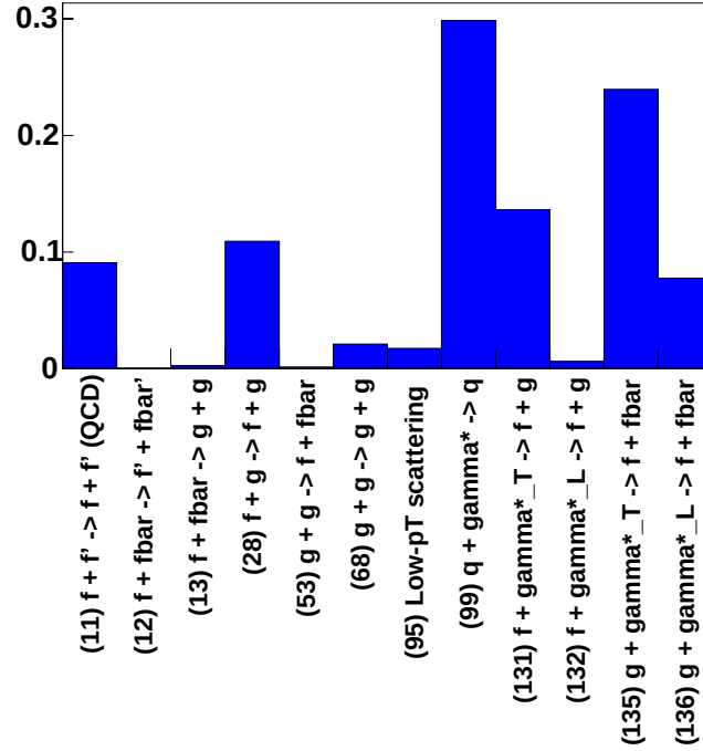
FIG. 7.17: Proportion des différents processus de PYTHIA dans l'échantillon grand p_T simulé, pour Q^2 > 1 .
