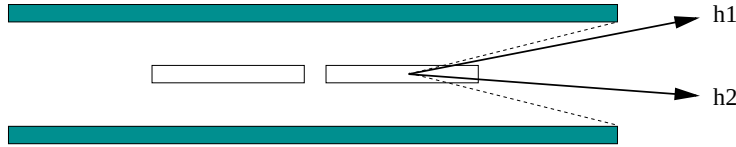
FIG. 7.7: Principe de la sélection des événements pour lesquels les deux premiers hadrons ne traversent pas le solénoïde de la cible.
