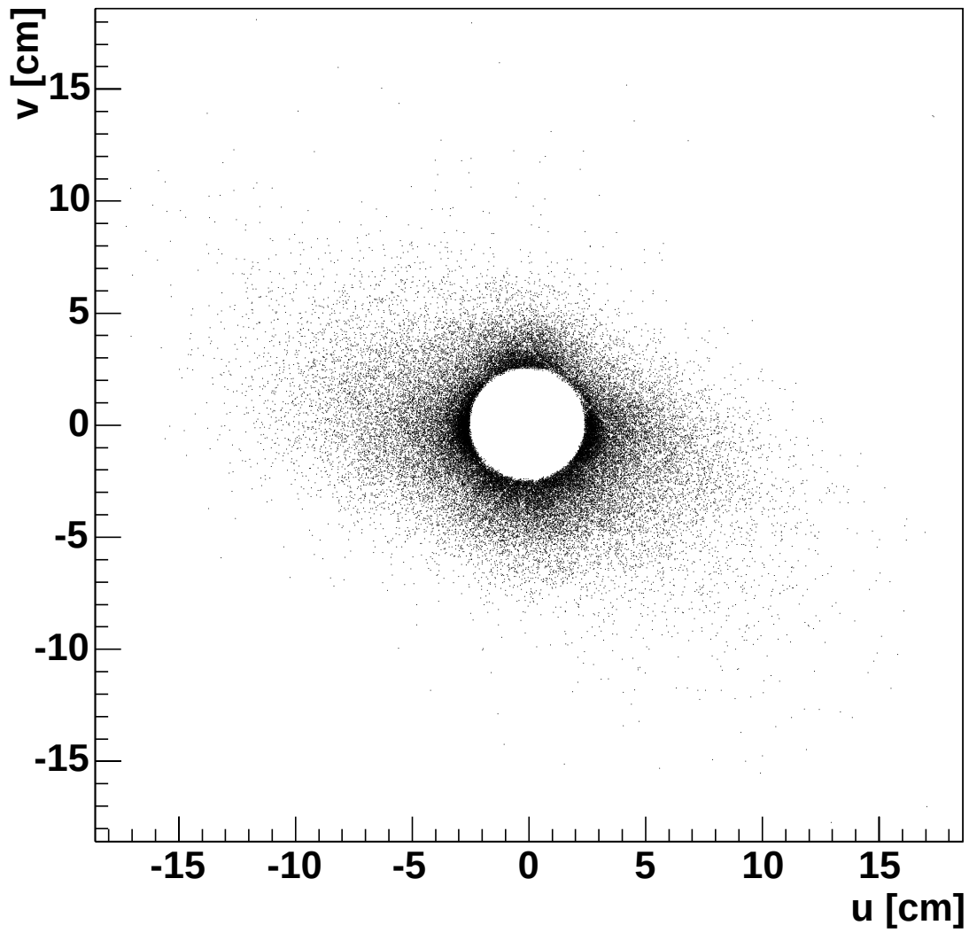
FIG. 5.4: Profil des traces p(\chi^2) > 0.3 extrapolées dans un plan de référence au centre du télescope. Le disque central de diamètre 5 cm correspond à la zone inactive des détecteurs.
