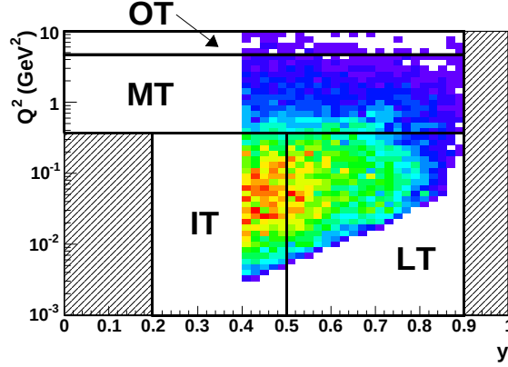
FIG. 7.8: Distribution de Q^2 en fonction de y pour les événements grand p T . On a représenté les régions couvertes par les 4 types de trigger .
