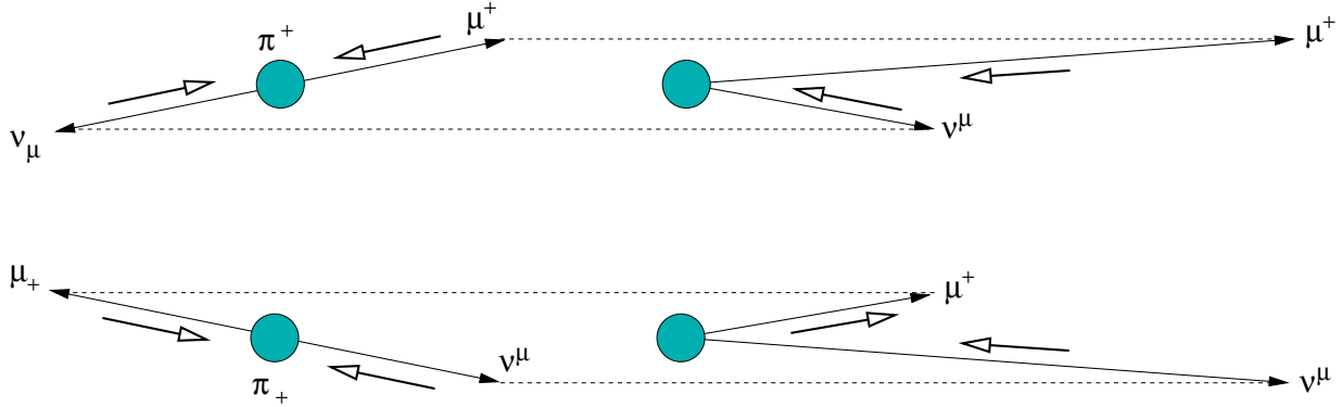
FIG. 2.5: Désintégration \pi^+ \rightarrow \mu^+ \nu_\mu , à gauche dans le référentiel du centre de masse du pion, à droite dans le laboratoire. En haut : émission du muon vers l'avant. En bas : émission du muon vers l'arrière.
