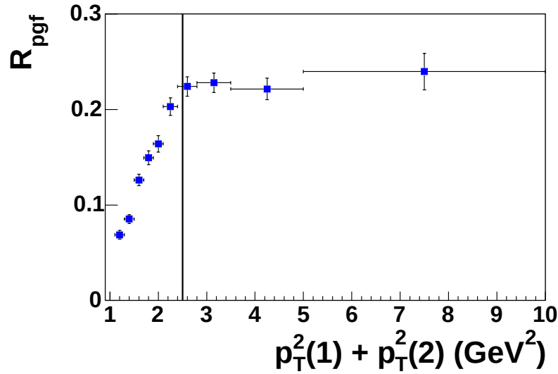
FIG. 7.14: R_{pgf} en fonction de p_T^2(1) + p_T^2(2) . La ligne représente la coupure p_T^2(1) + p_T^2(2) > 2.5 \text{ GeV}^2 , utilisée lors de la sélection de l'échantillon grand p T , pour les données réelles et la simulation.
