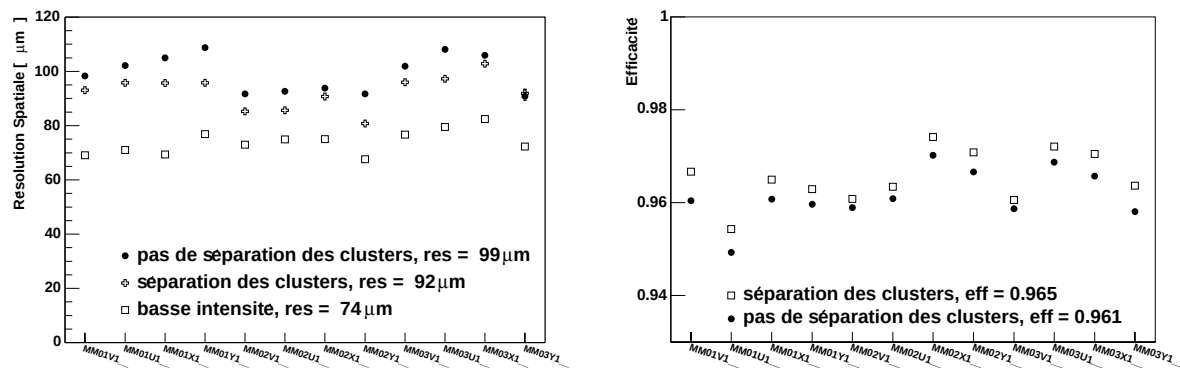
FIG. 5.18: Effet de la séparation des clusters sur la résolution spatiale (à gauche) et l'efficacité (à droite).
