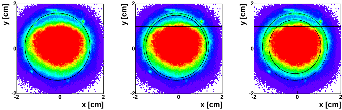
FIG. 6.11: Les trois jeux de coupures autour de la cible. À gauche : larges , R < 1.5 \text{ cm} . Au centre : optimales , R < 1.4 \text{ cm} and y < 1 \text{ cm} . À droite : étroites , R < 1.2 \text{ cm} and y < 1 \text{ cm} .
