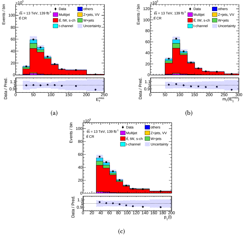
Figure R.14: Distribucions de (a) E_T^{\text{miss}} , (b) m_T(l, E_T^{\text{miss}}) i (c) p_T(l) en la regió de control de t\bar{t} , on es compara l'acord entre dades i simulacions de Monte Carlo dels processos del SM. Els esdeveniments del canal t , així com els dels fons de t\bar{t} i W +jets estan escalats utilitzant els resultats d'un ajust al nombre d'esdeveniments de dades en les regions de control i la regió de senyal.
