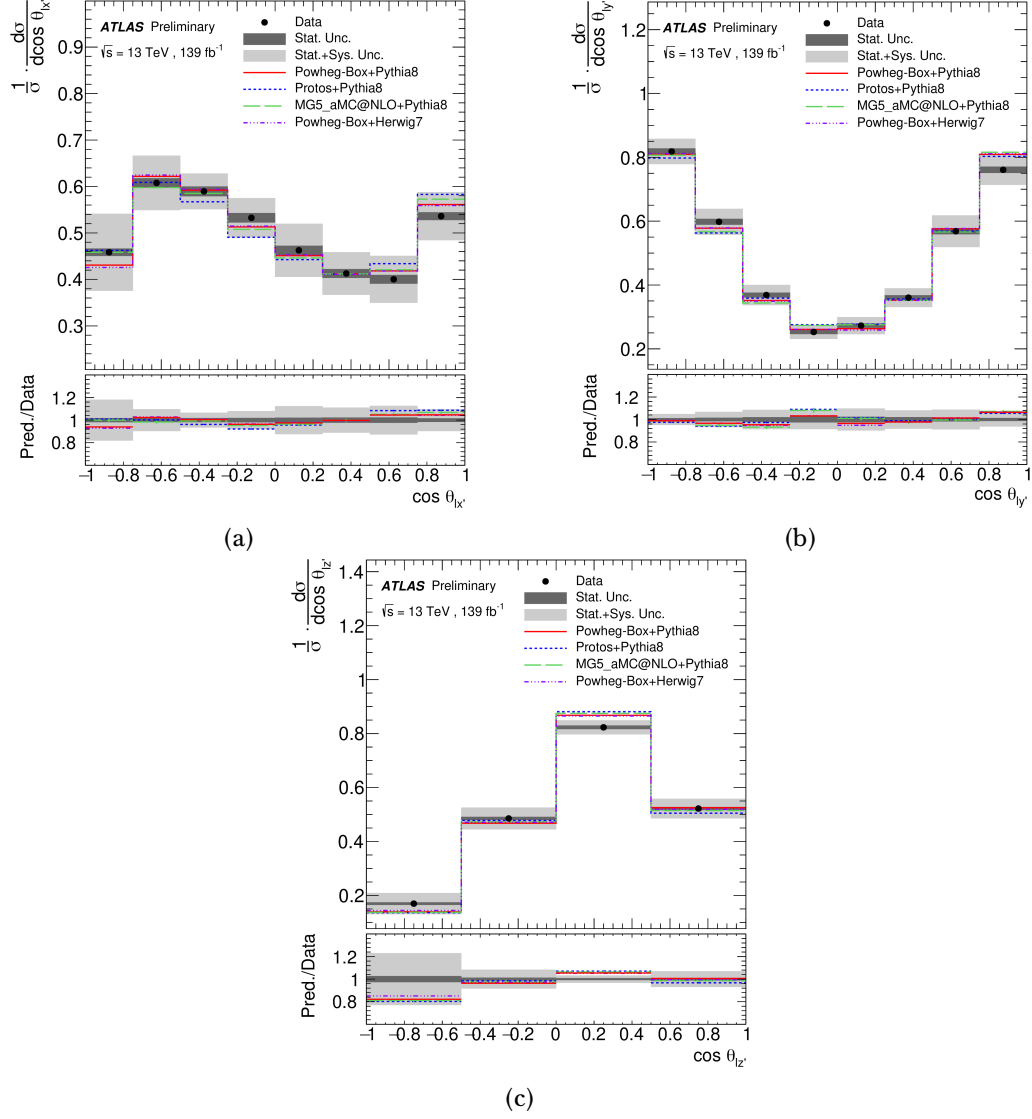
Figure R.16: Seccions eficaces diferencials normalitzades en funció de (a) \cos\theta_{lx'} , (b) \cos\theta_{ly'} i (c) \cos\theta_{lz'} , comparades amb diverses prediccions del SM obtingudes per simulació Monte Carlo, per a la mesura conjunta de quarks i antiquarks top.
