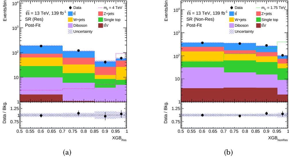
Figure R.24: Distribucions del XGBOOST en la regió de senyal dels models (a) ressonant i (b) no-ressonant després de l'ajust a les dades.
