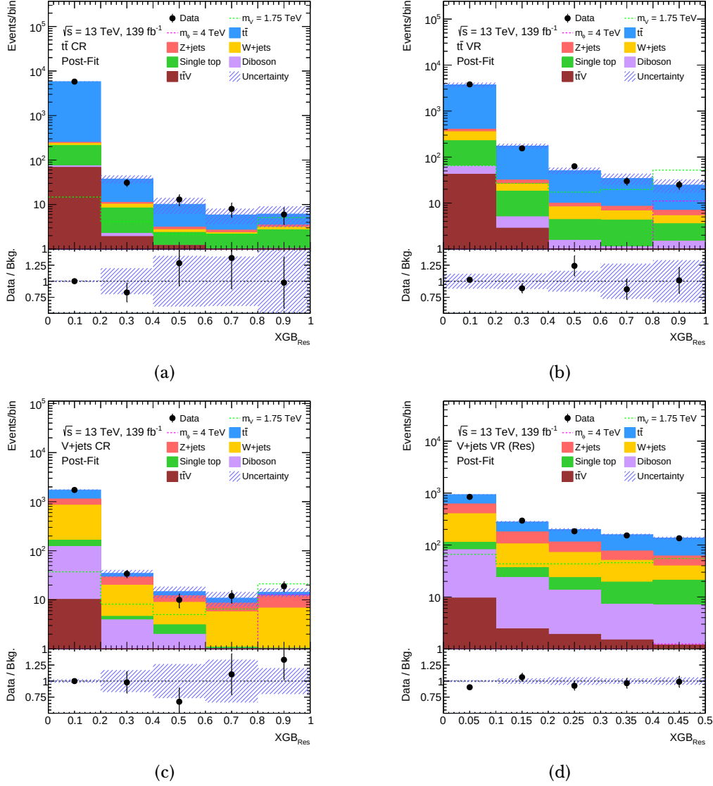
Figure R.22: Distribucions del XGBoost entrenat amb el model ressonant per a les dades i per als fons del SM, així com per als esdeveniments de senyal del model ressonant amb m_\phi = 4 TeV i del model no-ressonant amb m_V = 1.75 TeV a (a) la regió de control de t\bar{t} , (b) la regió de validació de t\bar{t} , (c) la regió de control de V +jets i (d) la regió de validació de V +jets del model ressonant.
