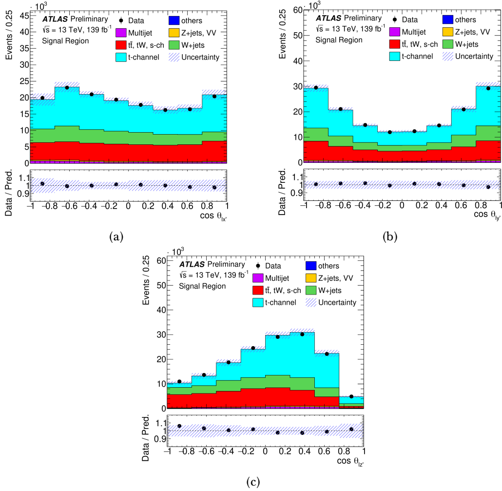
Figure R.15: Distribucions de (a) \cos \theta_{lx'} , (b) \cos \theta_{ly'} i (c) \cos \theta_{lz'} en la regió de senyal, on es compara l'acord entre dades i simulacions de Monte Carlo dels processos del SM. Els esdeveniments del canal t , així com els dels fons de t\bar{t} i W +jets estan escalats utilitzant els resultats d'un ajust al nombre d'esdeveniments de dades en les regions de control i la regió de senyal.
