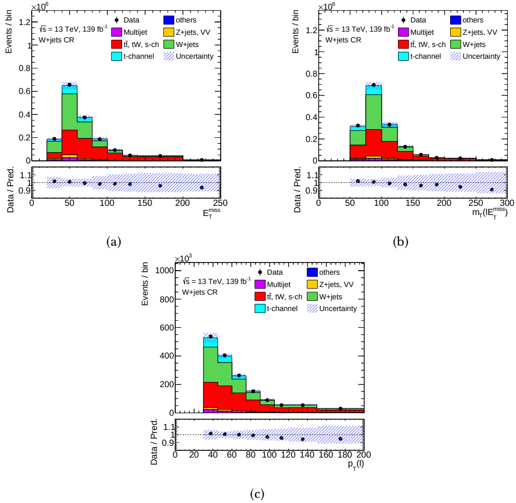
Figure R.13: Distribucions de (a) E_T^{\text{miss}} , (b) m_T(l, E_T^{\text{miss}}) i (c) p_T(l) en la regió de control de W +jets, on es compara l'acord entre dades i simulacions de Monte Carlo dels processos del SM. Els esdeveniments del canal t , així com els dels fons de t\bar{t} i W +jets estan escalats utilitzant els resultats d'un ajust al nombre d'esdeveniments de dades en les regions de control i la regió de senyal.
