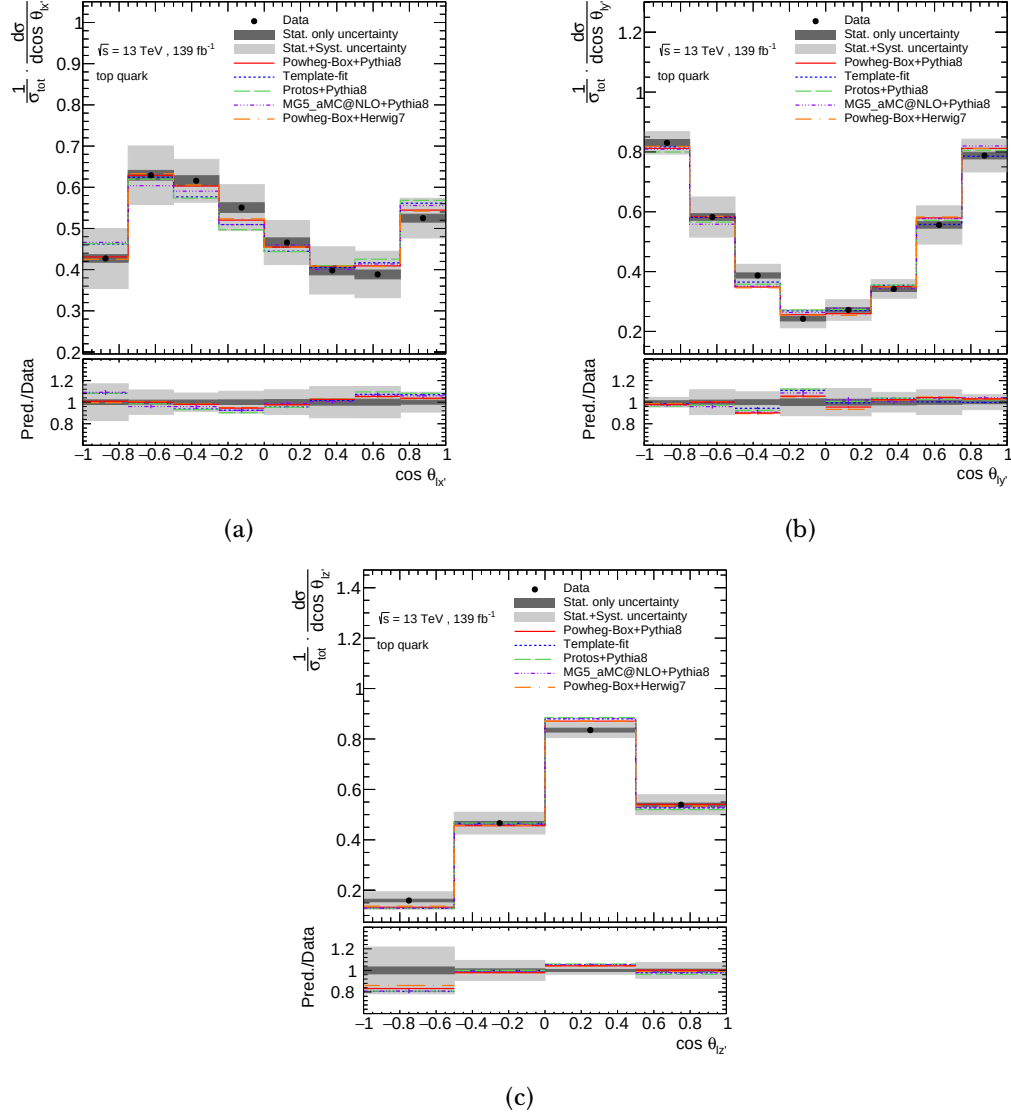
Figure R.17: Seccions eficaces diferencials normalitzades en funció de (a) \cos\theta_{lx'} , (b) \cos\theta_{ly'} i (c) \cos\theta_{lz'} , comparades amb diverses prediccions del SM obtingudes per simulació Monte Carlo, per a la mesura de quarks top. Els resultats també es comparen amb la mesura directa del vector de polarització del quark top, referenciada com a template-fit .
