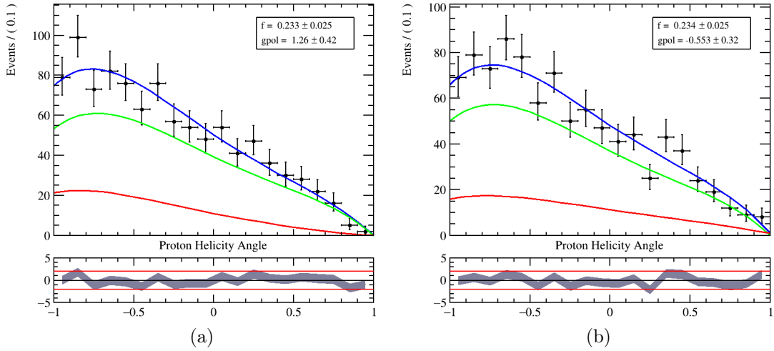
Figura 5: Ajust angular al cosinus de l'angle del protó per candidats (a) \Lambda_b^0 \rightarrow \Lambda \gamma and (b) \Lambda_b^0 \rightarrow \bar{\Lambda} \gamma . Dues contribucions són observables, provinents de la senyal i del fons.
