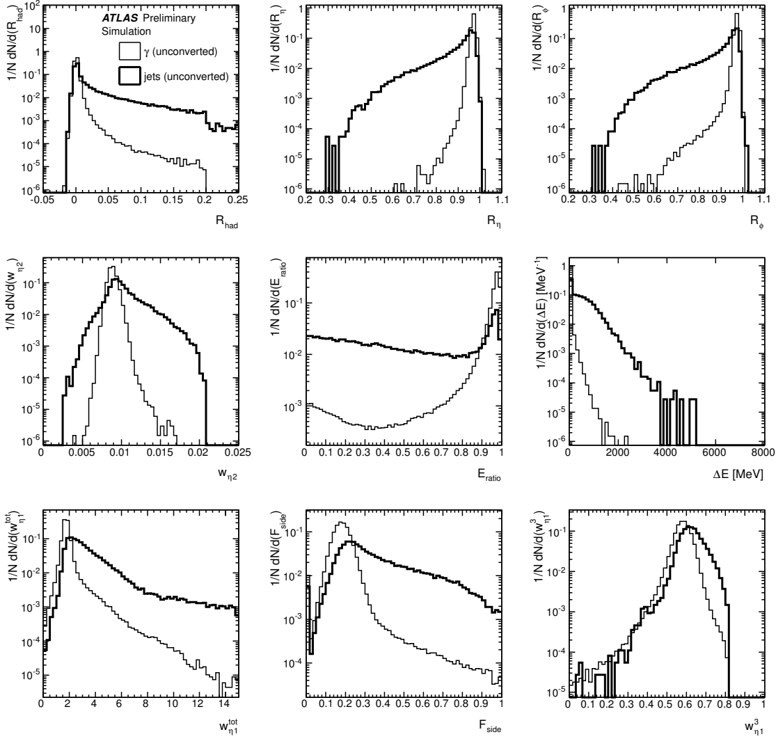
Figura 4.3 Distribuciones normalizadas de las variables discriminatorias calorimétricas en la región |\eta| < 0.6 para fotones reales y jets de E_T > 20 GeV reconstruidos como fotones no convertidos previo a cualquier selección.
