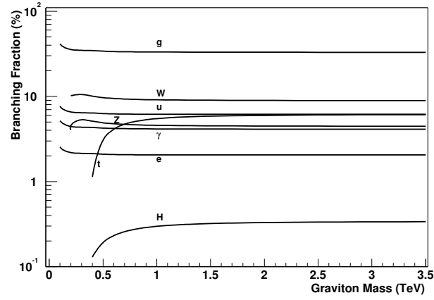
Figura 1.4 Tasa de decaimiento del gravitón RS en pares de partículas del Modelo Estándar [37].
