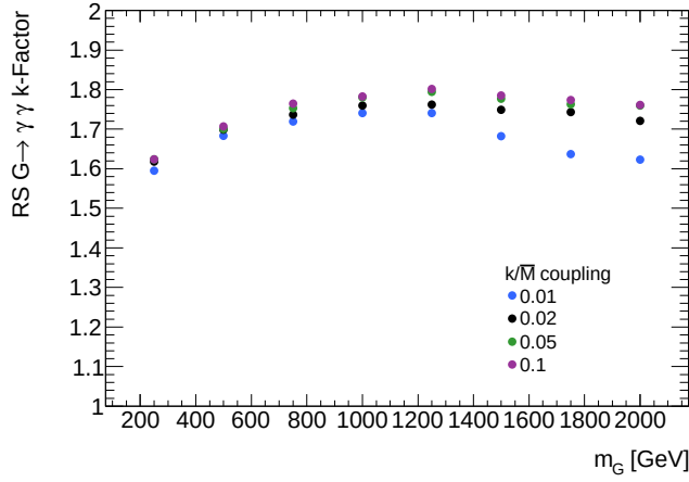
Figura 5.16 Correcciones NLO a la producción de gravitones RS como función de la m_G y para distintos valores de k/\bar{M}_{Pl} .
