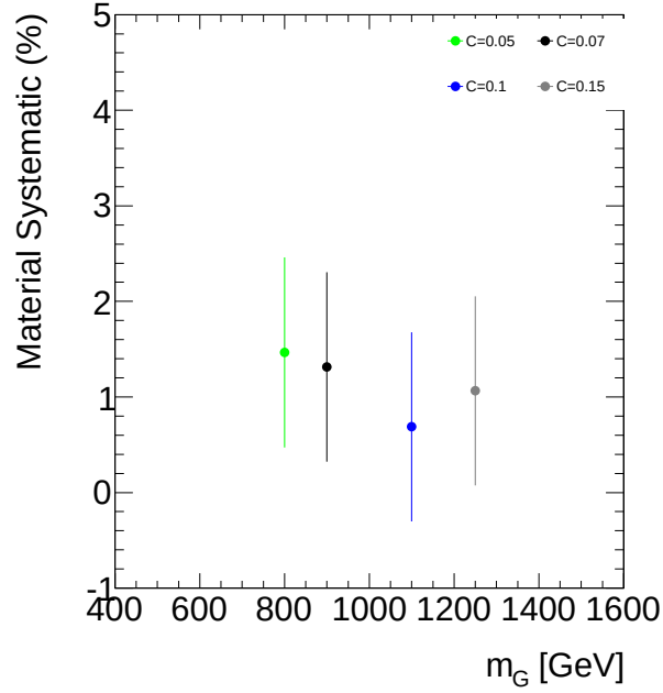
Figura 7.2 Incerteza sistemática en la eficiencia de selección de eventos de señal proveniente del desconocimiento de la composición exacta del material de cada uno de los subdetectores, calculada para gravitones tipo RS de distinta masa y acoplamiento.
