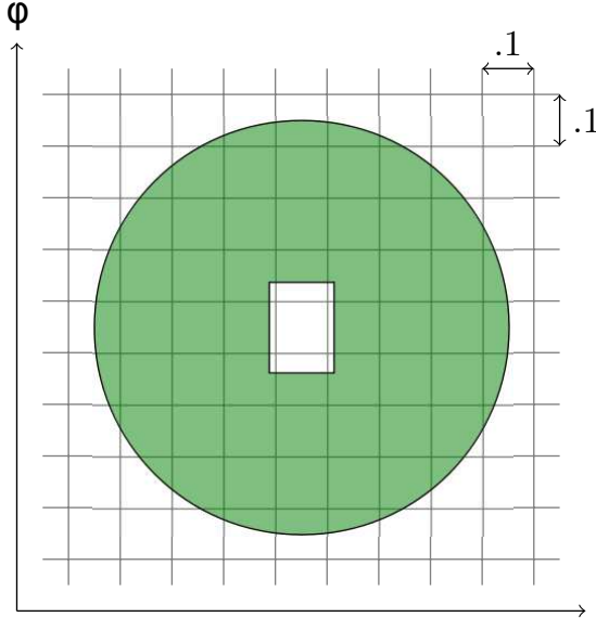
Figura 4.5 Ilustración del cono utilizado en el cálculo del aislamiento calorimétrico del fotón. El cono está centrado en la posición del baricentro del fotón y tiene un tamaño de \Delta R = 0.4 . A fin de sustraer la contribución propia del fotón, las celdas en la región central no se incluyen en la suma de la energía del cono.
