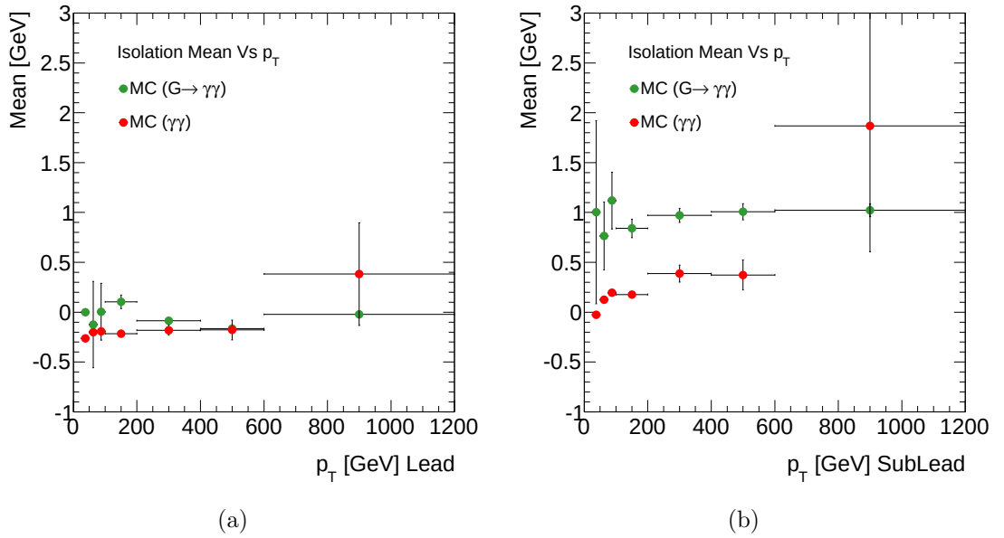
Figura 5.4 Valor medio del aislamiento calorimétrico como función del momento transversal del fotón. Se muestran los resultados para el fotón más energético (a) y el segundo más energético (b) en eventos tipo RS y \gamma\gamma del Modelo Estándar.
