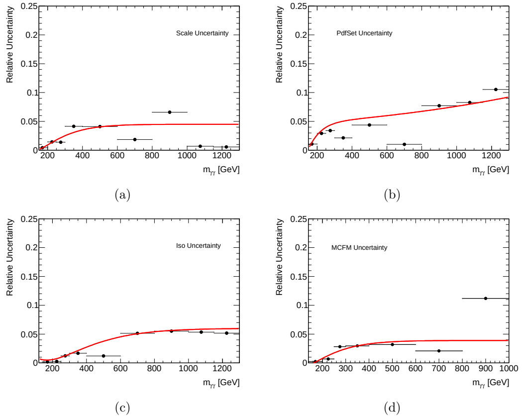
Figura 6.5 Incerteza sistemática en la predicción de DIPHOX como función de m_{\gamma\gamma} , proveniente de variaciones en (a) la escala, (b) las PDF, (c) el aislamiento, y (d) de la comparación con MCFM. La línea roja muestra la parametrización utilizada.
