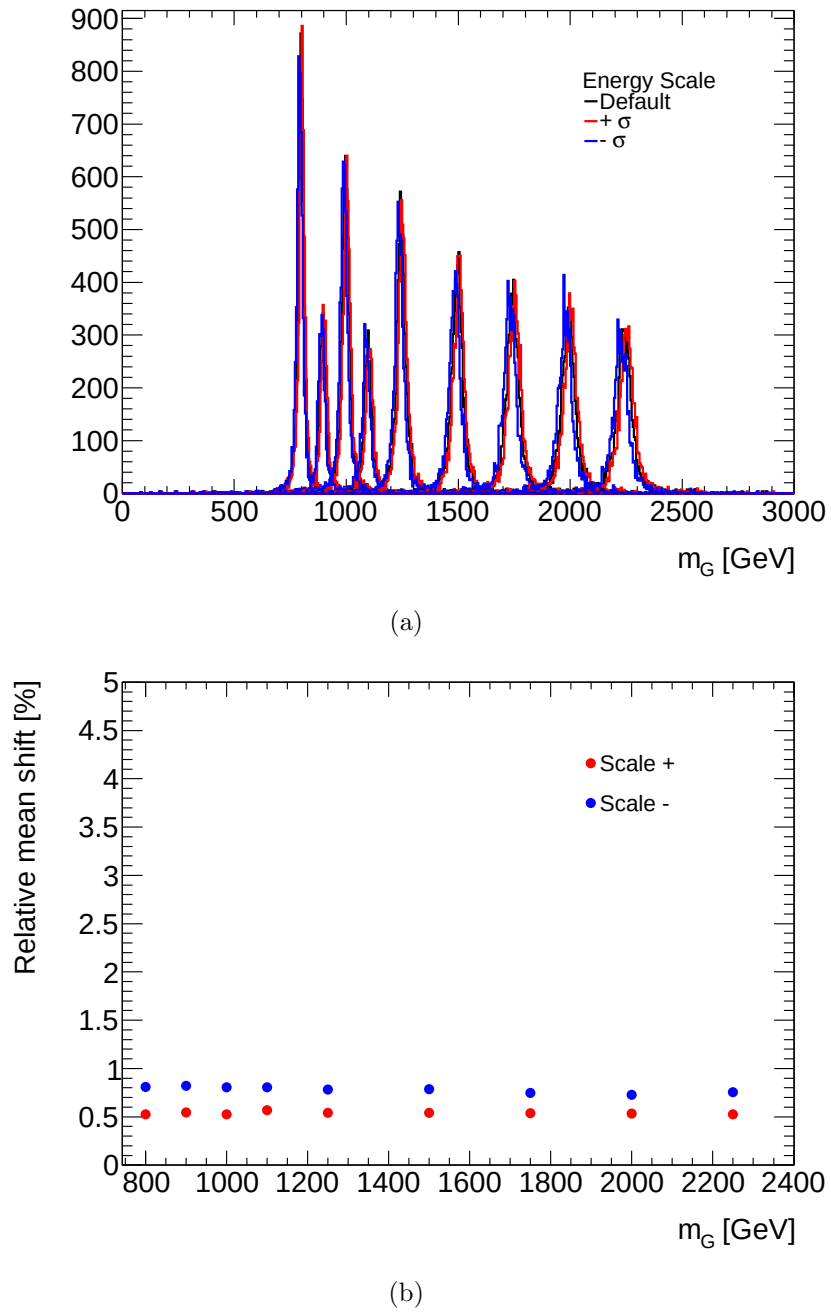
Figura 7.10 (a) Distribución de m_{\gamma\gamma} para gravitones RS con k/\overline{M}_{Pl}=0.1 y para distintos valores de m_G . Se muestran superpuestas las distribuciones obtenidas utilizando la escala de energía por defecto (negro) y aquellas obtenidas variando la misma en +\sigma (rojo) y -\sigma (azul) según la incerteza sistemática asociada a la corrección. (b) Corrimiento relativo de la media de la distribuciones de m_{\gamma\gamma} como función de m_G .
