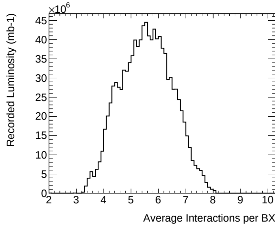
Figura 7.3 Distribución del número promedio de interacciones por bunch crossing en los datos colectados por ATLAS entre marzo y agosto del 2011.
