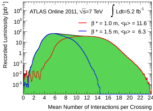
Figura 3.12 Media del número de interacciones por bunch crossing pesado por la luminosidad durante el año 2011. Se distinguen el período previo y posterior a Septiembre, cuando el parámetro \beta^* se redujo de 1.5 m a 1.0 m.
