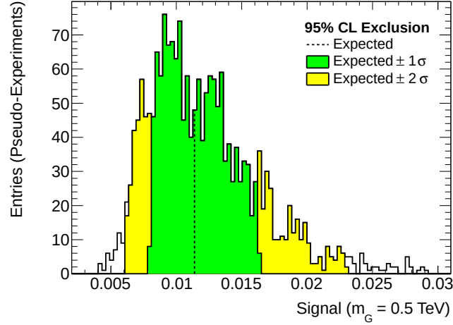
Figura 8.7 Distribución esperada del límite superior de \sigma B obtenida a partir de pseudo-experimentos en torno a la hipótesis del Modelo Estándar. Los resultados corresponden a un gravitón RS con m_G=0.5 TeV y k/\overline{M}_{Pl}=0.1 . Se distinguen el valor esperado (media) y las desviaciones en \pm 1\sigma (68%) y \pm 2\sigma (95%).
