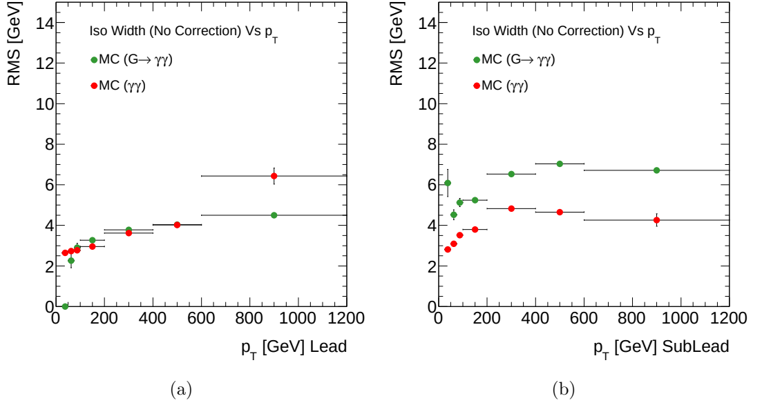
Figura 5.7 Como la Figura 5.5 pero con el aislamiento previo a las correcciones.
