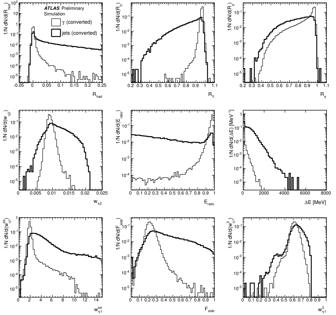
Figura 4.4 Distribuciones normalizadas de las variables discriminatorias calorimétricas en la región |\eta| < 0.6 para fotones reales y jets de E_T > 20 GeV reconstruidos como fotones convertidos previo a cualquier selección.
