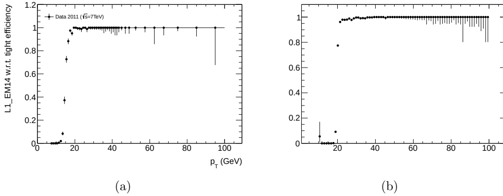
Figura 5.11 Eficiencias de selección \epsilon_{MinBias}^{L1\_EM14} (a) y \epsilon_{L1\_EM14}^{g20\_loose} (b) como función del p_T del fotón obtenidas por el método bootstrap . Para más detalles ver el texto.
