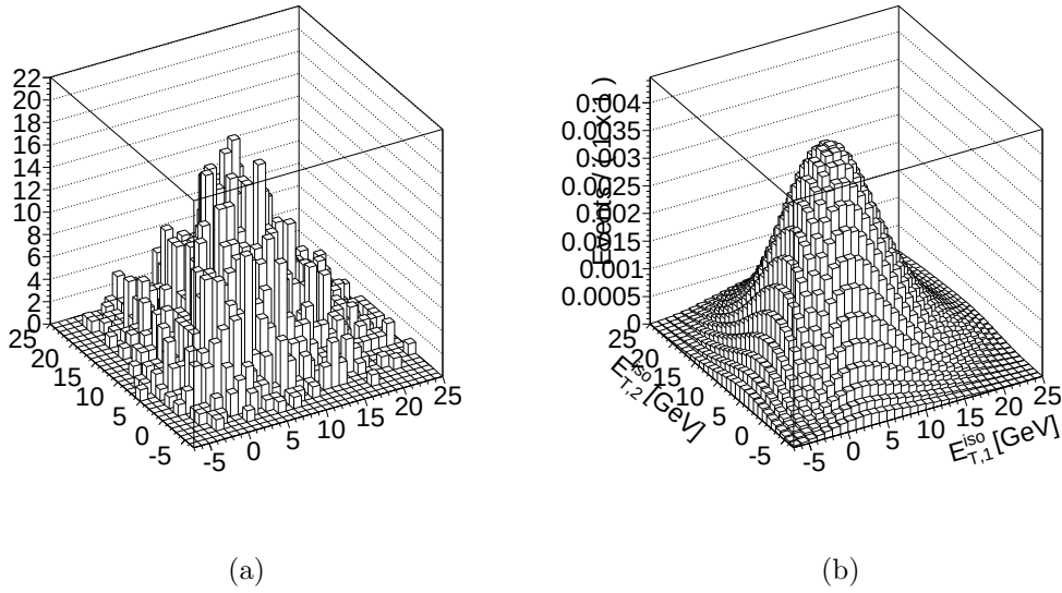
Figura 6.12 (a) Histograma 2D de eventos con dos candidatos a fotón donde ambos satisfacen la selección loose pero fallan la selección tight . (b) Versión suavizada del histograma anterior obtenida mediante el uso de la herramienta RooKeyPdf. Este último se identifica como la función de distribución conjunta de probabilidad de eventos di-jets ( J(E_{T,1}^{iso}, E_{T,2}^{iso}) ).
