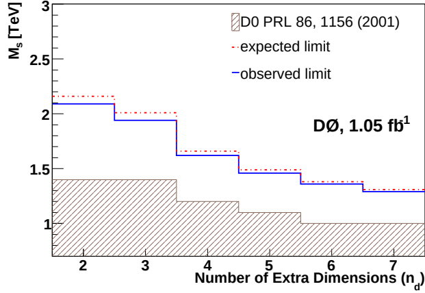
Figura 1.2 Límites de exclusión a 95% CL sobre la escala efectiva ( M_S ) como función del número de dimensiones extras para el formalismo de HLZ, provenientes del estudio del canal combinado \gamma\gamma/e^+e^- en el experimento D0 de Tevatron [9].
