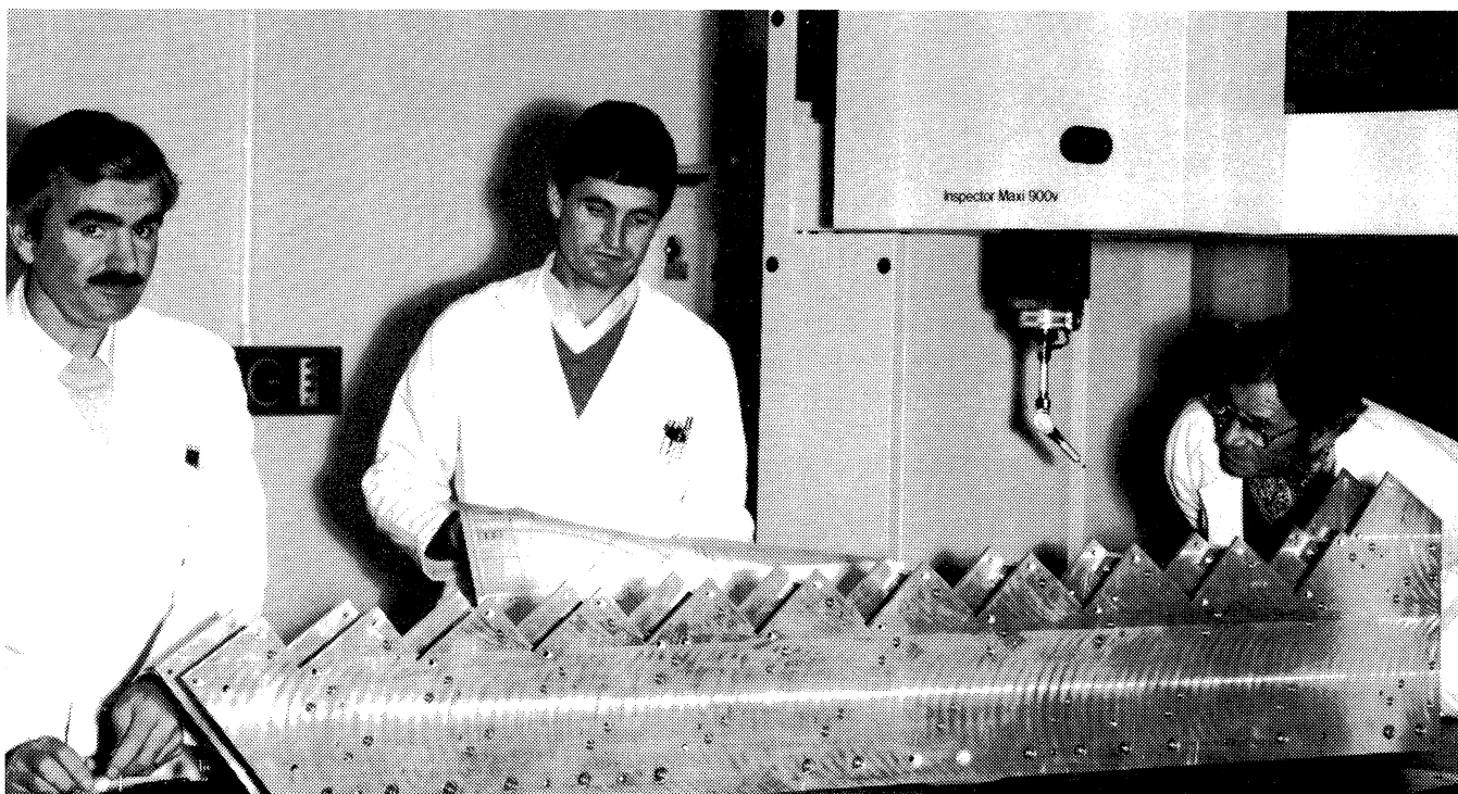
Examen sur notre nouveau dispositif de mesure d'une pièce mécanique qui n'est autre que l'une des huit cents barres de support des blocs de verre au plomb du complexe de détection d'OPAL. De gauche à droite, Christian Boudineau et René Angelloz en compagnie de Severino Rossari, chef du service de Métrologie auprès de nos Ateliers centraux. (Photo 108.11.84)
