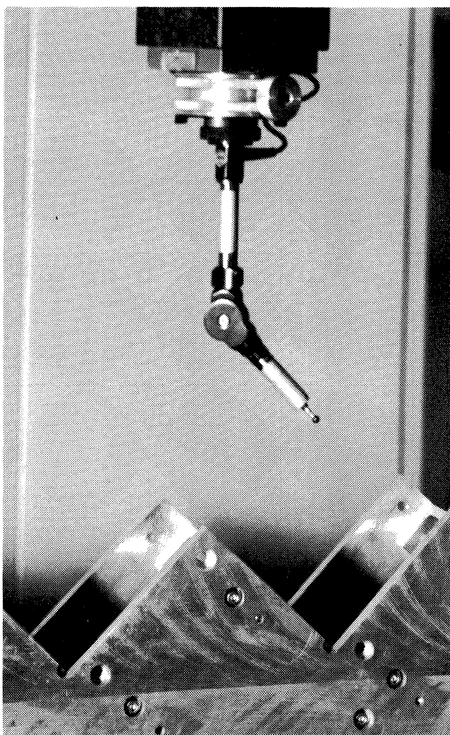
Examen sur notre nouveau dispositif de mesure d'une pièce mécanique qui n'est autre que l'une des huit cents barres de support des blocs de verre au plomb du complexe de détection d'OPAL. De gauche à droite, Christian Boudineau et René Angelloz en compagnie de Severino Rossari, chef du service de Métrologie auprès de nos Ateliers centraux. (Photo 108.11.84)
