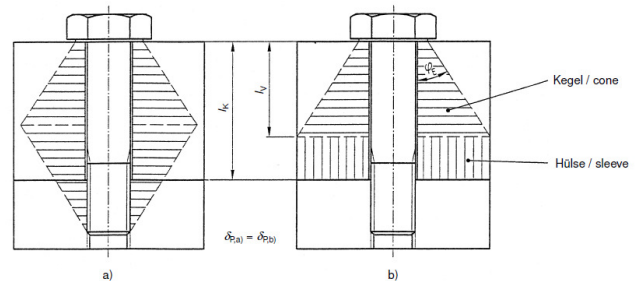
Bild 9. Zylindrische ESV a) Ersatzverformungskegel b) Berechnungsmodell
