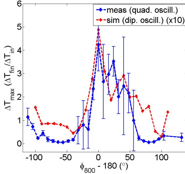
Figure 3: Λόγος τελικών προς αρχικών τετραπολικών (μετρήσεις) και διπολικών (προσομοιώσεις) Ρατίο οφ φινάλ το ινιτιαλ χυαδρουπολε (μεασυρεμεντς) ανδ πλατών ταλάντωσης, πολλαπλασιασμένοι με τη μέγιστη τιμή του ( \Delta T_{max} ) συναρτήσεως της \phi_{800} στο σύστημα 2 RF του SPS με V_r = 0.25 . Αριθμός πρωτονίων ανα πακέτο \sim 1 \times 10^{11} με \epsilon_l \simeq 0.25 eVs .
