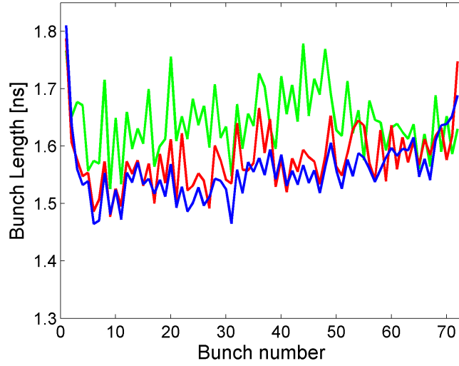
Figure 5: Μετρήσεις μήκους των πακέτων σωματιδίων πριν την ελεγχόμενη αύξηση της διαμήκους εκπεμπικότητας (πράσινο), αμέσως μετά (κόκκινο) και στο τέλος της επιτάχυνσης (μπλέ).
