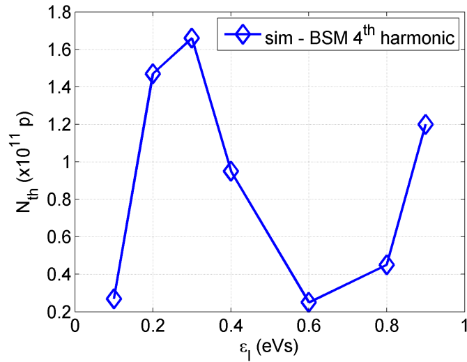
Figure 2: Κατώφλι απώλειας απόσβεσης Landau συναρτήσει της διαμήκους εκπεμπτικότητας για h_2/h_1 = 4 σε BSM τρόπο λειτουργίας, με βάση προσομοιώσεις.
