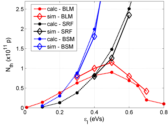
Figure 1: Κατώφλι απώλειας απόσβεσης Landau συναρτήσει της διαμήκους εκπεμπτικότητας σε σύστημα δυο RF ( BLM - κόκκινο, BSM - μπλε) και σε σύστημα μιας RF (μαύρο) με βάση αναλυτικούς υπολογισμούς (τελείες) και προσομοιώσεις (ρόμβοι).
