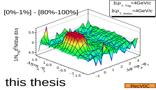
(d) Rec.MC, V0C event estimator.
