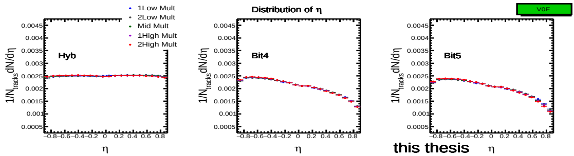
(d) ALICE experimental data, V0E event estimator.
