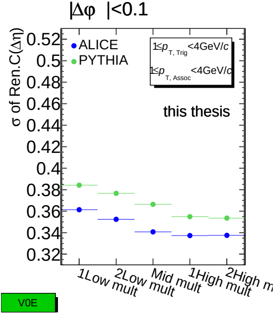
(d) ALICE experimental data, V0E event estimator.
