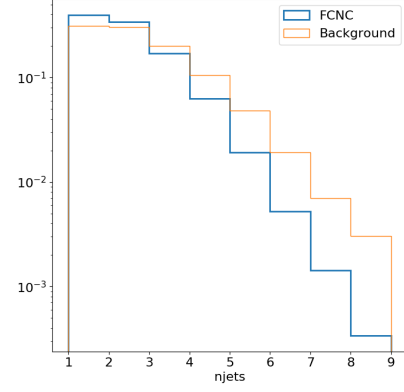
(d) n_{lets}
