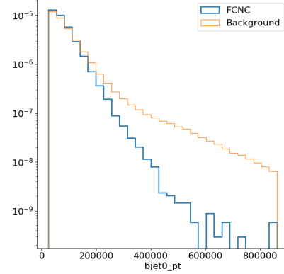
(d) p_T(b)
