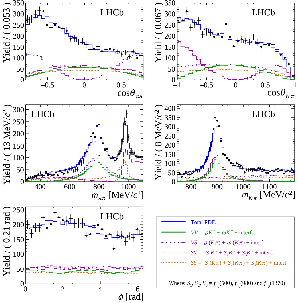
Figure A.7: Proxeccións do axuste multidimensional na mostra de datos do \bar{B}^0 .
