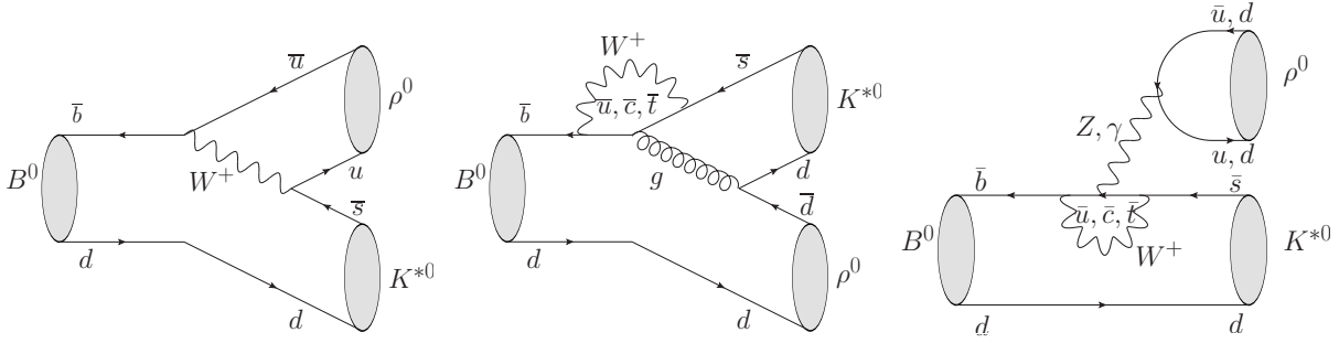
Figure A.1: Esquemas dos diagramas de Feynman que dominan o decaemento B^0 \rightarrow \rho^0 K^{*0} . De esquerda a dereita: diagrama “tree” dobreemente suprimido por Cabibbo, diagrama “penguin” gluónico e diagrama “penguin” electrofeble.
