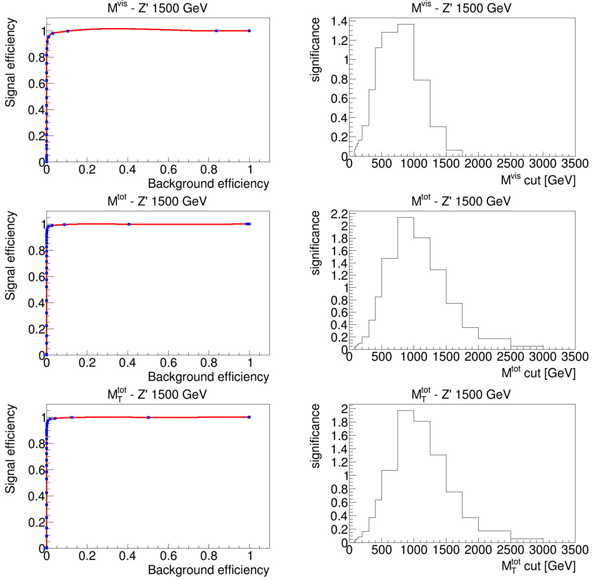
FIGURE 3.5 – Du côté gauche, les courbes ROC, représentant l'efficacité du signal (Z' de 1500 GeV du MSS) en fonction de l'efficacité du bruit de fond, pour différentes coupures sur la masse reconstruite. Les coupures sont de la forme M_{\text{reco}} > x . x commence à 0 au coin supérieur droit et augmente de 50 en 50 GeV jusqu'à atteindre 1000 GeV. À partir de là les augmentations se font de 100 en 100 GeV. Du côté droit, les distributions de la signification du signal en fonction de la coupure utilisée sur la masse reconstruite. La coupure correspond à la valeur inférieure de chaque bin. De haut en bas, les graphiques concernent la masse visible, la masse totale et la masse transverse totale.
