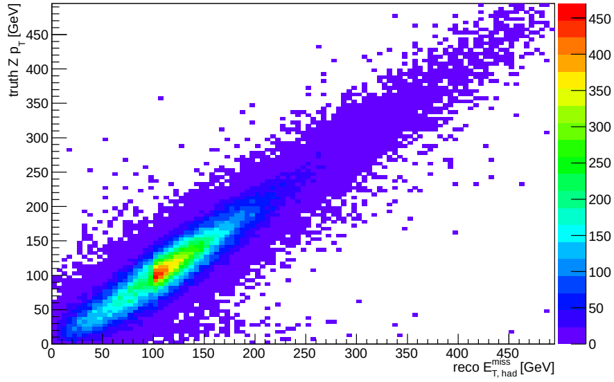
(b) E_{T,\text{had}}^{\text{miss}}
